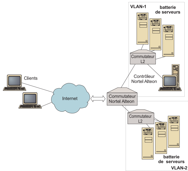
Figure 29. Exemple de consultant connecté derrière le commutateur
