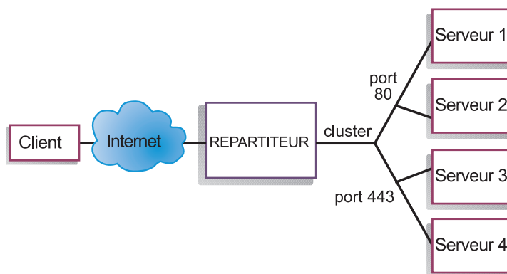
Figure 9. Exemple de composant Dispatcher configuré avec un cluster et 2 ports
