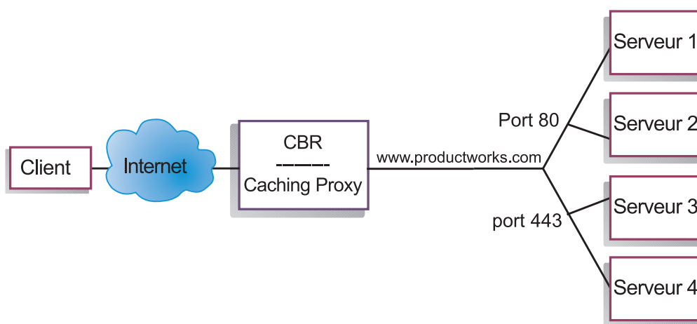
Figure 17. Exemple de composant CBR configuré avec un cluster et 2 ports
