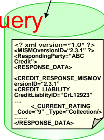
BLOB (Oracle)
