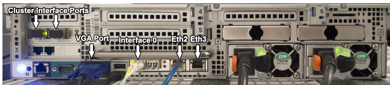
図 3. クラスター・マスターまたはスタンドアロン・システム
