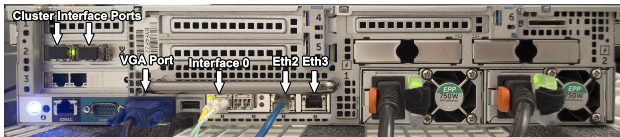
図 1. クラスター・マスターまたはスタンドアロン・システム
