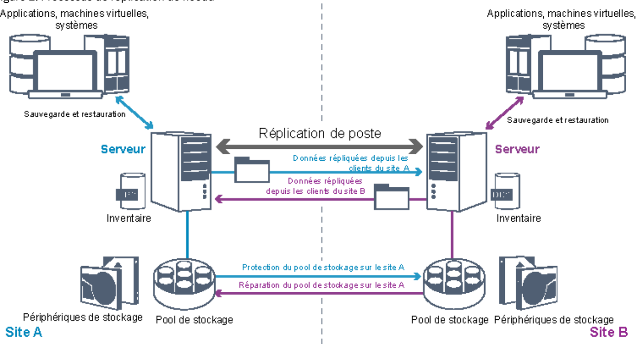
Figure 1. Processus de réplication de noeud
