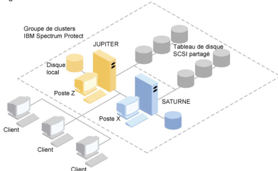
Figure 1. Mise en cluster avec JUPITER comme noeud Z et SATURNE comme noeud X
