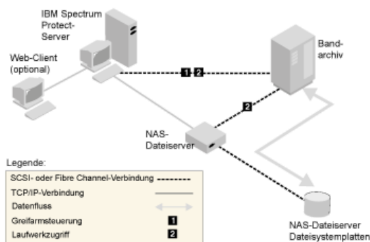
Abbildung 1. Konfiguration 1: An den IBM Spectrum Protect-Server angeschlossenes SCSI-Speicherarchiv
