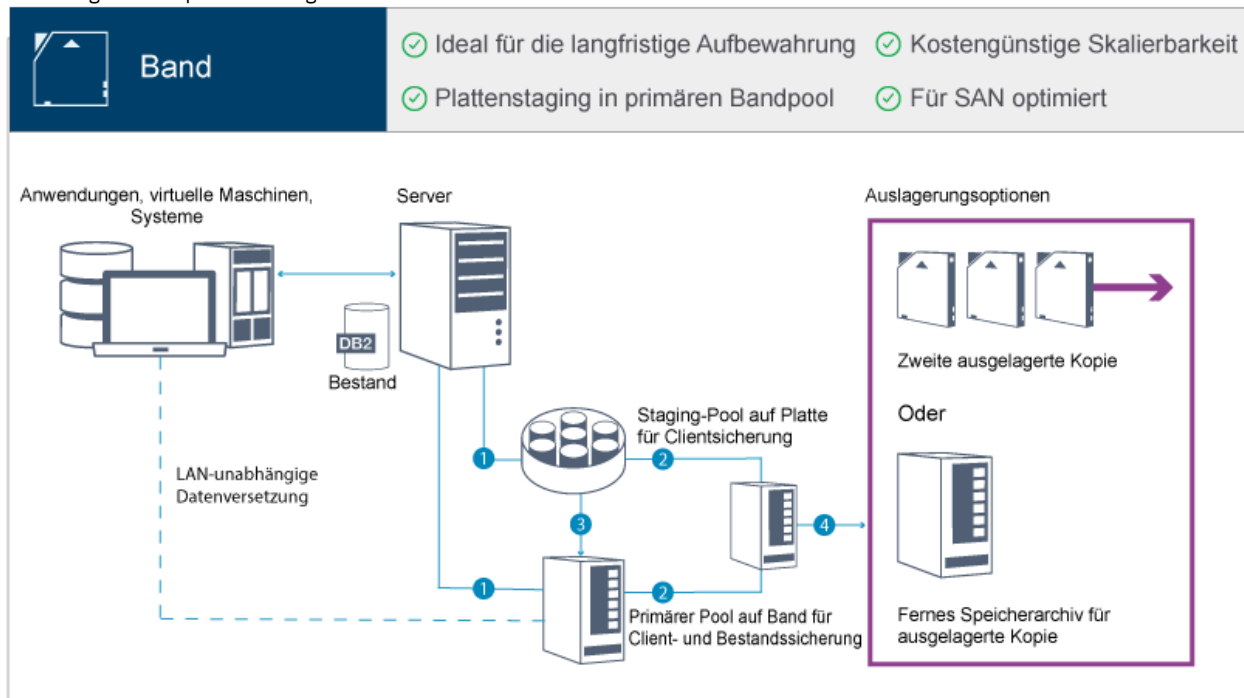
Abbildung 1. Bandspeicherlösung
