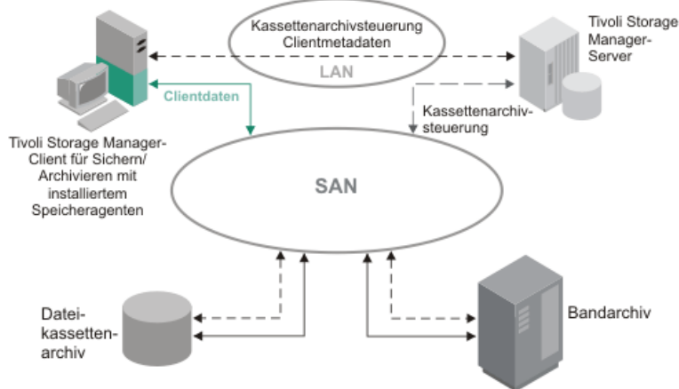
Abbildung 1. LAN-unabhängige Datenversetzung
