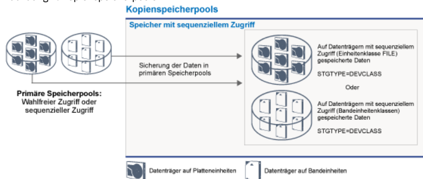
Abbildung 2. Kopierspeicherpools
