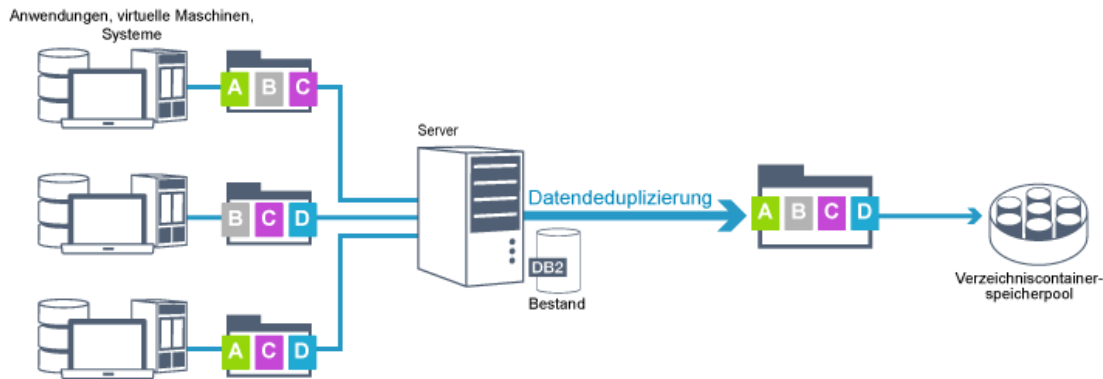
Abbildung 1. Dateneduplizierungsprozess
