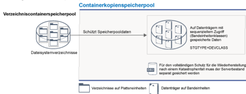
Abbildung 3. Containerkopierspeicherpools
