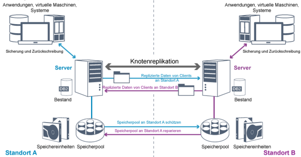
Abbildung 1. Knotenreplikationsprozess
