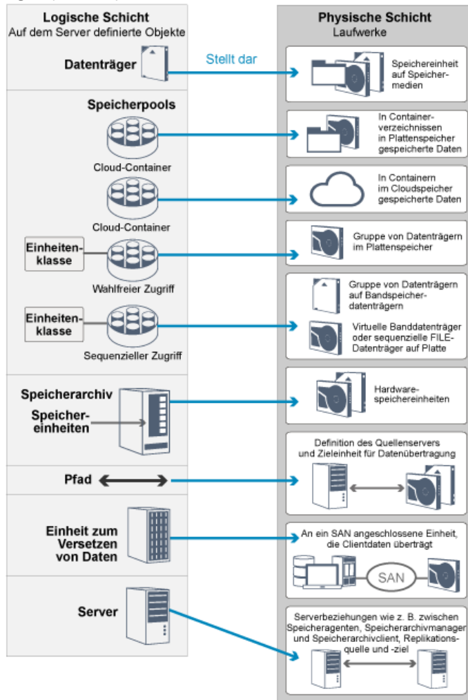
Abbildung 1. Speicherobjekte
