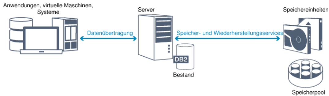
Abbildung 1. Datenschutzservices
