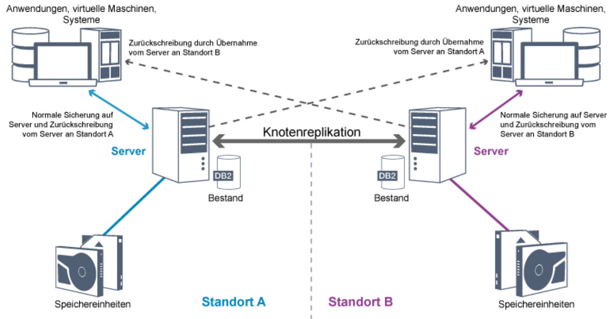
Abbildung 1. Automatischer Übernahmeprozess
