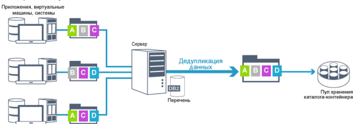
Рис. 1. Процесс дедубликации данных
