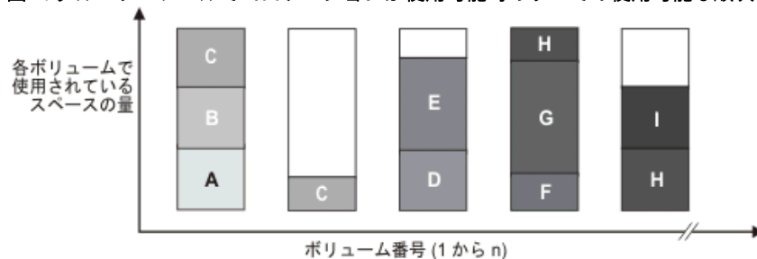
図 2. グループ・レベルでコロケーションが使用可能時のすべての使用可能な順次アクセス・ストレージ・ボリュームの使用
