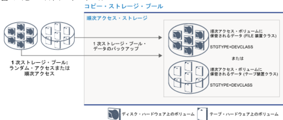
図2. コピー・ストレージ・プール
