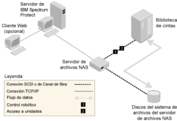
Figura 1. Configuración 2: biblioteca SCSI conectada al servidor de archivos NAS
