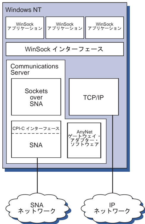
図 14. Sockets over SNA が実行される Windows NT ノードの構造
