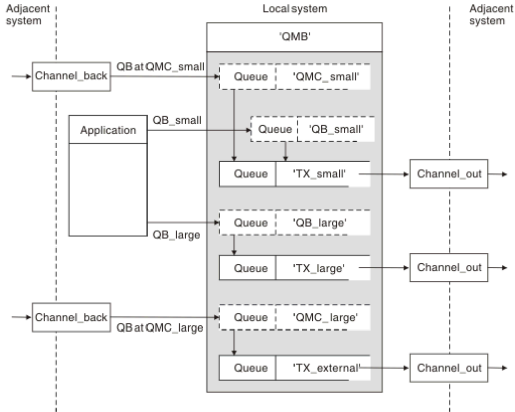
图 10: 分隔消息流
