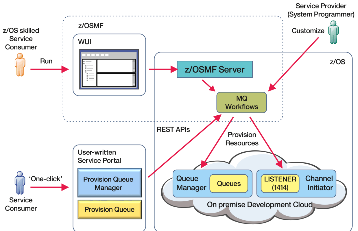
图 125: "一键式" 供应 IBM MQ for z/OS 资源
