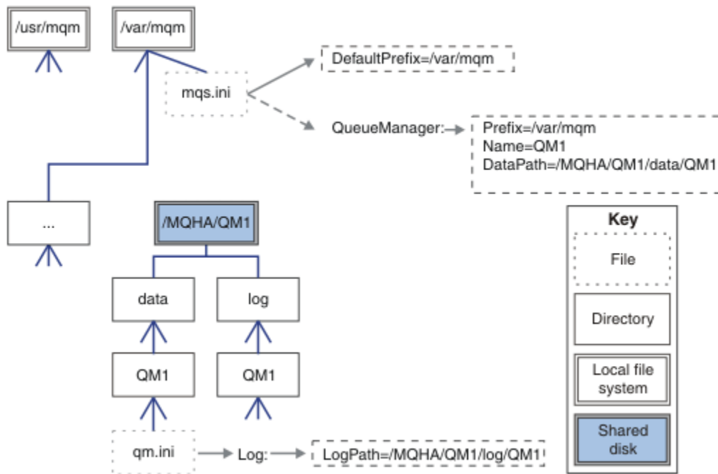
图 70: 共享名为 data 和 log 的目录
