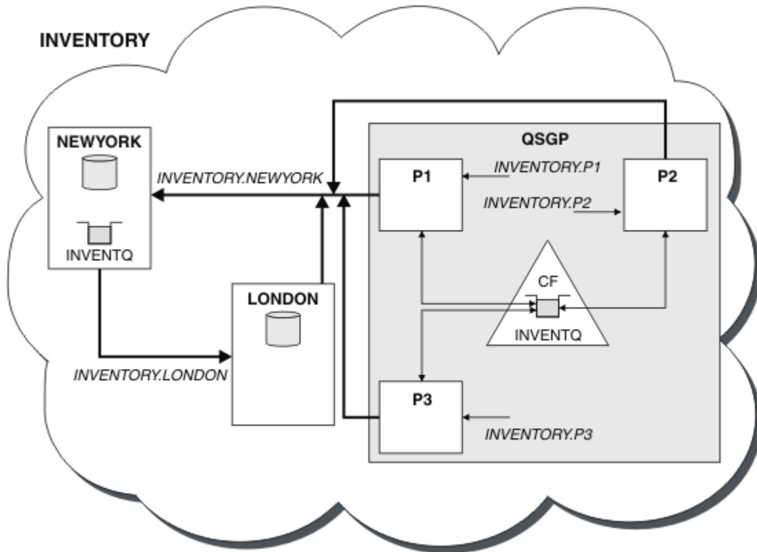
图 43: 集群和队列共享组
