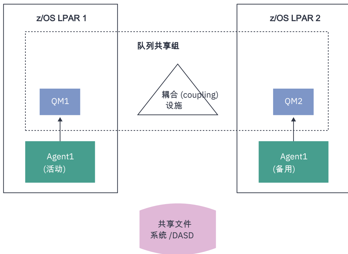
图 95: 使用队列共享组的高可用性 MFT 代理
