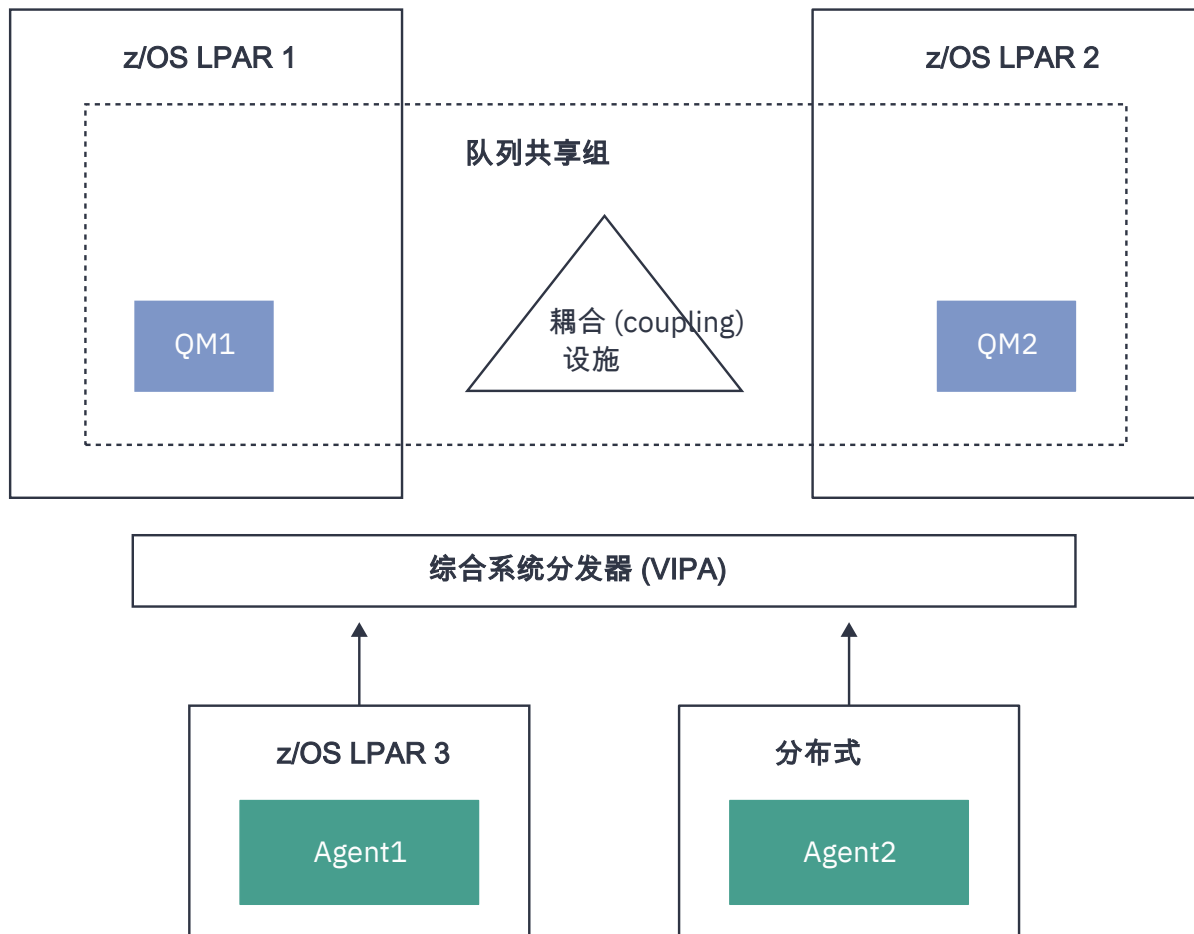
图 96: 作为客户机连接到队列共享组的 MFT 代理程序
