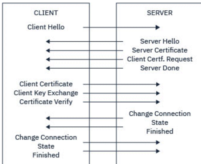
Figura 5. Visão geral do handshake do TLS
