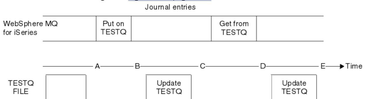
Figura 22. Sequência de eventos ao atualizar objetos MQM
