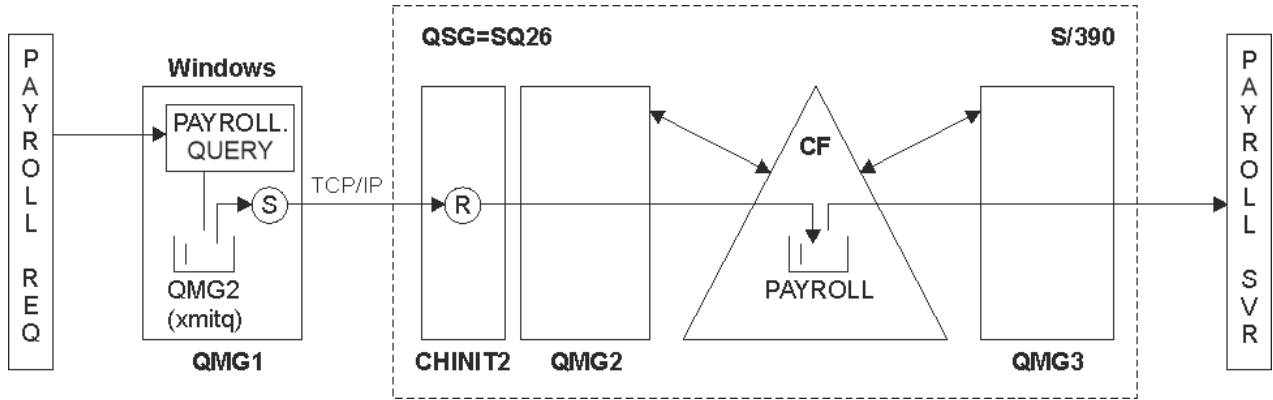
그림 4. 구성 3
