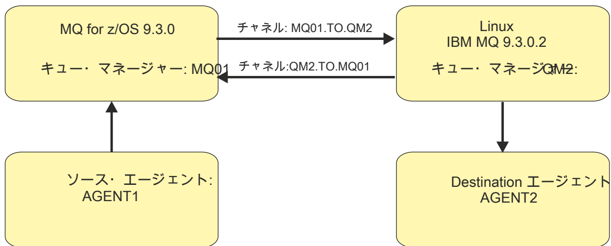
図 54. ソース・エージェント AGENT1 と宛先エージェント AGENT2、およびそれらのエージェント・キュー・マネージャー MQ01 と QM2 が接続される方法を示す単純な図。
