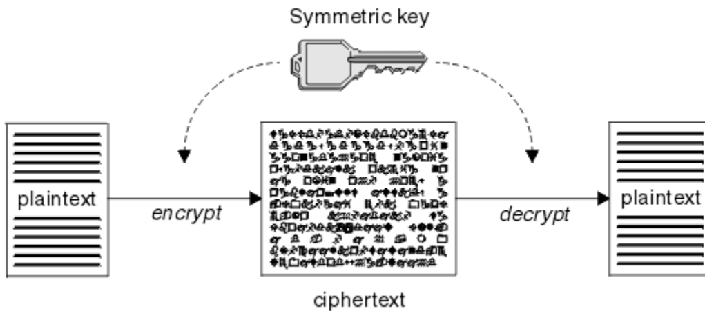
図 1. 対称鍵暗号化方式
