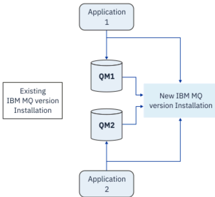
図 6. 横並びマイグレーション: マイグレーションされたキュー・マネージャーが新しいバージョンに接続され、アプリケーションが新しいバージョンに関連付けられている
