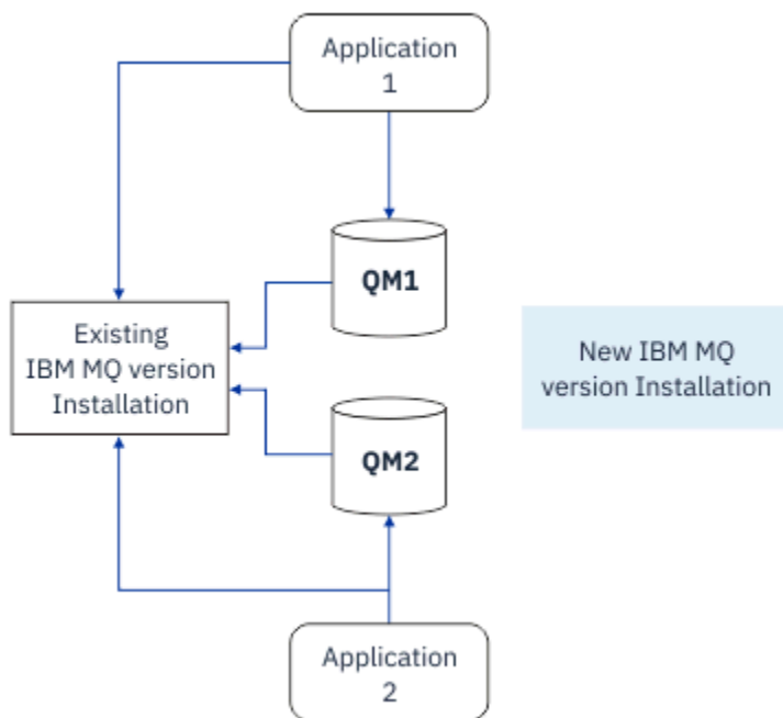
図 5. 横並びマイグレーション: 新しいバージョンがインストールされているが、キュー・マネージャーはまだ前のバージョンに接続され、アプリケーションはまだ前のバージョンに関連付けられている
