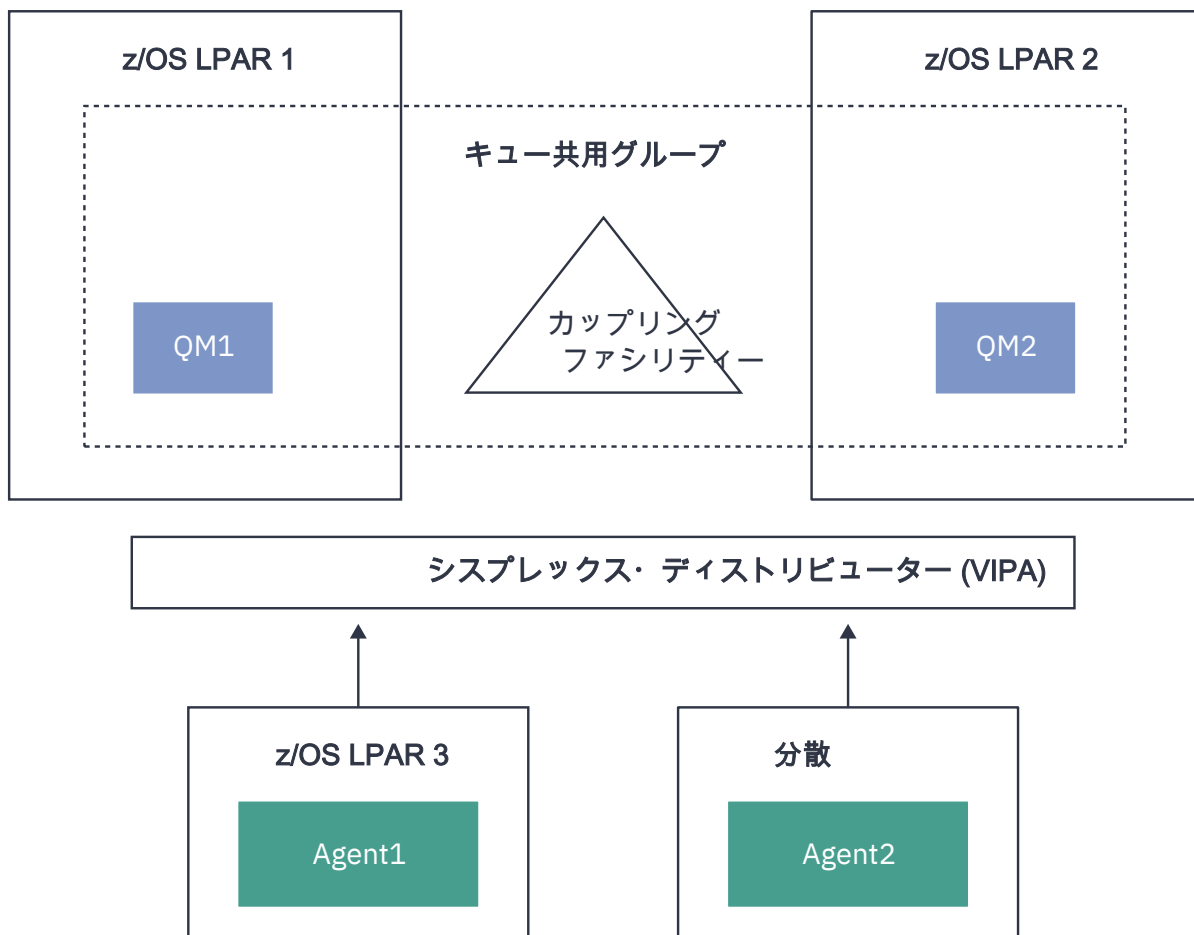
図 96. クライアントとしてキュー共有グループに接続する MFT エージェント
