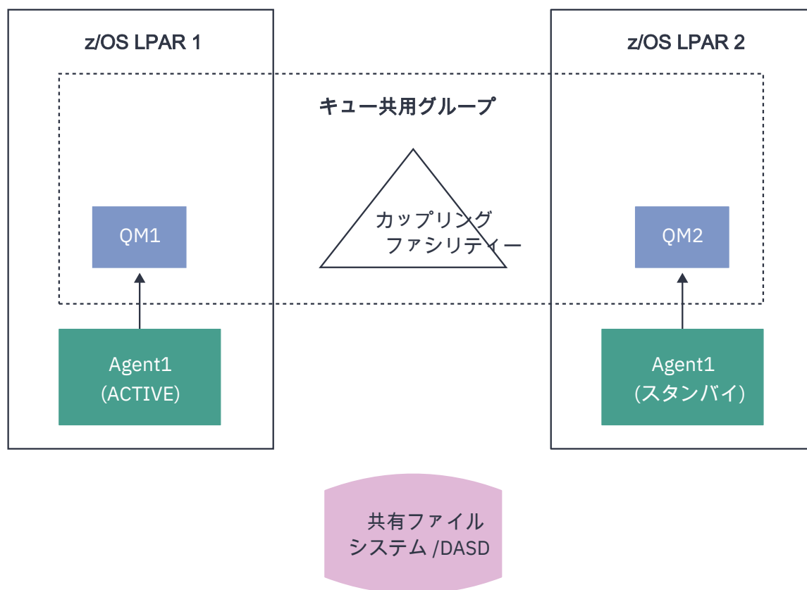
図 95. キュー共有グループを使用した高可用性 MFT エージェント
