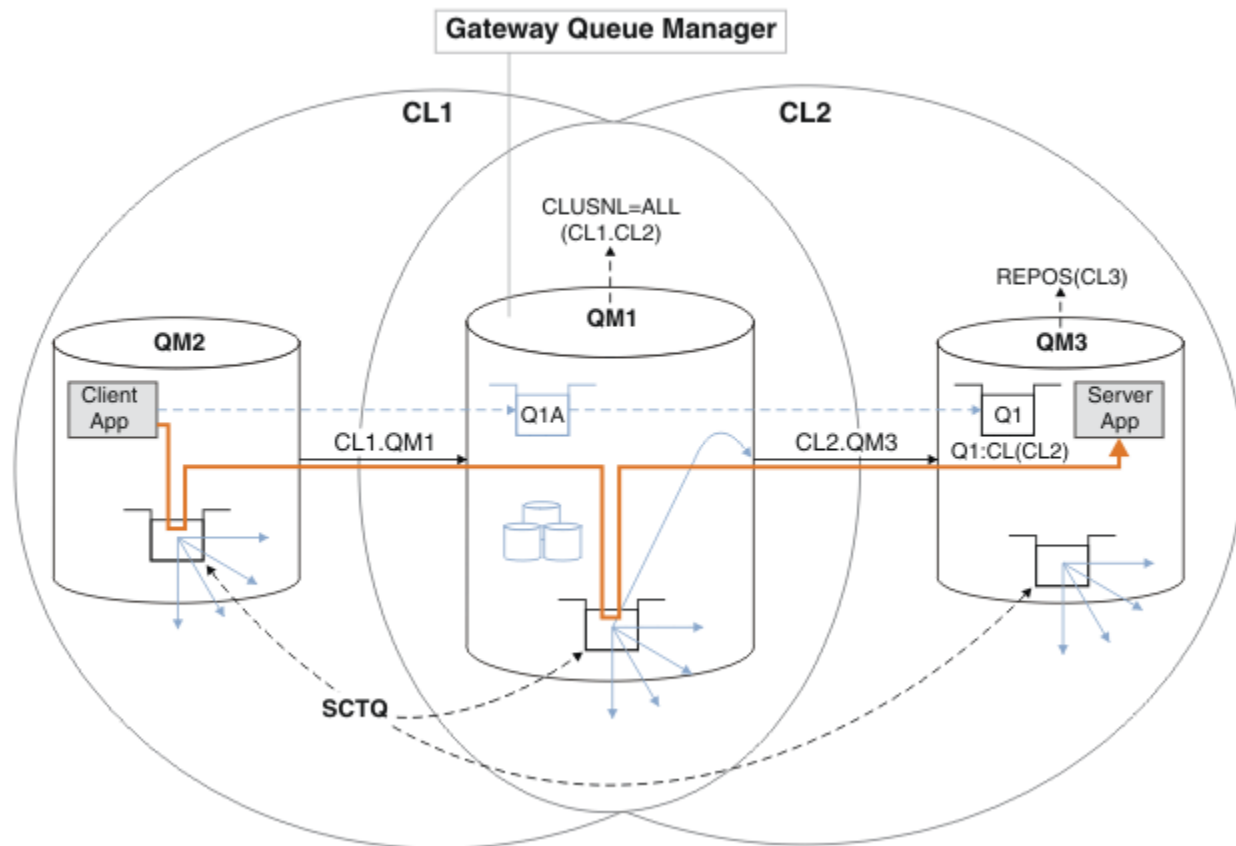
図 47. ハブ・スポーク・アーキテクチャにデプロイされた、IBM MQ クラスタを使用するクライアント/サーバー・アプリケーション
