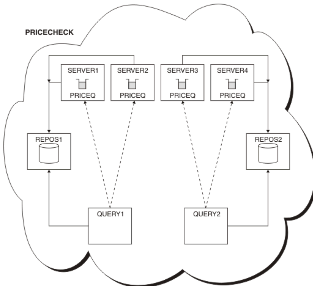
図 63. 4つのサーバー・キュー・マネージャー、2つのリポジトリ、および2つの照会キュー・マネージャーを持つ PRICESCHECK クラスター
