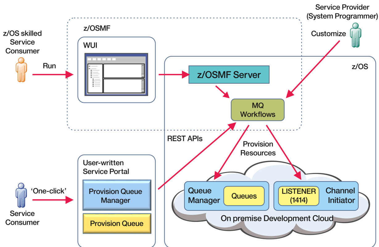
図 125. IBM MQ for z/OS リソースの「ワンクリック」プロビジョニング
