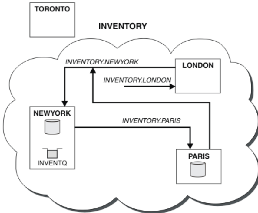
図 44. 完全リポジトリが PARIS に移動した INVENTORY クラスタ
