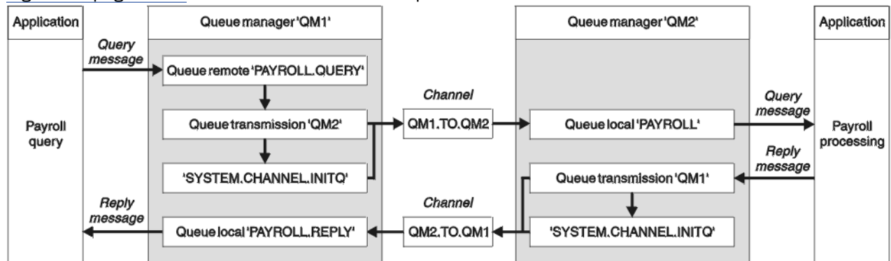
Figura 7. Esempio di canale dei messaggi per sistemi AIX, Linux, and Windows
