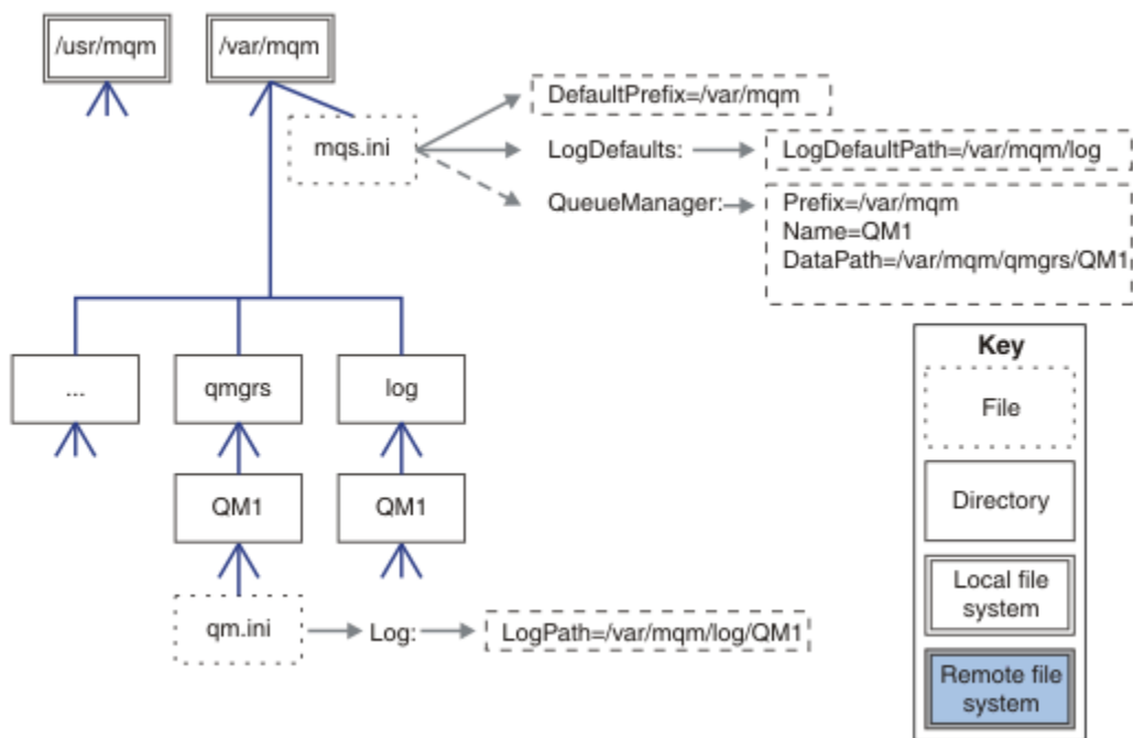
Figura 35. Struttura di directory IBM MQ predefinita di esempio per sistemi AIX and Linux
