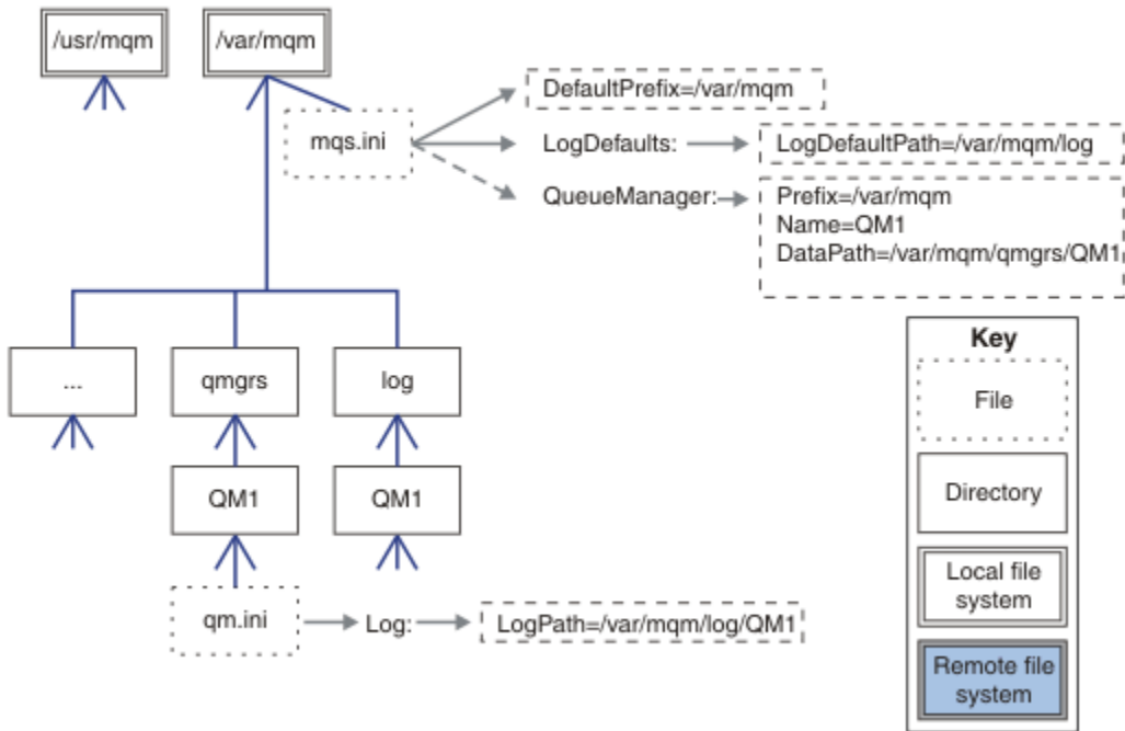
Figura 37. Struttura di directory IBM MQ predefinita di esempio per sistemi AIX and Linux
