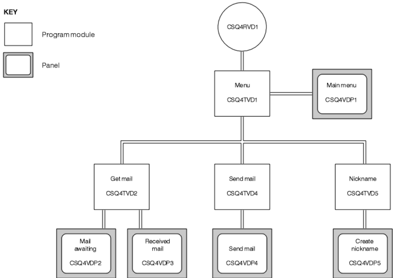
Figure 140. Programmes et panneaux pour les versions TSO du gestionnaire de messagerie
