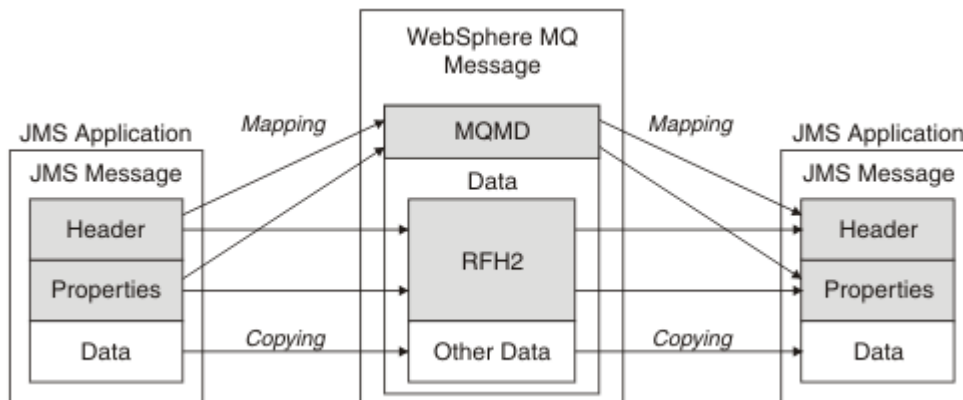
Figure 10. Comment les messages sont transformés entre JMS et IBM MQ à l'aide de l'en-tête MQRFH2
