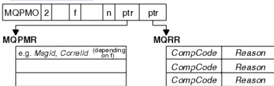
Figure 59. Insertion d'un message dans une liste de distribution en C
