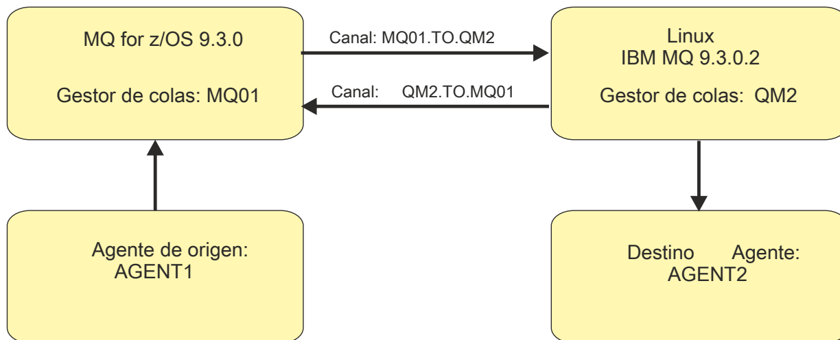
Figura 55. Ejemplo de un diagrama simple que muestra cómo se conectan un agente de origen, AGENT1, y un agente de destino, AGENT2, y sus gestores de colas de agente, MQ01 y QM2 .
