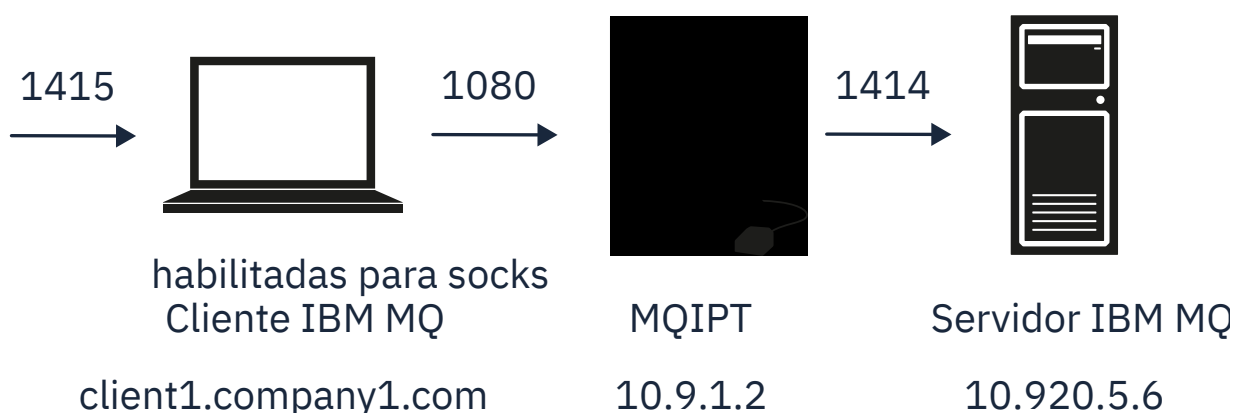
Figura 36. Diagrama de red de proxy SOCKS
