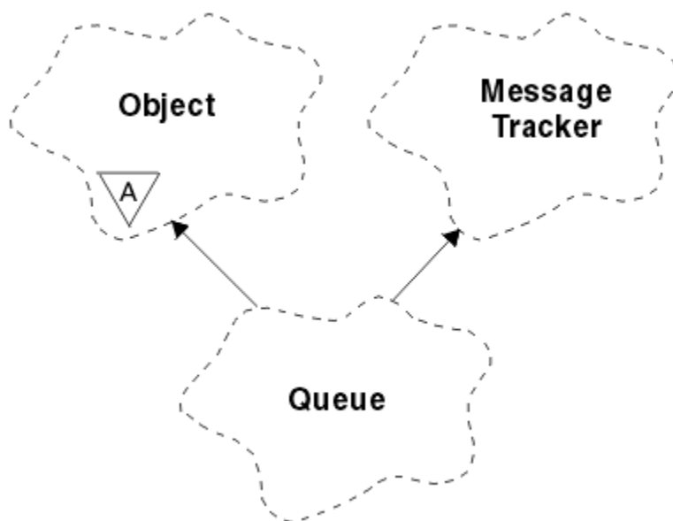
Figura 32. Clase ImqQueue
