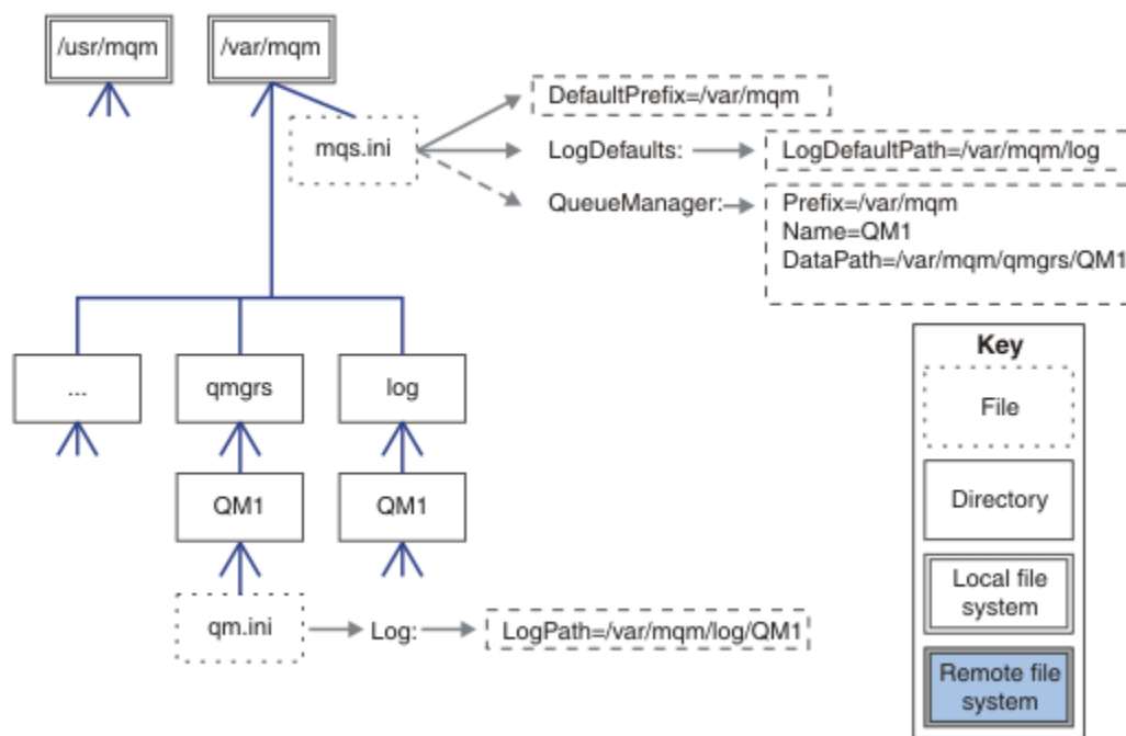
Figura 35. Ejemplo de estructura de directorios predeterminada de IBM MQ para los sistemas AIX and Linux
