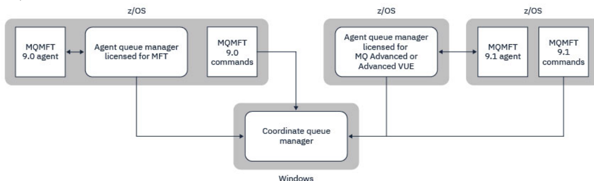
Figura 48. Determinados mandatos, como por ejemplo ftelistagents , se conectan directamente al gestor de colas de coordinación para una topología de MFT.
