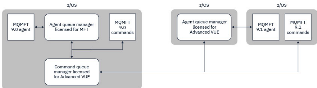
Figura 46. Los mandatos se conectan al gestor de colas de mandatos para una topología MFT. Al ejecutar estos mandatos en z/OS, el gestor de colas de mandatos también debe estar en z/OS
