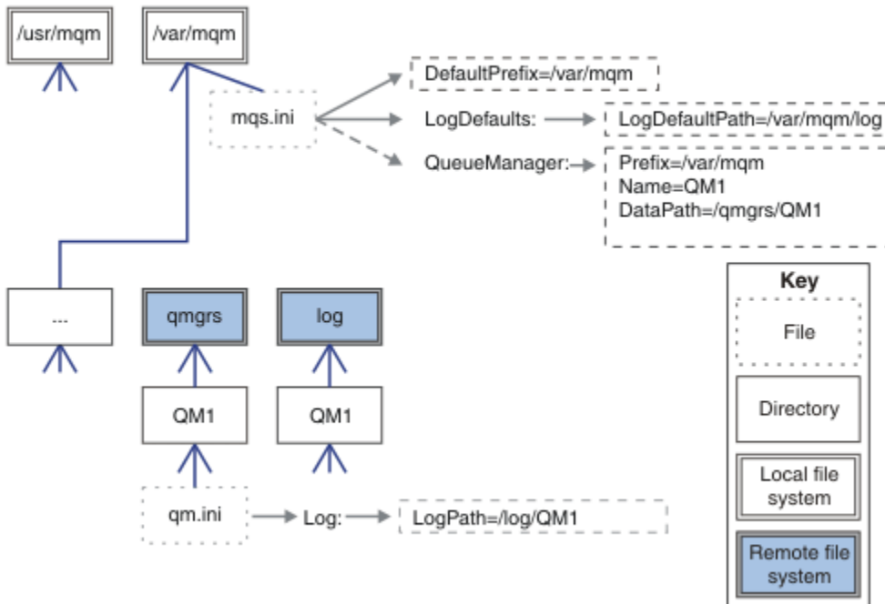
Abbildung 38. qmgrs- und log-Verzeichnisse gemeinsam nutzen
