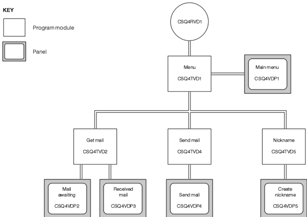
Abbildung 140. Programme und Anzeigen für die TSO-Versionen des Mail-Manager-Beispielprogramms
