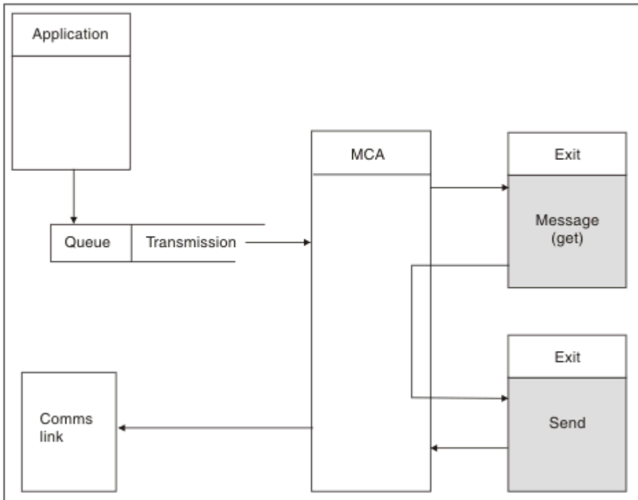
Abbildung 104. Beispiel eines Sendeexits auf der Sendeseite des Nachrichtenkanals
