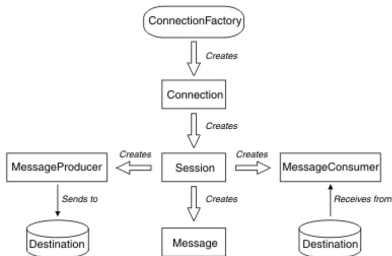
Abbildung 52. XMS-Objekte und ihre Beziehungen
