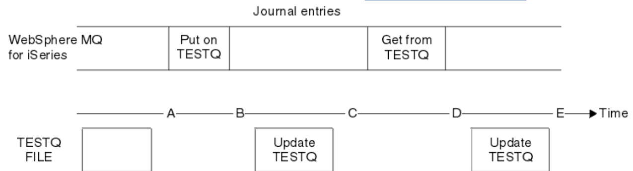
Abbildung 22. Reihenfolge von Ereignissen beim Aktualisieren von MQM-Objekten
