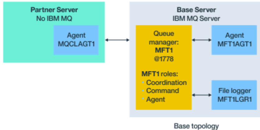
圖 28: 含有 Managed File Transfer Agent 友機的基本拓撲
