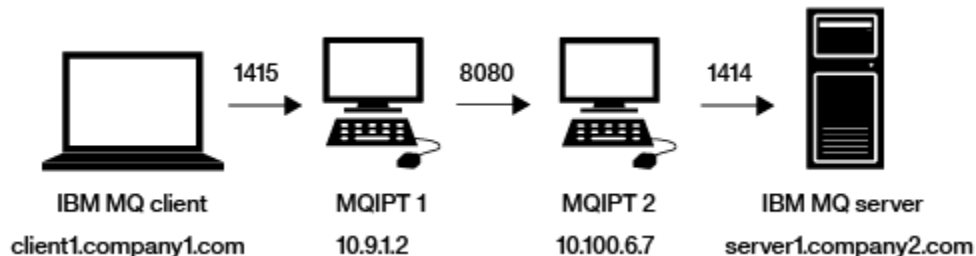
圖 33: HTTP 通道作業網路圖
