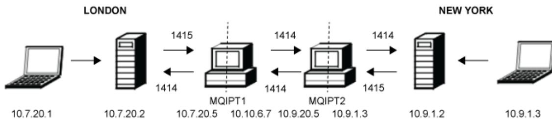
圖 37: 叢集作業網路圖
