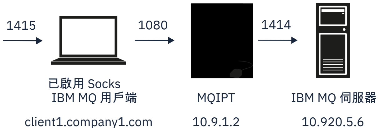
圖 35: SOCKS Proxy 網路圖
