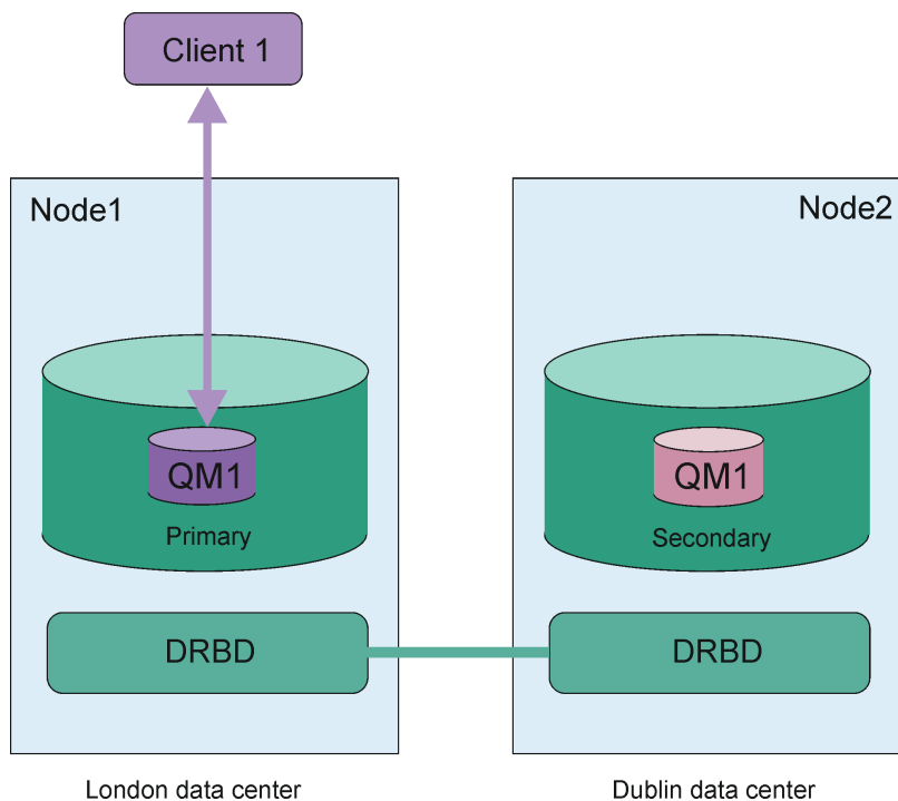
圖 84: 單一 RDQM 配對
