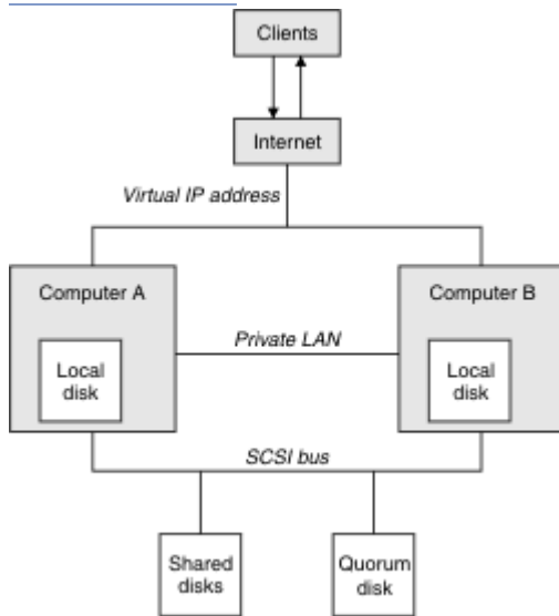
圖 74: 雙電腦 MSCS 叢集
