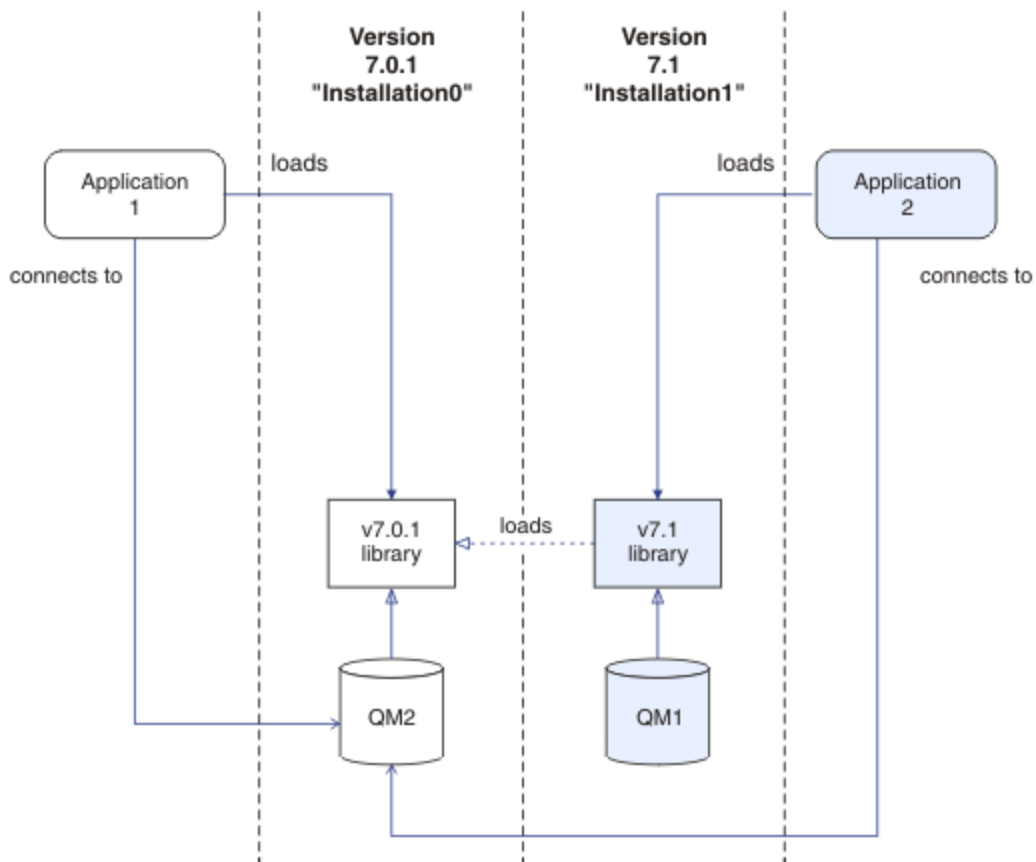
圖 70: 在多重安裝環境中連接應用程式
