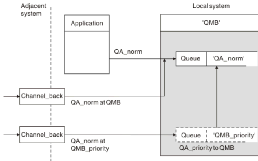
圖 10: 直接接收訊息，並解析別名佇列管理程式名稱
