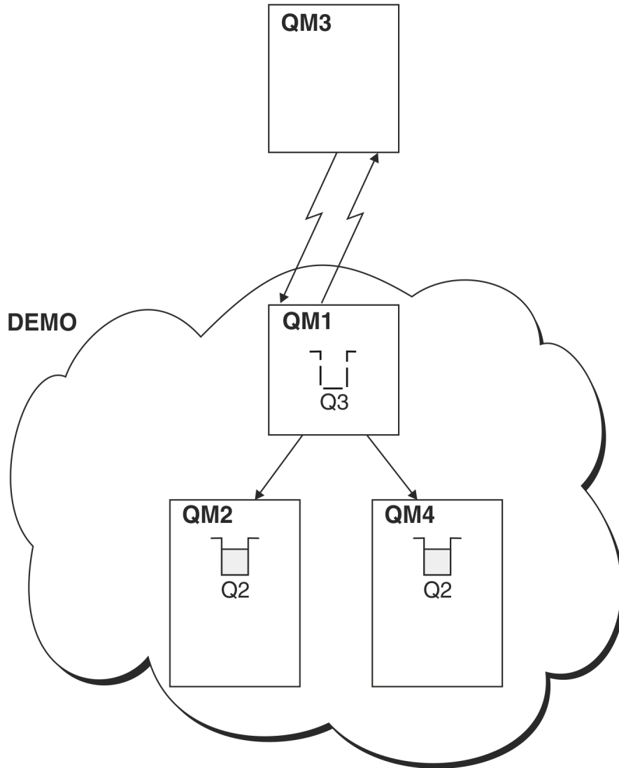
圖 58: 從叢集外部的佇列管理程式放置
