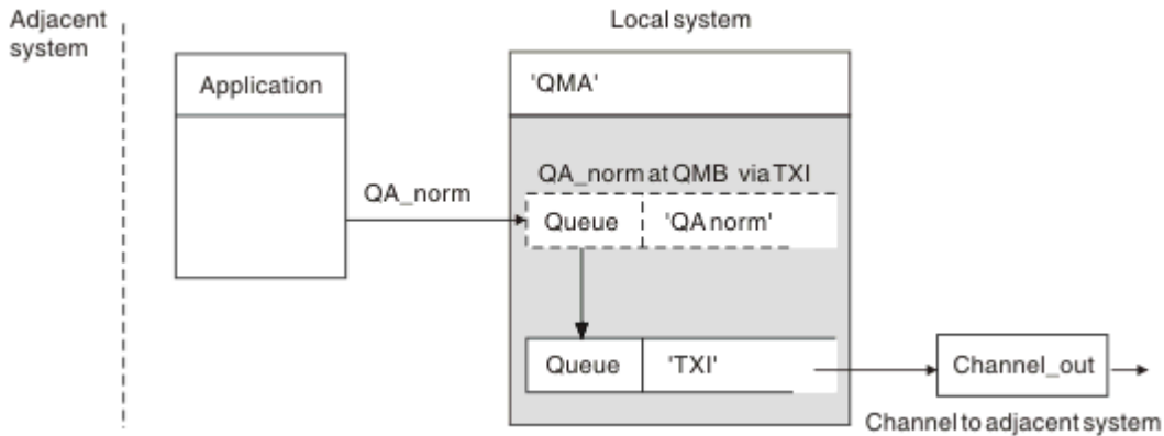
圖 9: 遠端佇列定義容許使用不同的傳輸佇列
