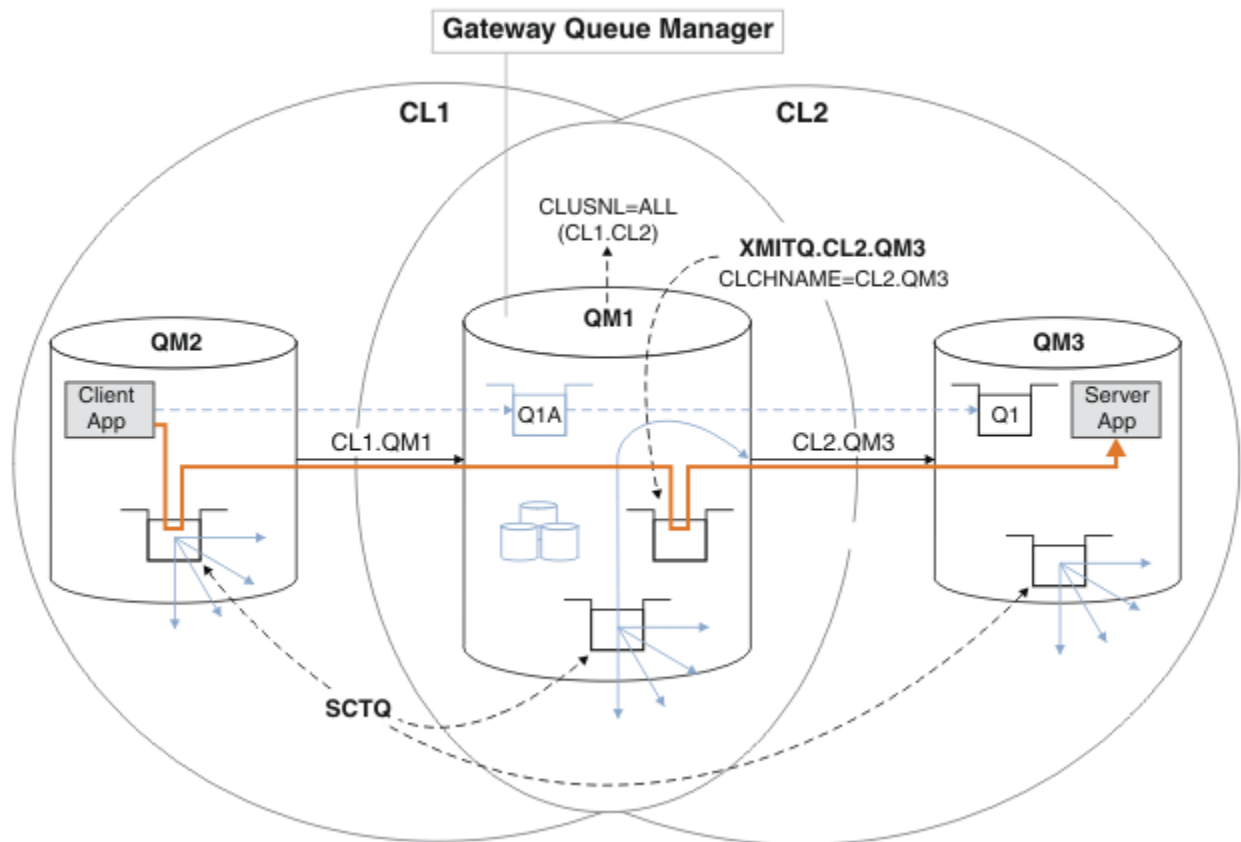
圖 52: 使用其他叢集傳輸佇列部署至中心及分支架構的主從架構應用程式。
