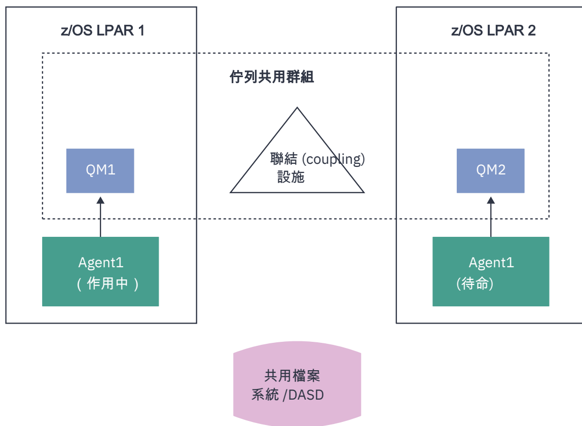
圖 98: 使用佇列共用群組的高可用性 MFT 代理程式
