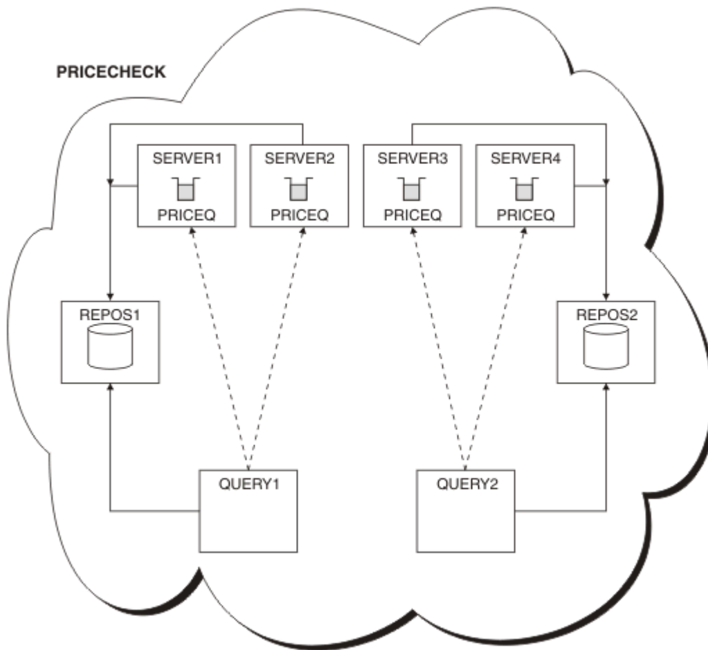
圖 65: PRICECHECK 叢集，具有四個伺服器佇列管理程式、兩個儲存庫及兩個查詢佇列管理程式
