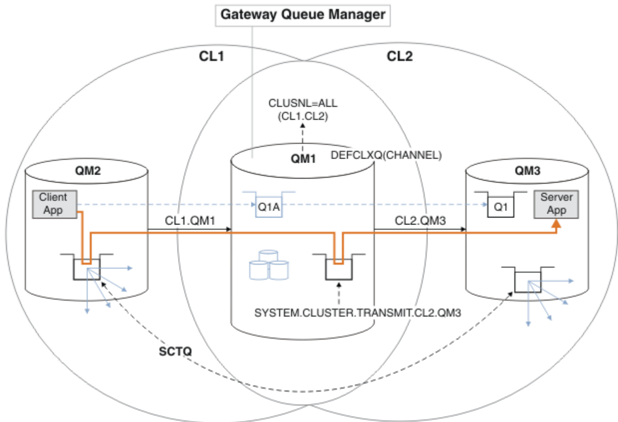
圖 54: 將主從架構應用程式部署至閘道佇列管理程式上具有個別叢集傳輸佇列的 hub 及輪輻架構。
