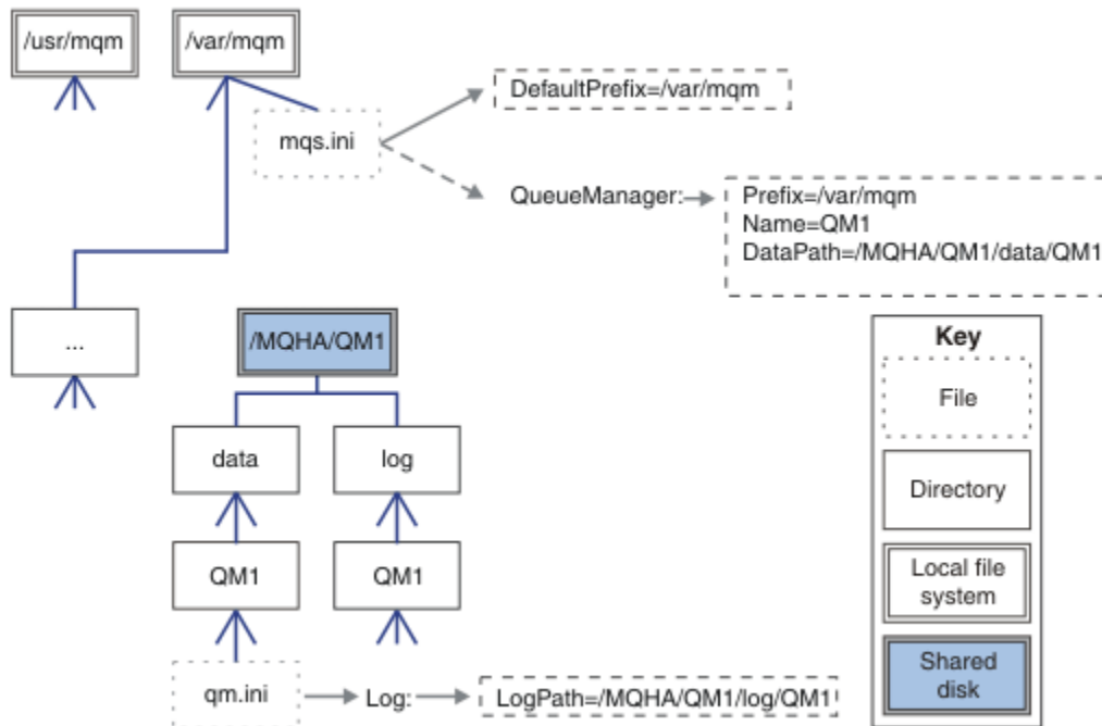
圖 73: 共用具名 data 及 log 目錄
