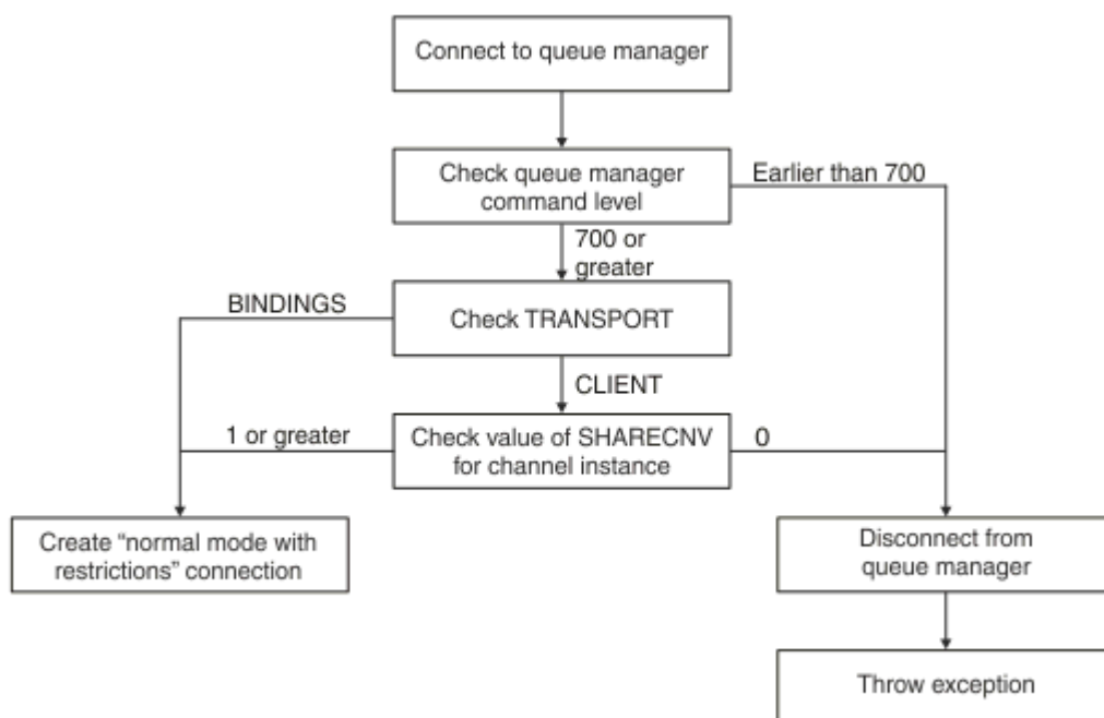
圖 94: PROVIDERVERSION 標準模式有限制
