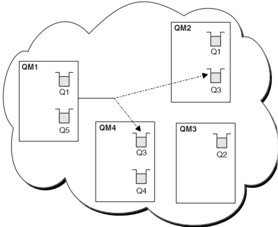
圖 61: 具有相同佇列的多個實例的叢集
