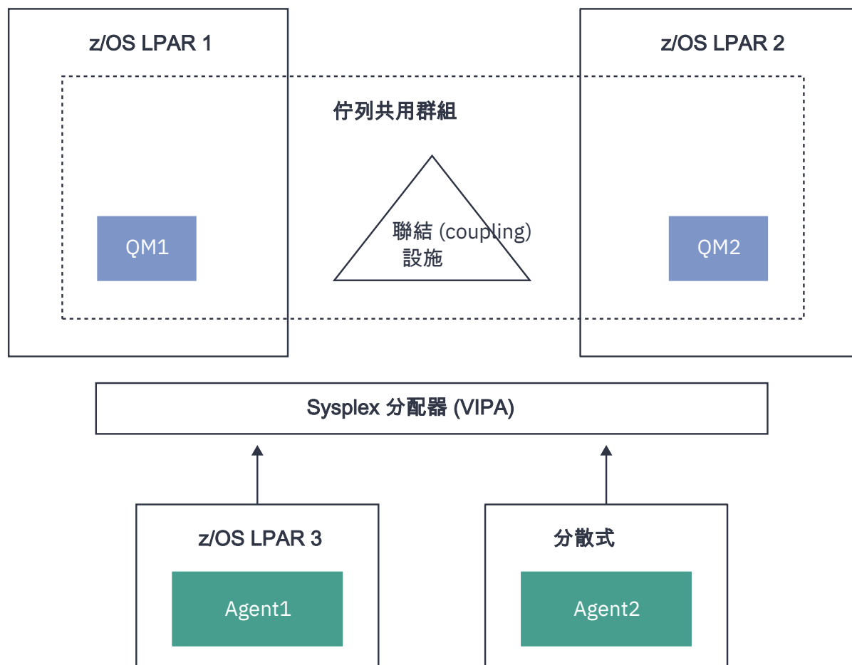
圖 99: 作為用戶端連接至佇列共用群組的 MFT 代理程式
