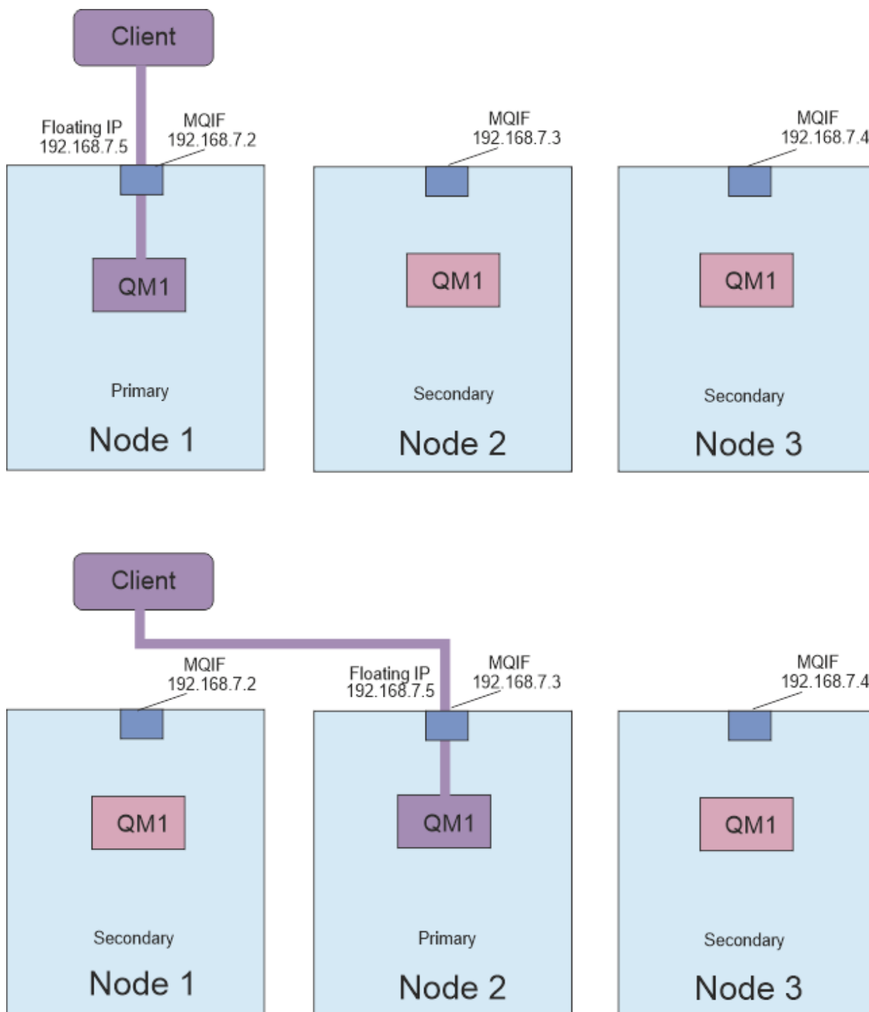
圖 83: 浮動 IP 位址
