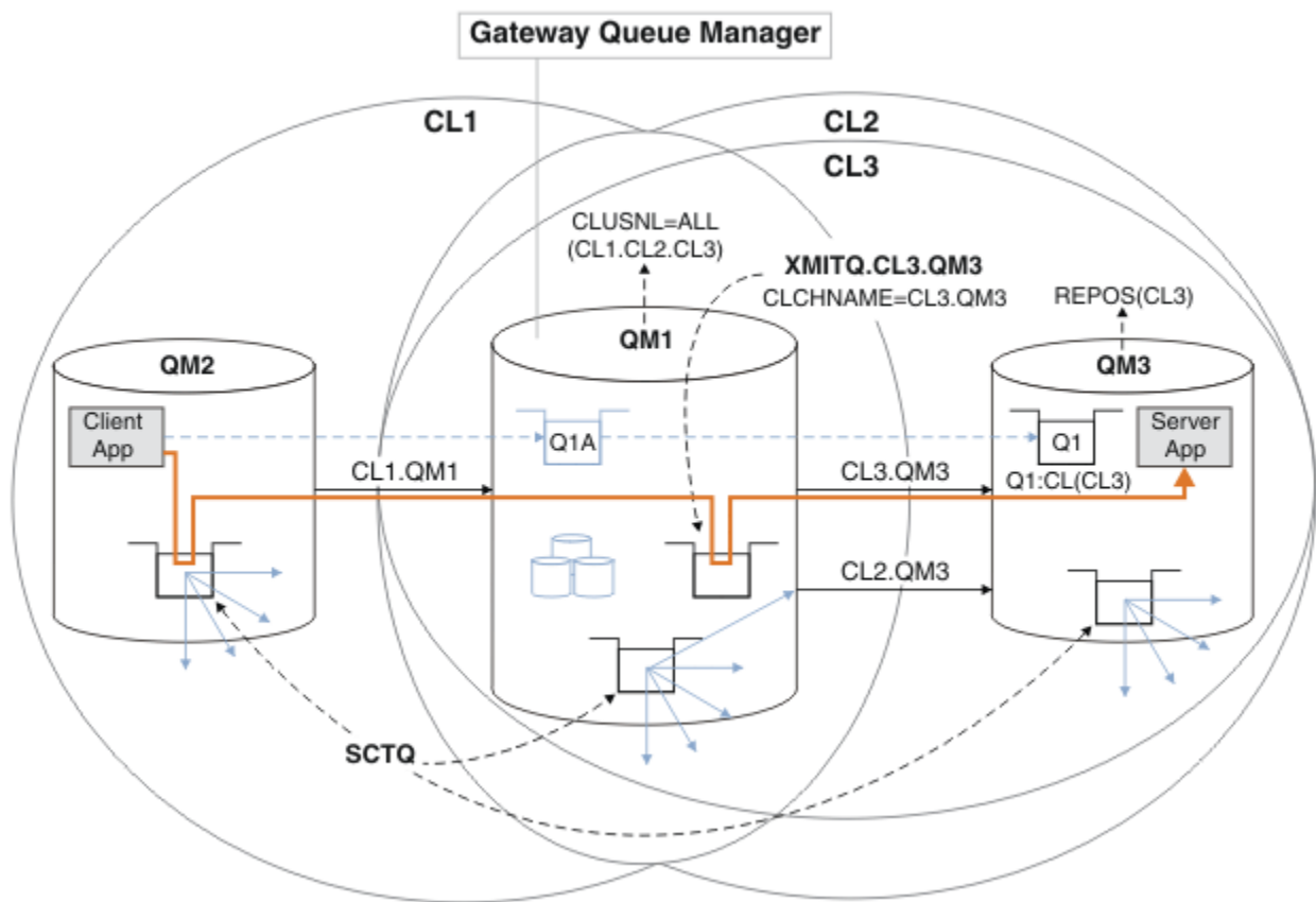
圖 53: 使用額外叢集來區隔閘道佇列管理程式中的訊息資料流量，該閘道佇列管理程式會進入相同佇列管理程式上的許多叢集佇列之一
