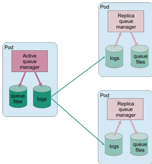
圖 86: 原生 HA 配置範例
