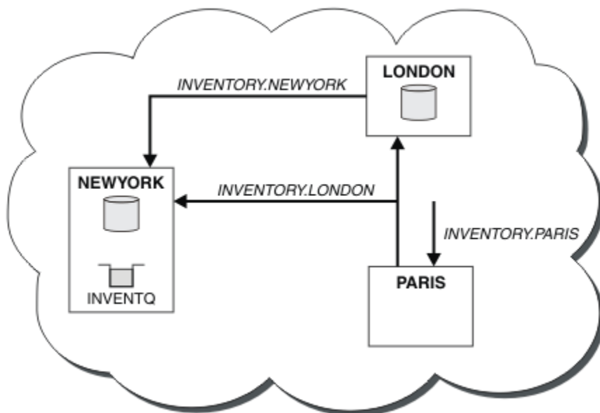
圖 43: 具有三個佇列管理程式的 INVENTORY 叢集
