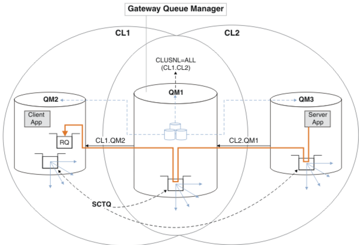
圖 50: 使用佇列管理程式別名將回覆訊息傳回至不同的叢集
