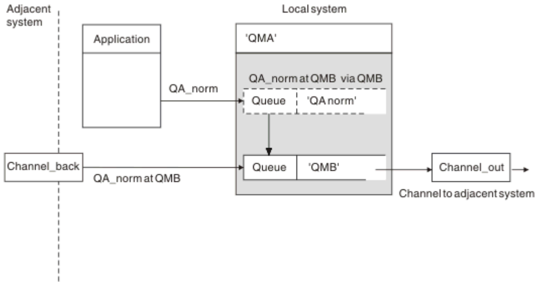
圖 8: 遠端佇列定義用來將佇列名稱解析成相鄰佇列管理程式的傳輸佇列
