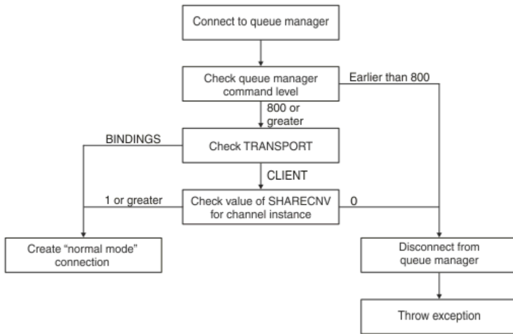
圖 93: PROVIDERVERSION 標準模式
