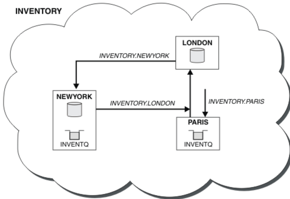
圖 62: INVENTORY 叢集，具有三個佇列管理程式
