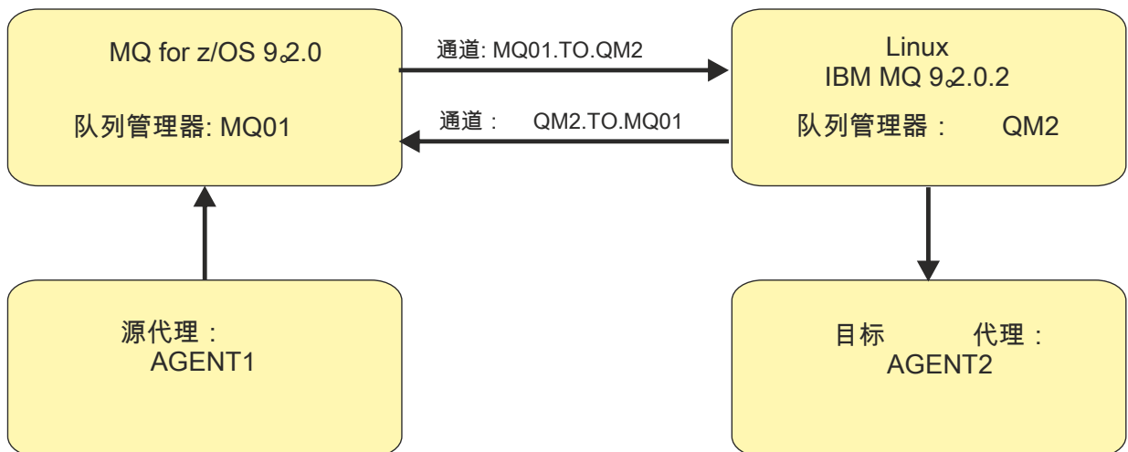
图 56: 显示如何连接源代理 AGENT1 和目标代理 AGENT2 及其代理队列管理器 MQ01 和 QM2 的简单图示例。
