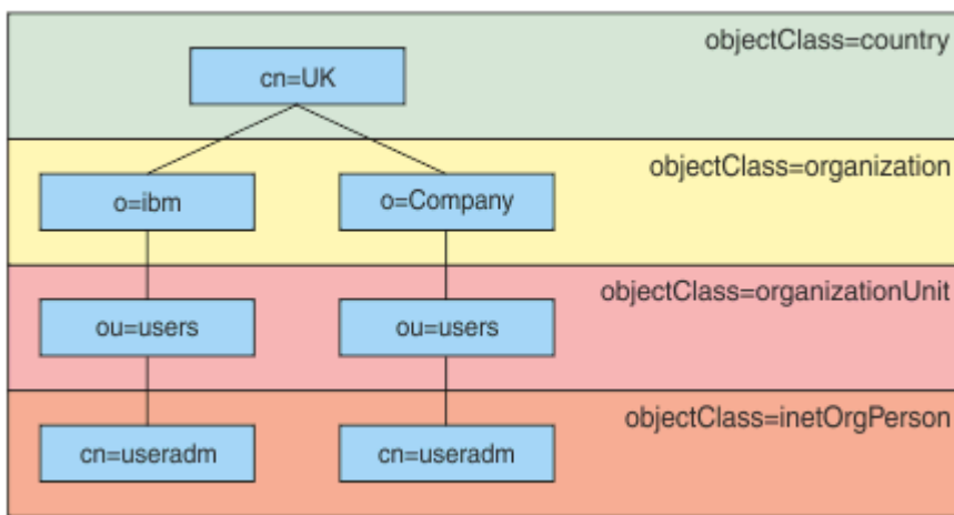
图 8: 示例 LDAP 层次结构
