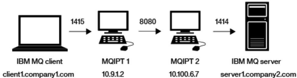
图 33: HTTP 隧道网络图
