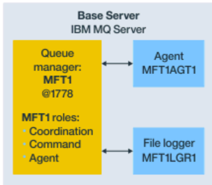
图 25: 包含一个队列管理器的基本拓扑
