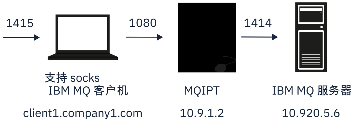
图 35: SOCKS 代理网络图
