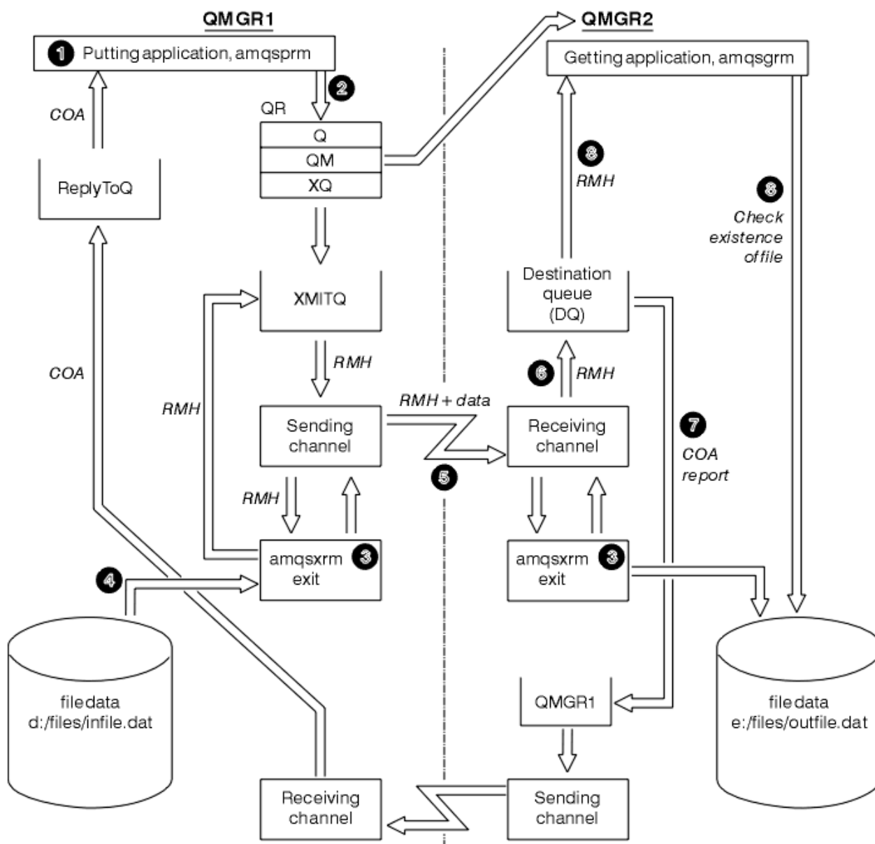
图 135: 运行“参考消息”样本
