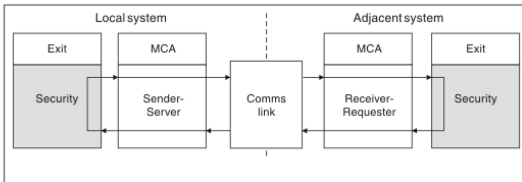
图 107: 安全出口循环
