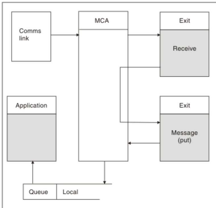
图 109: 消息通道的接收方端的接收出口示例
