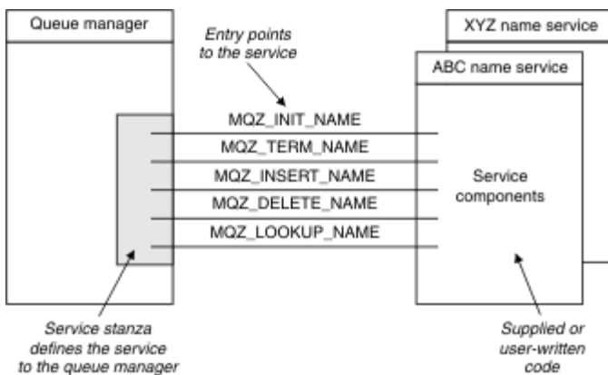
图 103: 理解服务、组件和入口点
