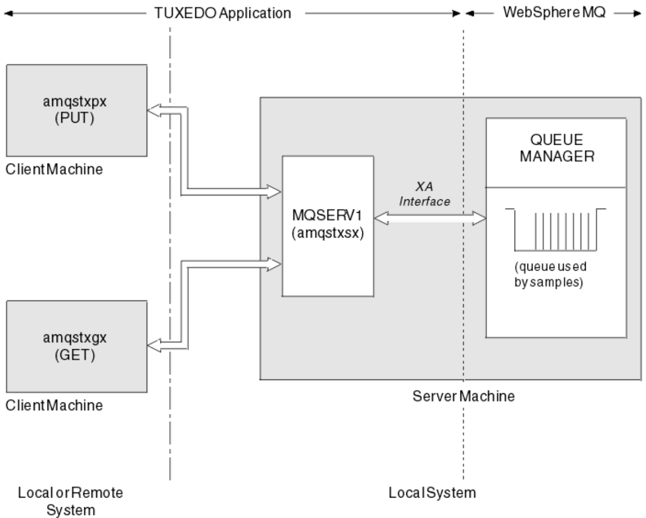
图 142: TUXEDO 样本如何协同工作
