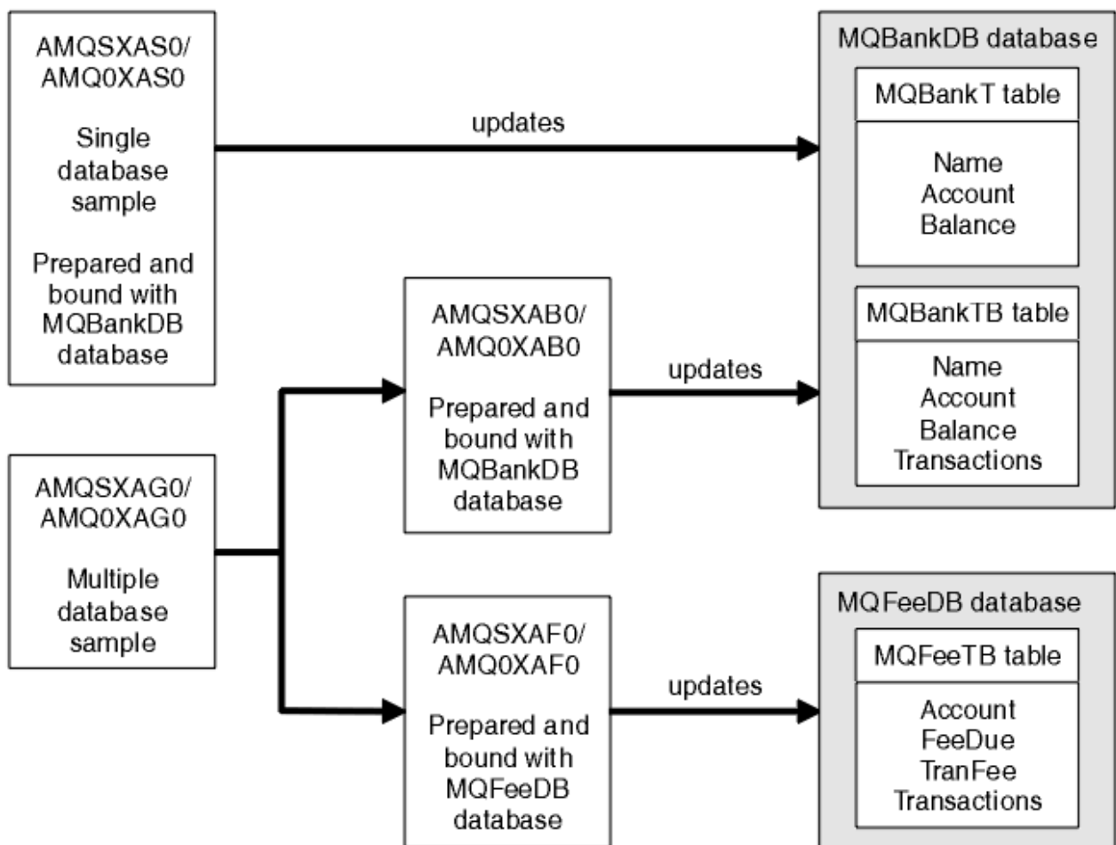
图 132: “数据库协调”样本
