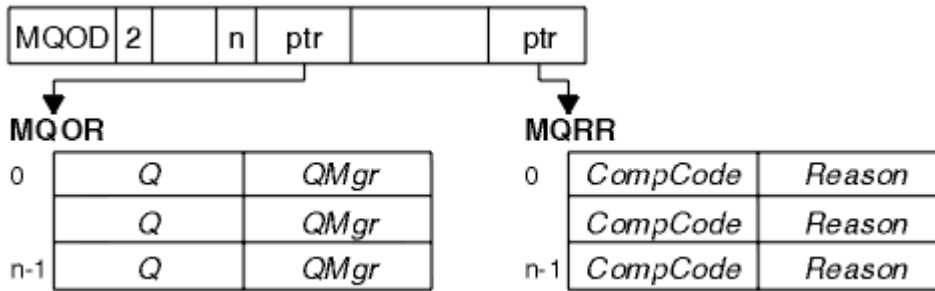
图 61: 在 C 中打开分发列表
