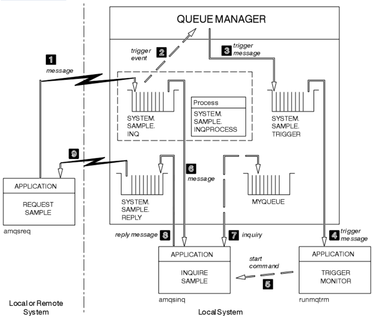
图 136: 使用触发机制的“请求”和“查询”样本
