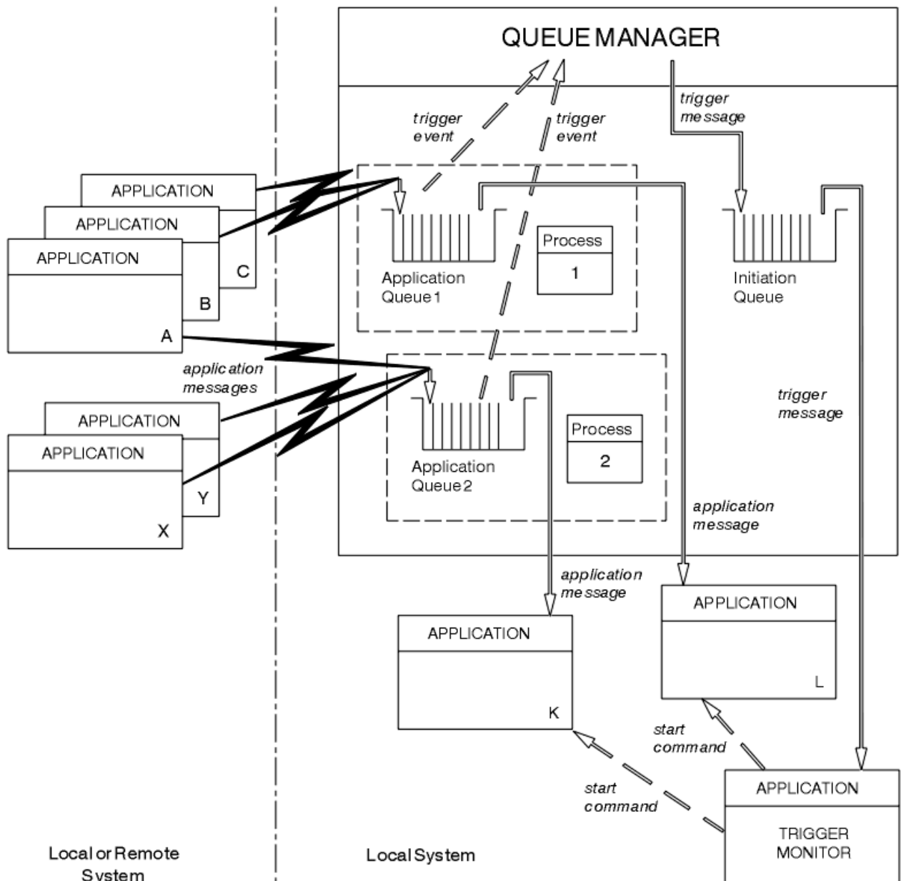
图 100: 触发内队列的关系
