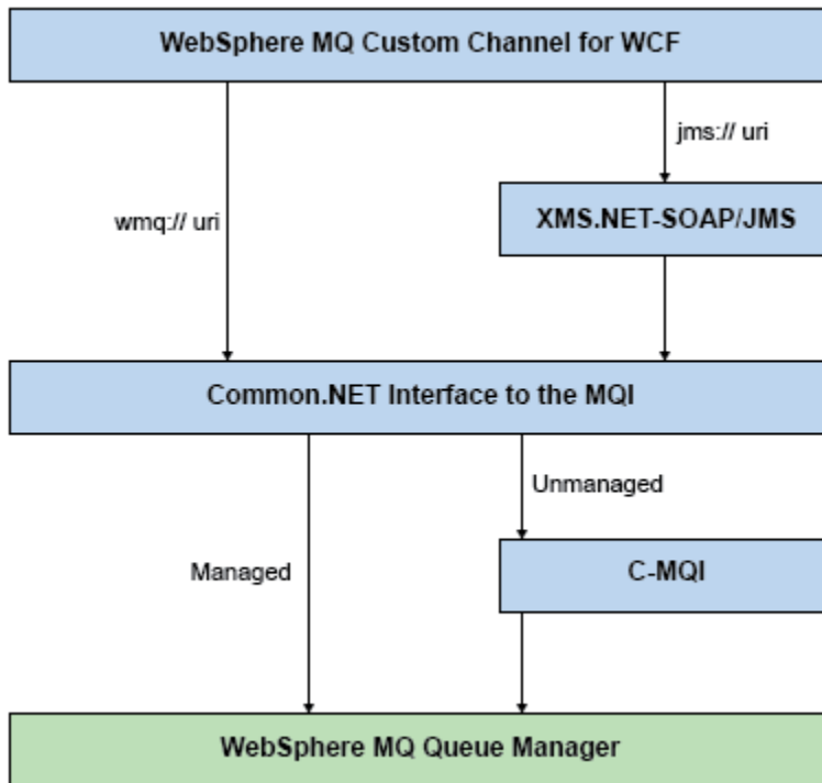
图 154: 面向非 SOAP/非 JMS 接口的 WCF 体系结构
