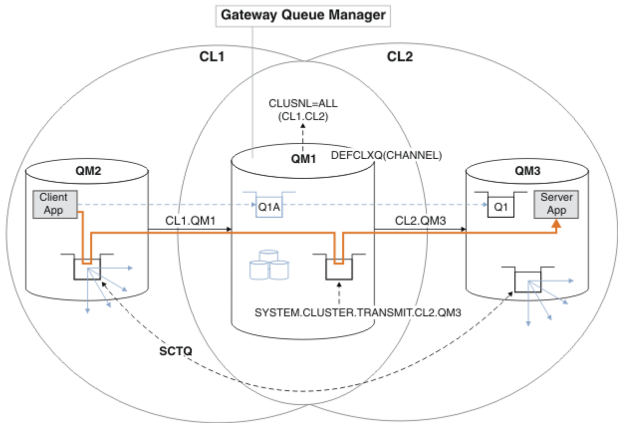
图 54: 客户机/服务器应用程序已部署到具有网关队列管理器上的独立集群传输队列的中心和辐射体系结构。
