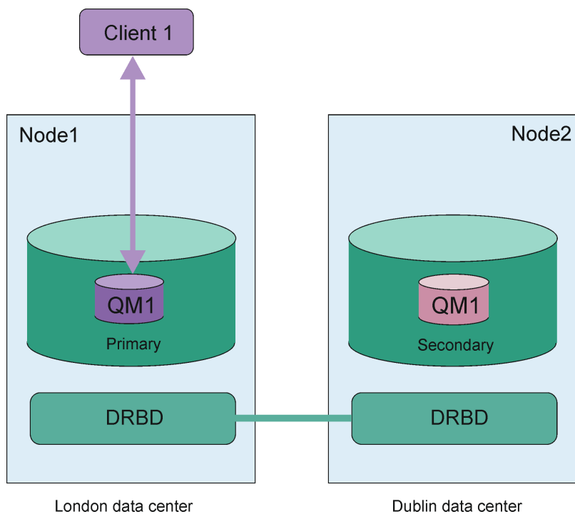
图 84: 单个 RDQM 对
