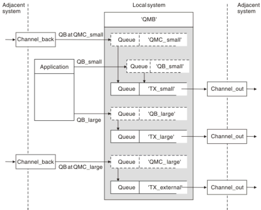
图 12: 分隔消息流
