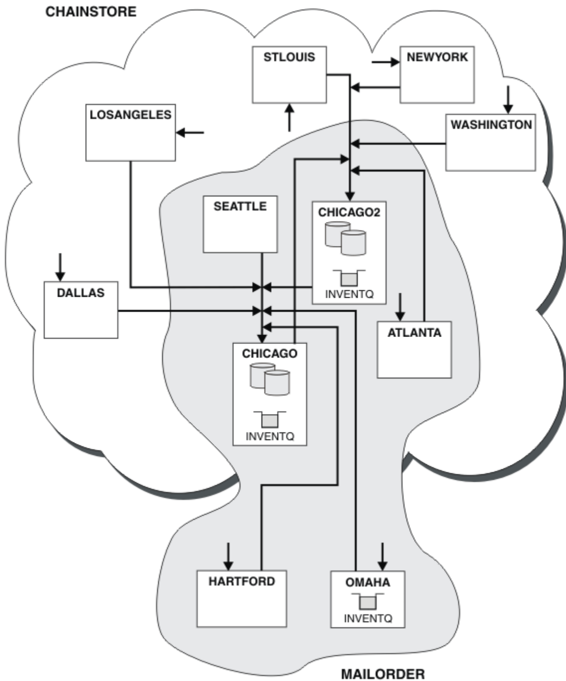
图 48: 互连集群
