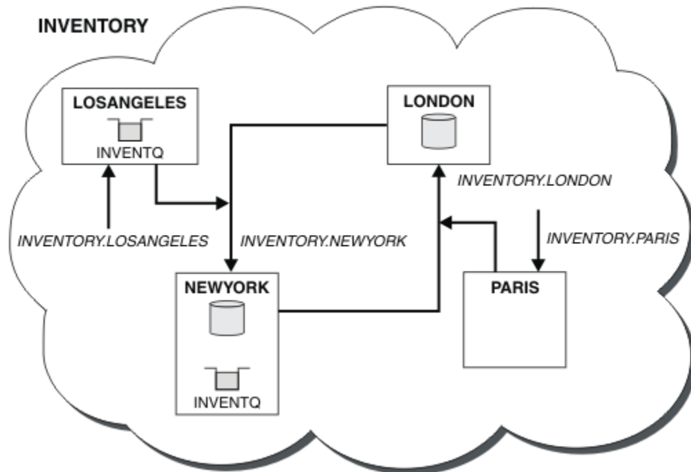
图 66: 具有四个队列管理器的 INVENTORY 集群
