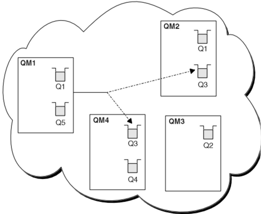
图 61: 具有同一队列的多个实例的集群
