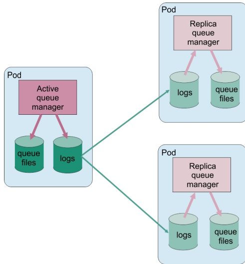
图 86: 本机 HA 配置示例
