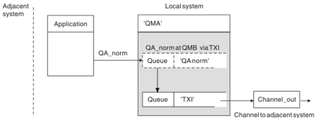
图 9: 远程队列定义允许使用其他传输队列
