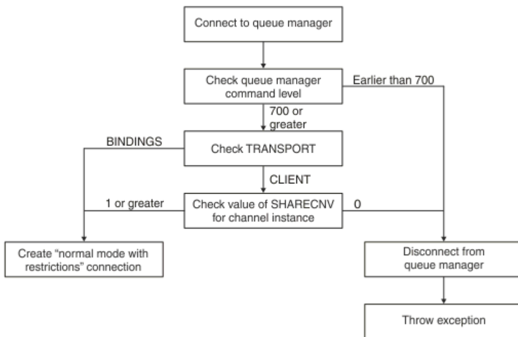
图 94: 具有限制的 PROVIDERVERSION 正常方式
