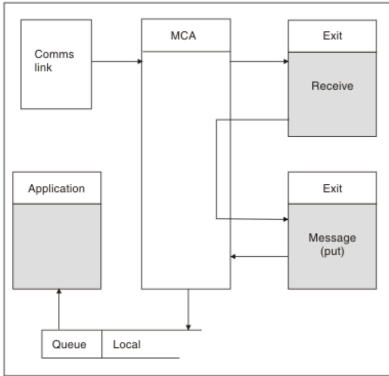
Şekil 109. İleti kanalının günlük nesnesindeki alma çıkışa örneği
