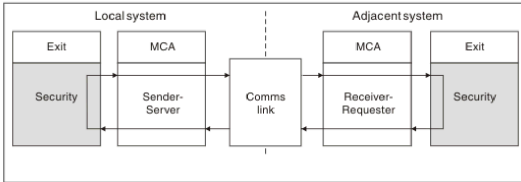
Şekil 107. Güvenlik çıkış döngüsü
