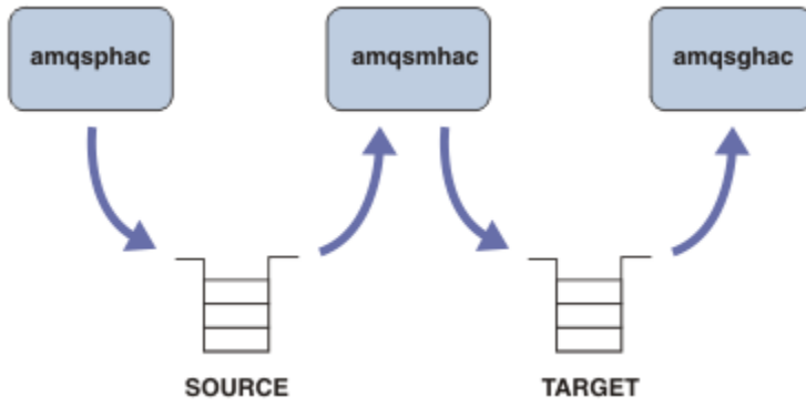
Şekil 133. Yeniden bağlanabilir istemci örnekleri
