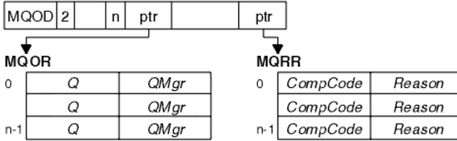
Şekil 61. C içinde bir dağıtım listesinin açılması
