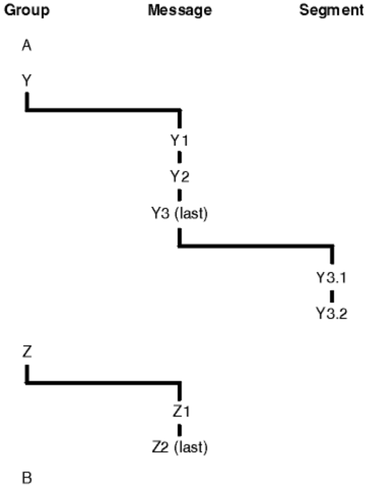
Şekil 65. Kuyruğun mantıksal sırası
