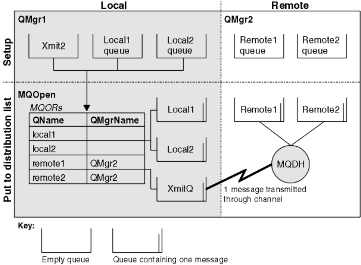
Şekil 60. Dağıtım listeleri nasıl çalışır
