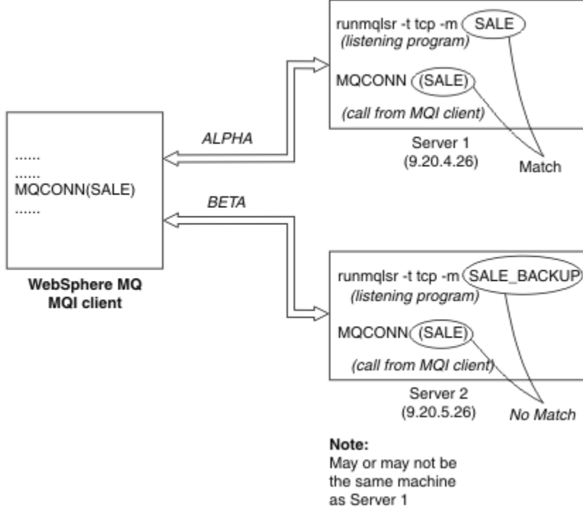
Şekil 102. MQCONN örneği
