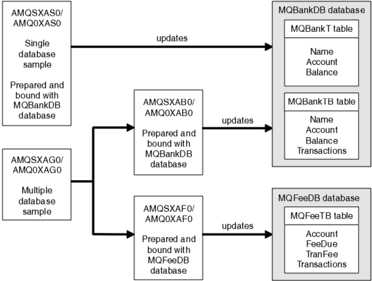
Şekil 132. Veritabanı koordinasyonu örnekleri
