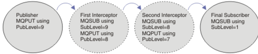
Şekil 90. Engellenen abonelerin sırası
