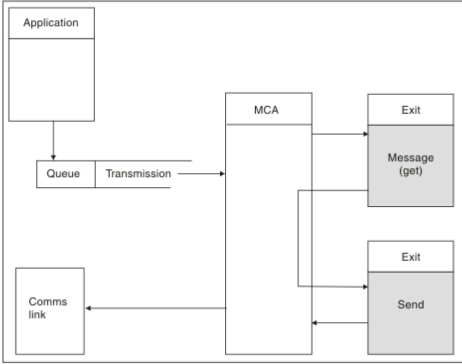
Şekil 108. İleti kanalının gönderici bitişindeki gönderme çıkışı örneği
