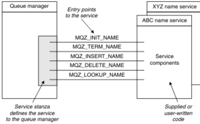
Şekil 103. Hizmetlerin, bileşenlerin ve giriş noktalarının anlaşılması
