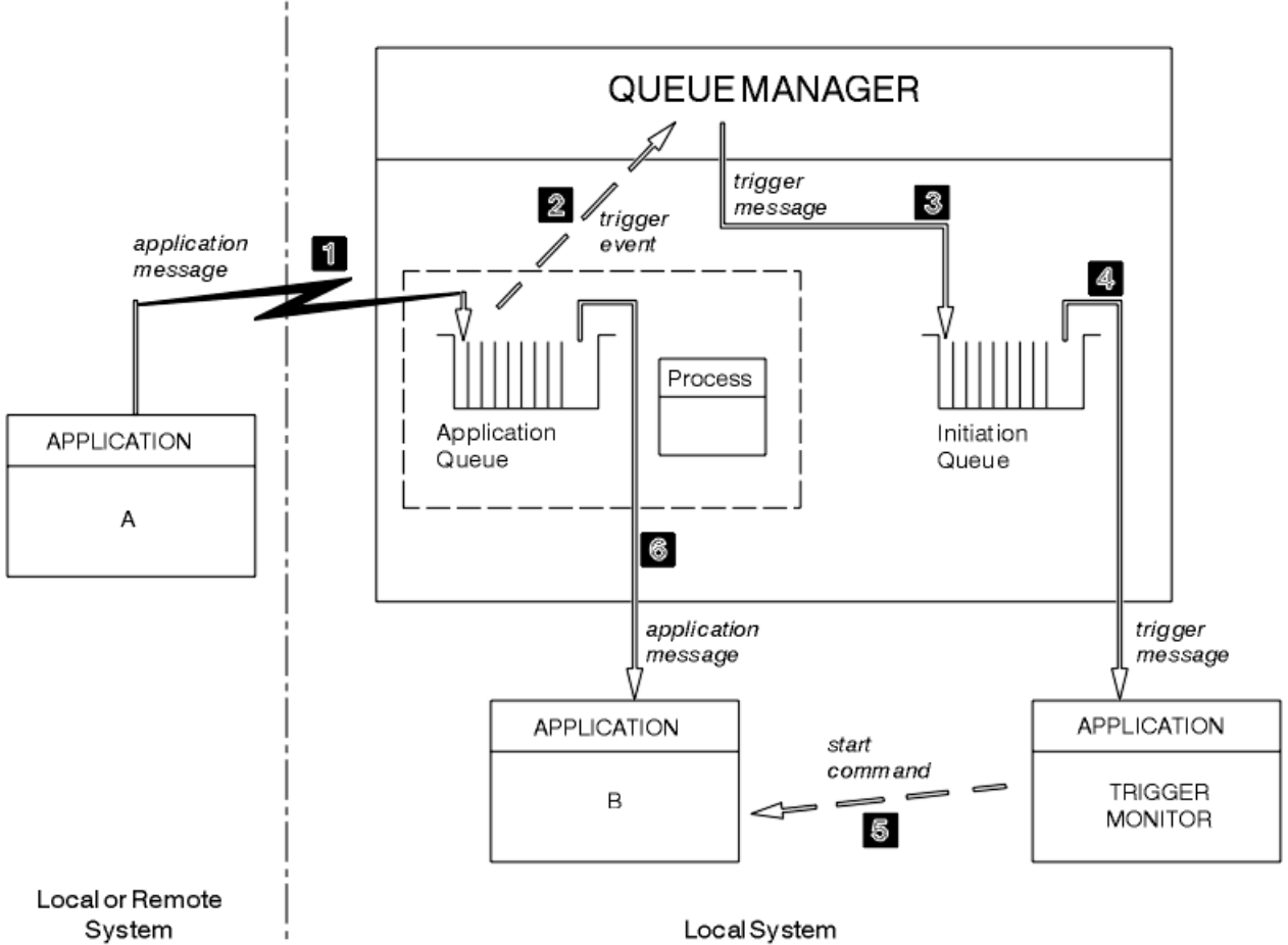
Şekil 99. Uygulama akışı ve tetikleme iletileri
