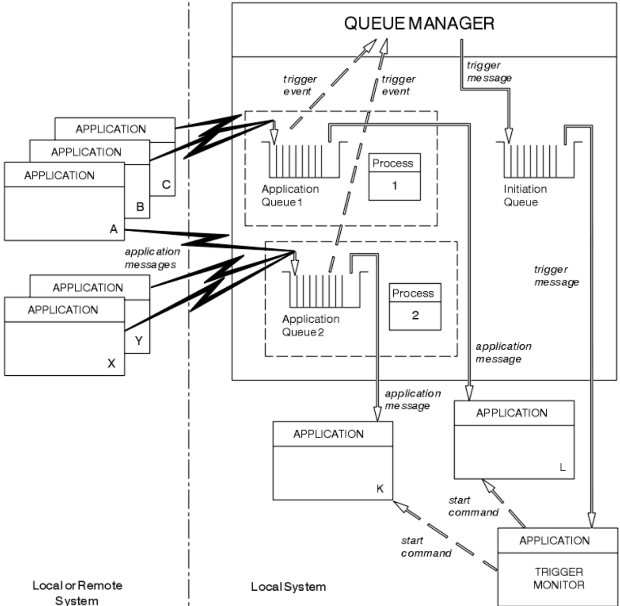
Şekil 100. Tetikleme içindeki kuyrukların ilişkisi
