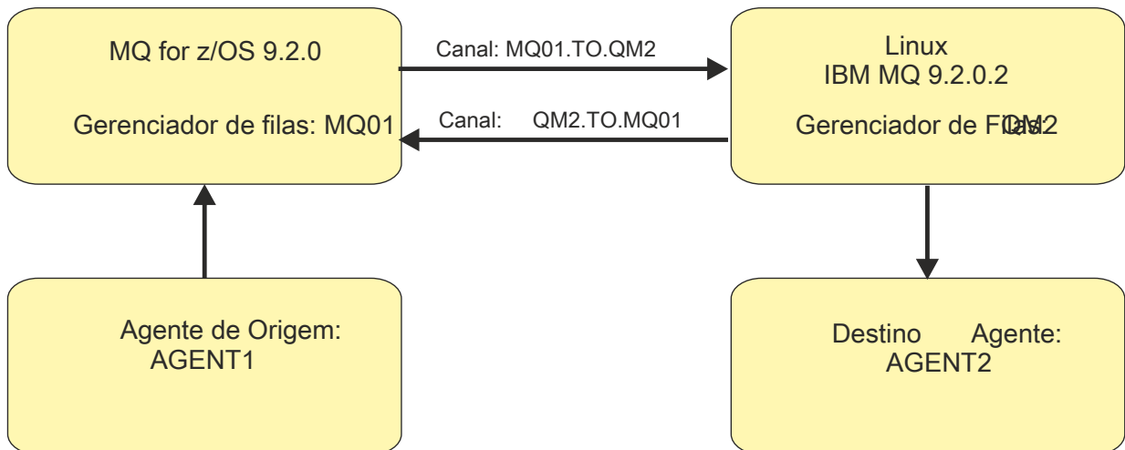
Figura 56. Exemplo de um diagrama simples mostrando como um agente de origem, AGENT1, e um agente de destino, AGENT2, e seus gerenciadores de filas do agente, MQ01 e QM2 estão conectados.
