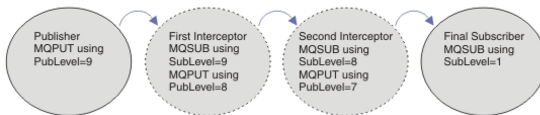
Figura 90. Sequência de assinantes de interceptação
