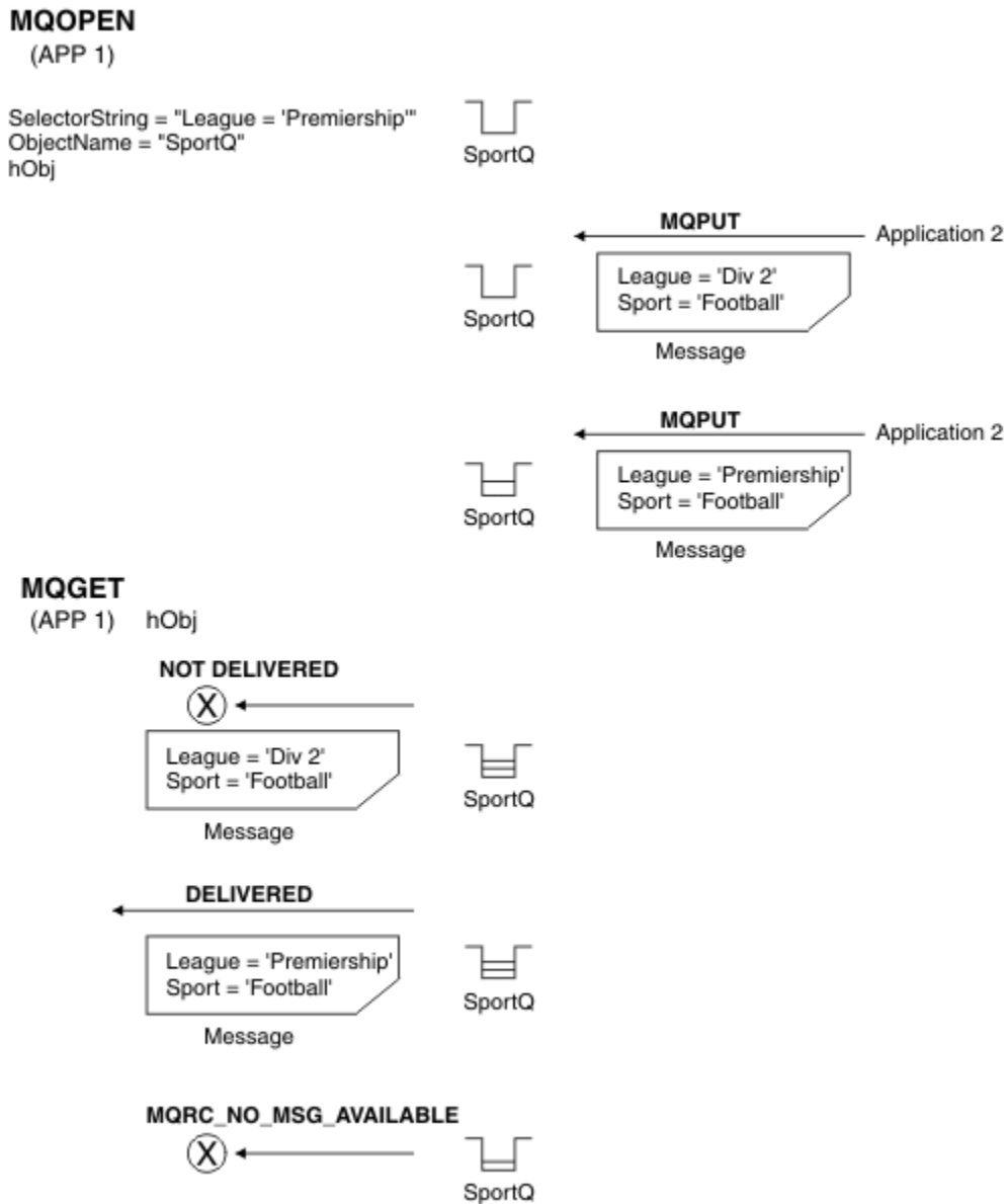
Figura 4. Seleção usando a chamada MQOPEN
