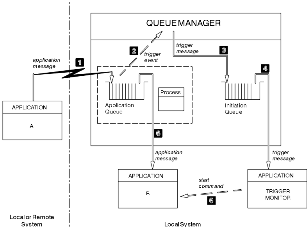
Figura 99. Fluxo de mensagens do aplicativo e do acionador
