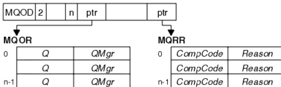
Figura 61. Abrindo uma lista de distribuição em C
