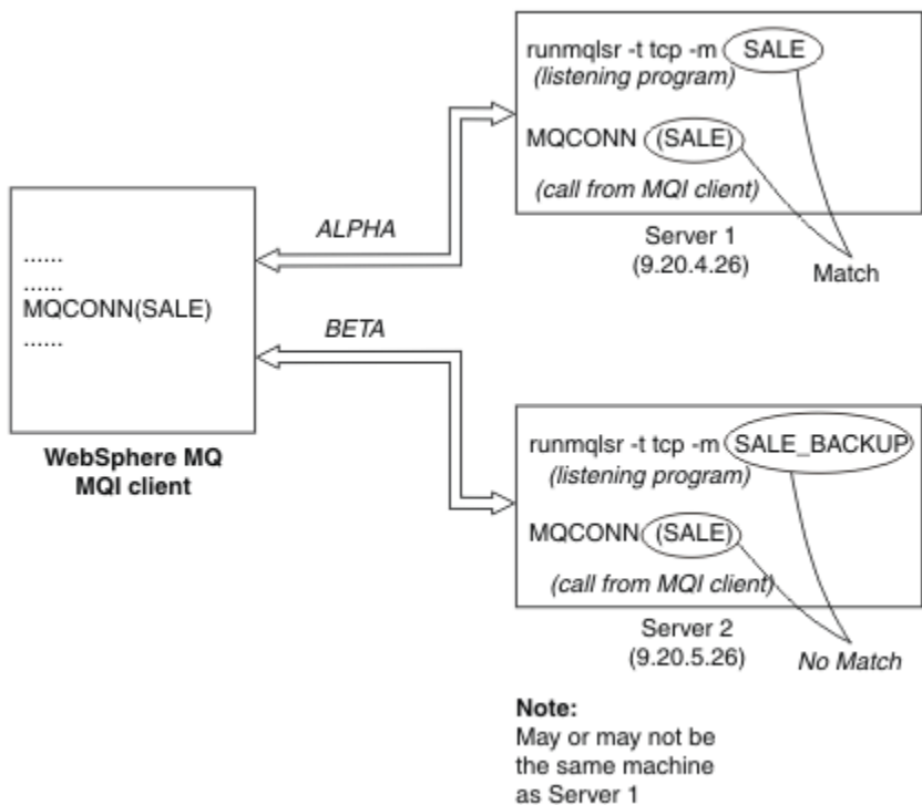
Figura 102. Exemplo de MQCONN
