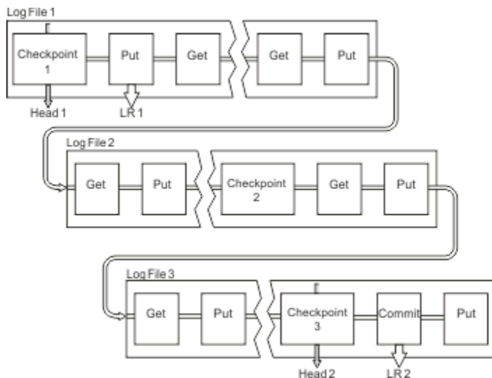
Figura 88. Ponto de verificação com uma transação de execução longa
