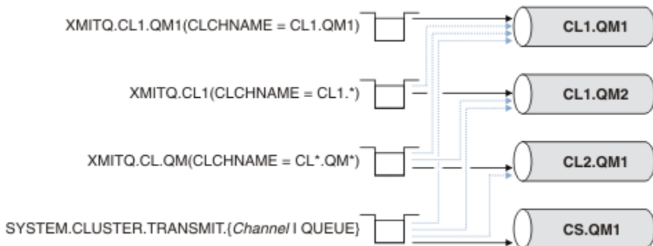
Figura 39. Precedência de Fila de Transmissão / Canal do Emissor de Clusters
