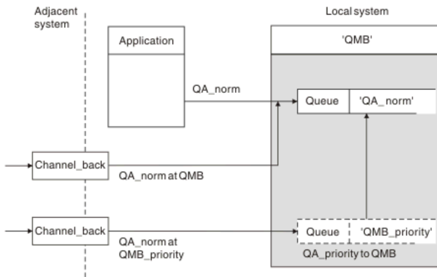
Figura 10. Recebendo Mensagens diretamente e resolução de alias do nome do gerenciador de filas
