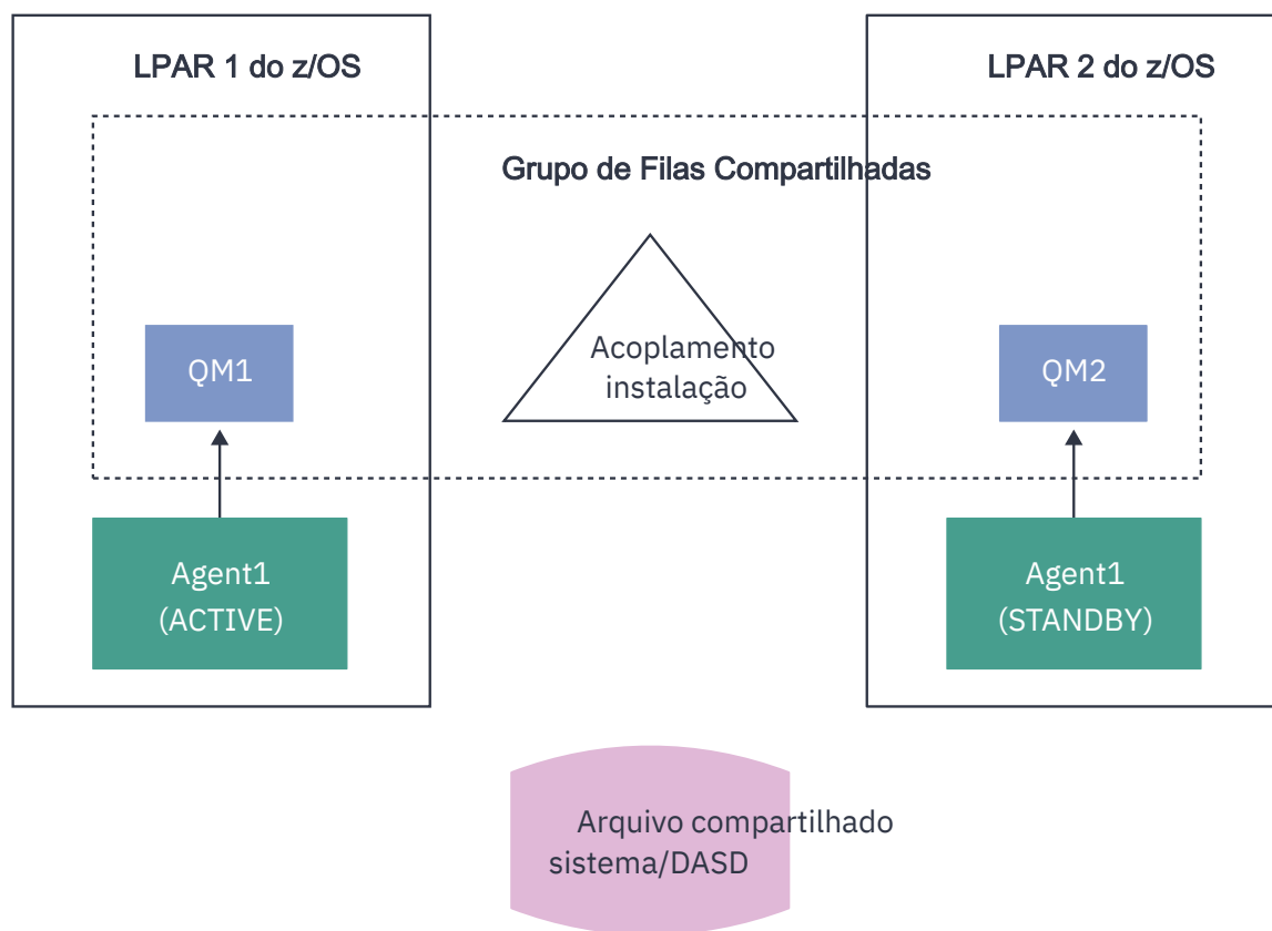
Figura 98. Agente do MFT altamente disponível usando um grupo de filas compartilhadas
