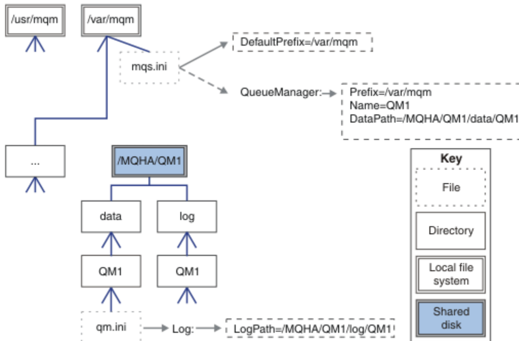
Figura 73. Diretórios nomeados compartilhados data e log
