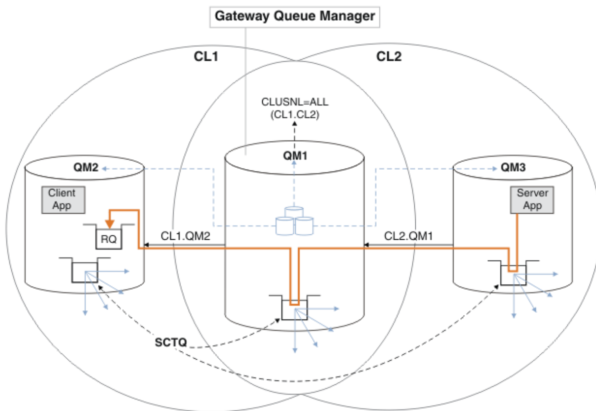
Figura 50. Usando um Alias de Gerenciador de Filas para retornar a mensagem de resposta para um cluster diferente
