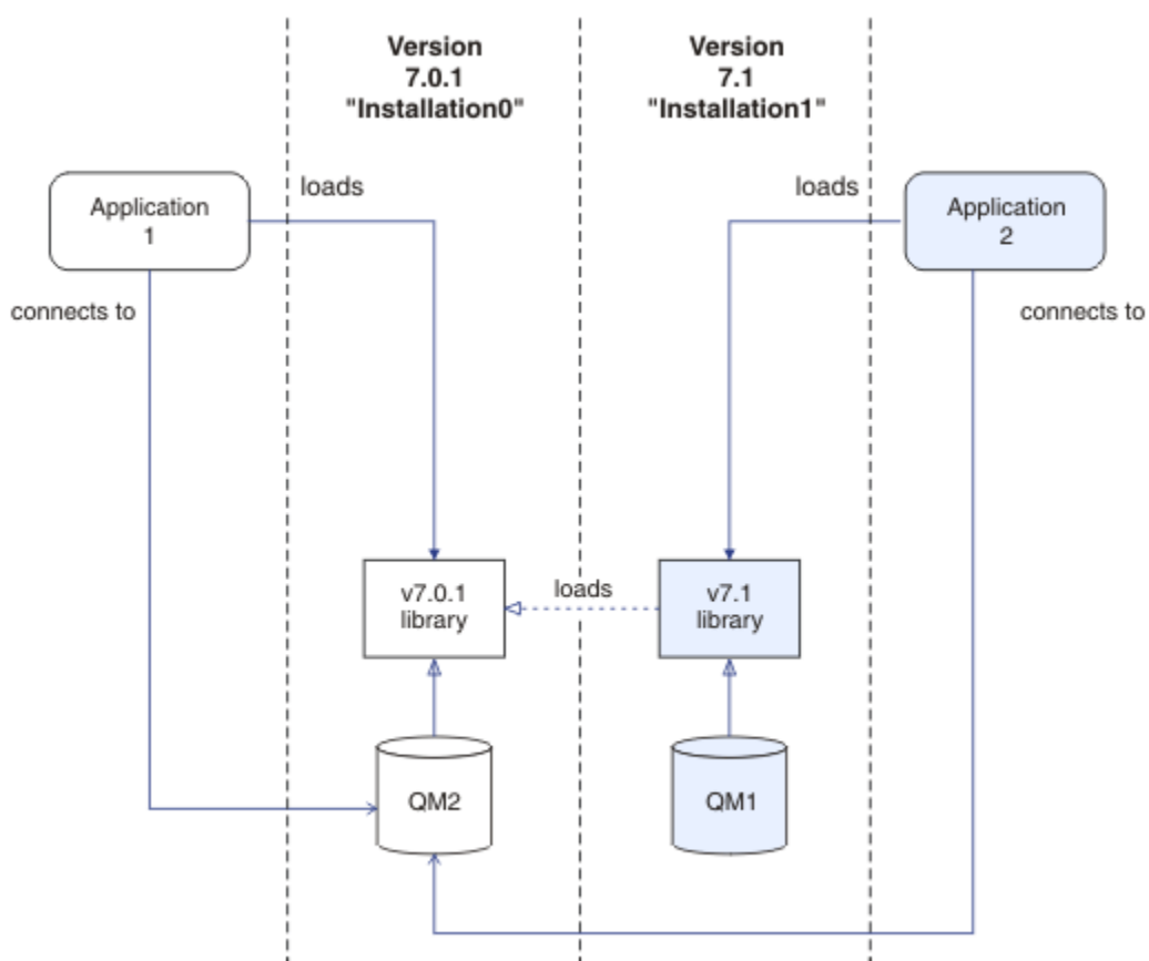
Figura 70. Conectando Aplicativos em um Ambiente com Diversas Instalações
