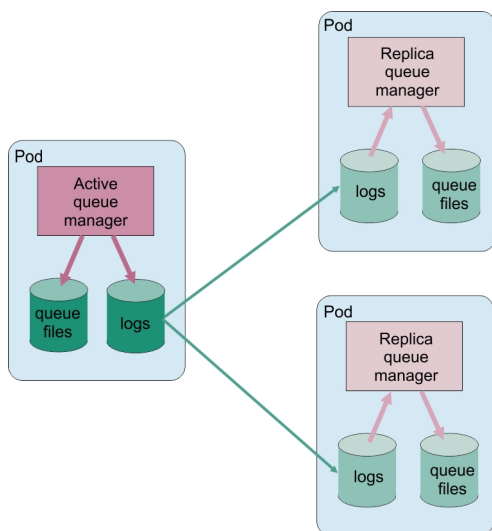
Figura 86. Exemplo de configuração de HA nativa
