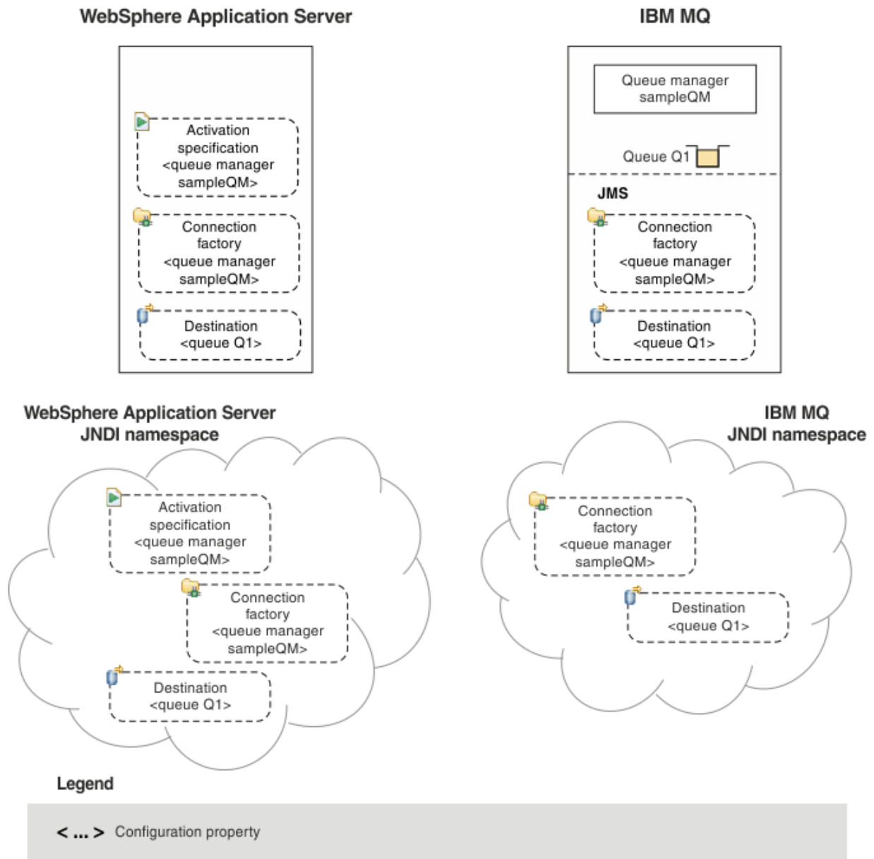
Figura 91. Objetos criados em WebSphere Application Server e os objetos correspondentes em IBM MQ
