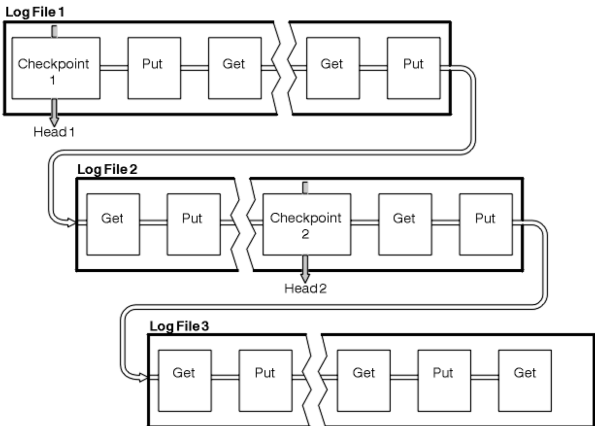
Figura 87. Ponto de verificação
