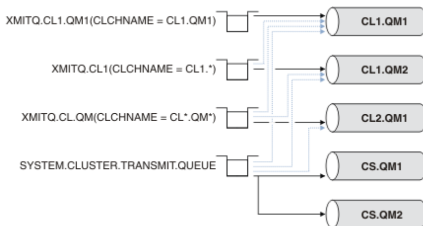
Figura 40. Diversos Canais do Emissor de Clusters
