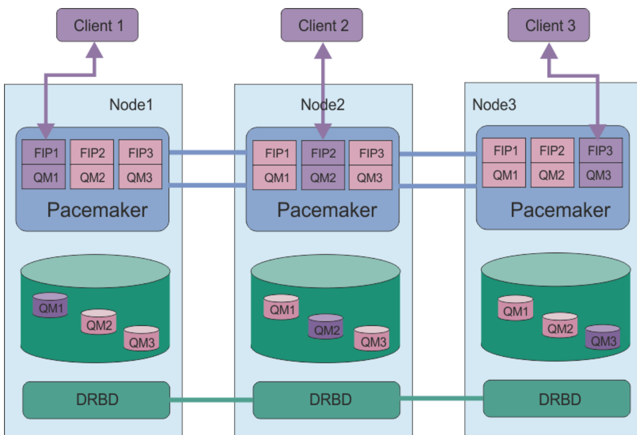
Figura 81. Exemplo de grupo de HA com três RDQMs
