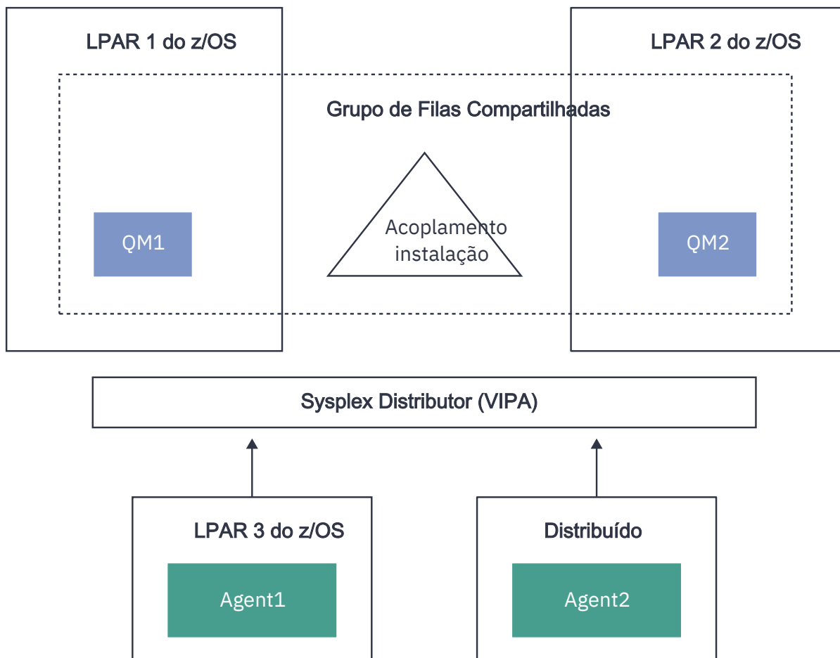
Figura 99. Agentes do MFT conectando-se a um grupo de filas compartilhadas como um cliente
