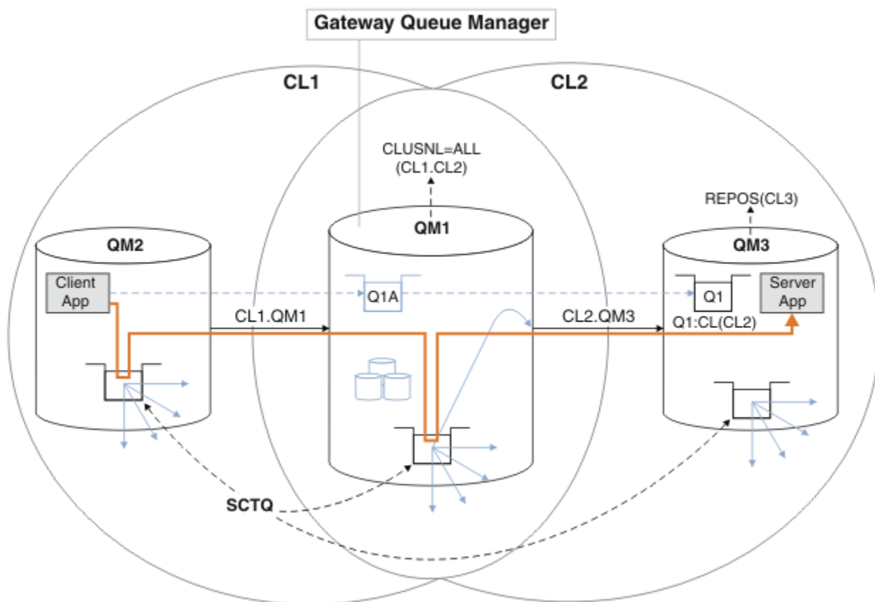
Figura 49. Aplicativo cliente-servidor implementado na arquitetura hub e spoke usando os clusters IBM MQ
