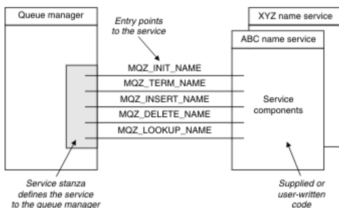
Rysunek 103. Zrozumienie usług, komponentów i punktów wejścia
