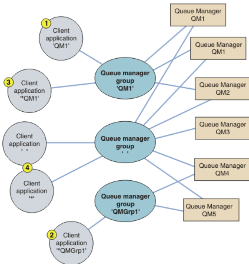
Rysunek 101. Grupy menedżerów kolejek
