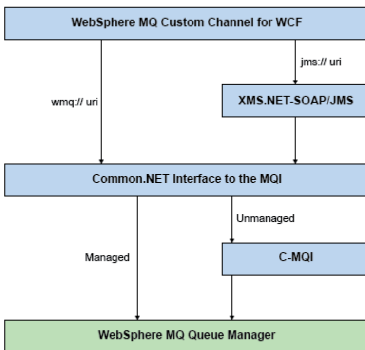
Rysunek 154. Architektura WCF dla interfejsu Non-SOAP/Non-JMS
