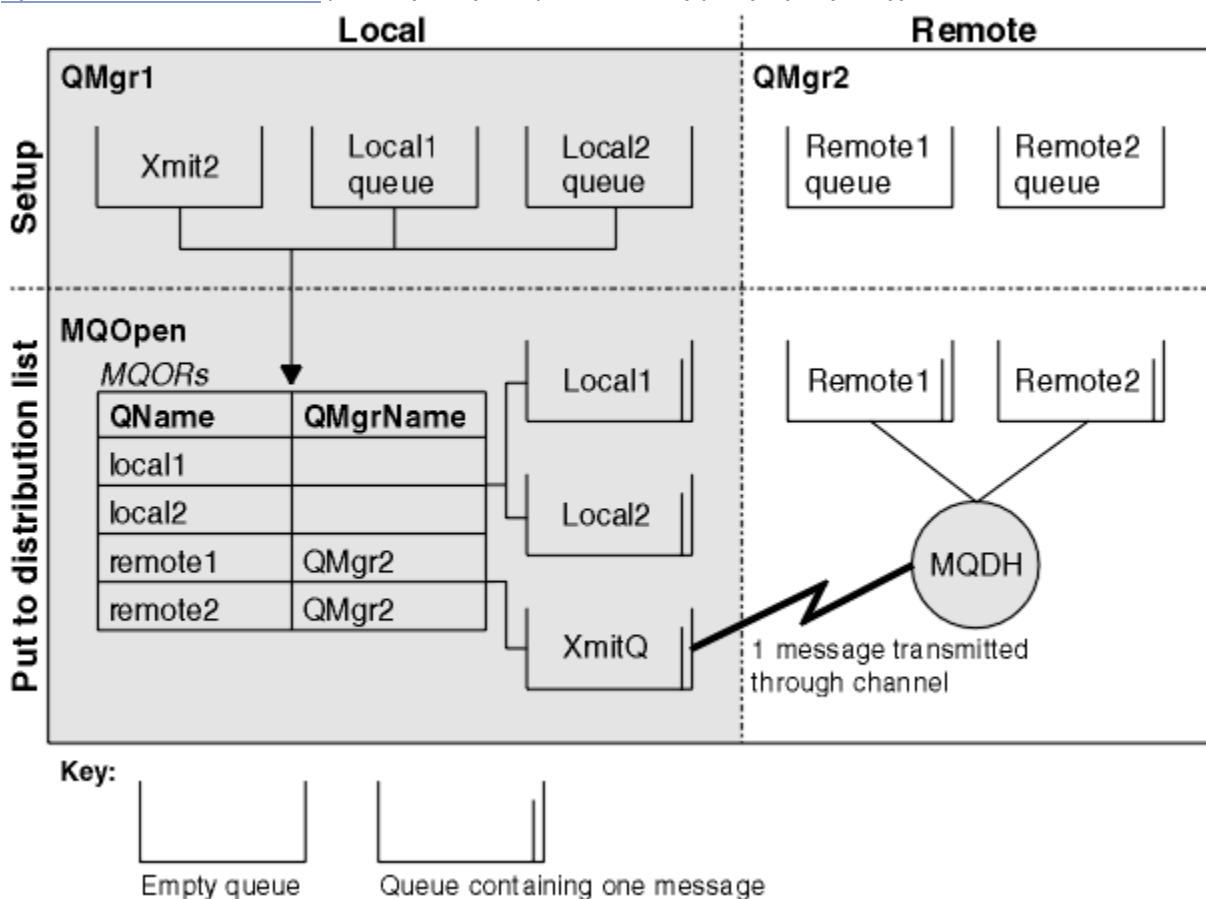
Rysunek 60. Sposób działania list dystrybucyjnych
