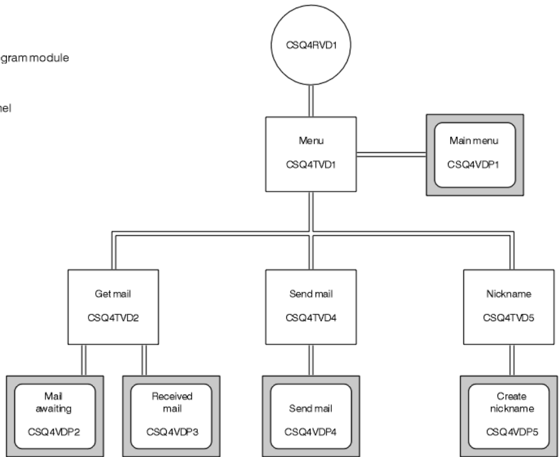
Rysunek 144. Programy i panele dla wersji TSO programu Mail Manager
