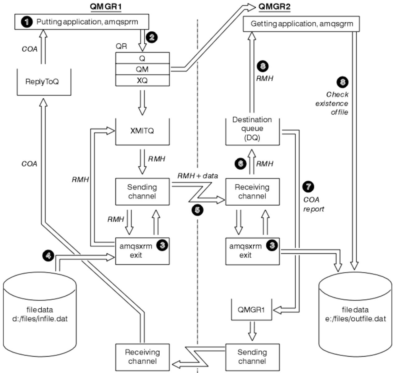
Rysunek 135. Uruchamianie przykładów komunikatów odniesienia
