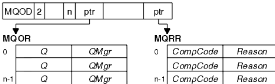
Rysunek 61. Otwieranie listy dystrybucyjnej w języku C
