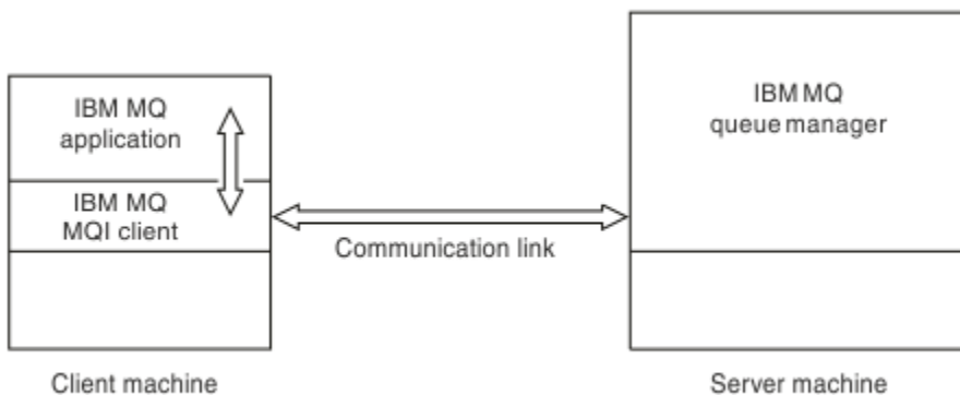
그림 52. 클라이언트와 서버 사이의 링크
