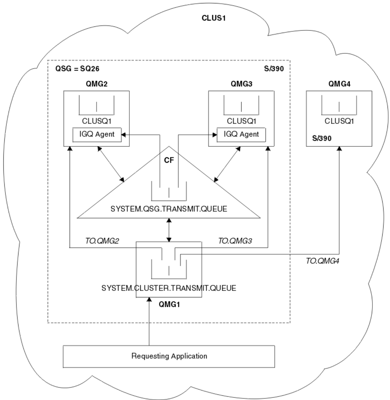
그림 71. 그룹 내 큐잉을 포함한 클러스터링 예제
