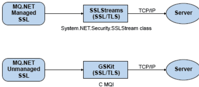
그림 51. IBM MQ.NET 관리 및 비관리 TLS 비교
