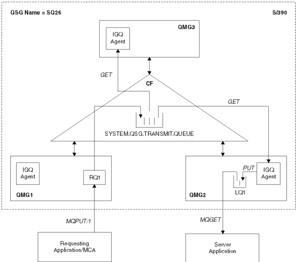
그림 68. 그룹 내 큐잉 예
