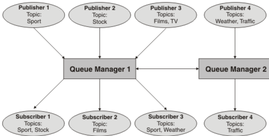
그림 33. 큐 관리자가 2개인 발행/구독 예제
