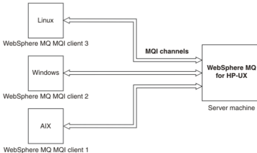
그림 53. 다른 플랫폼의 클라이언트에 연결된 IBM MQ 서버
