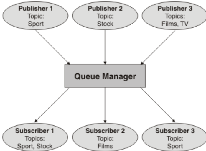
그림 32. 단일 큐 관리자 발행/구독 예제
