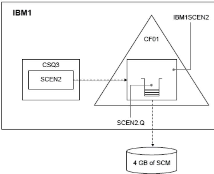
그림 65. 성능 향상을 위해 SCM을 추가하는 구성
