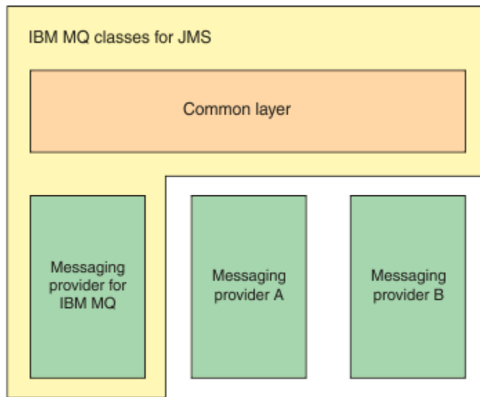
그림 55. IBM JMS 제공자를 위한 계층 아키텍처
