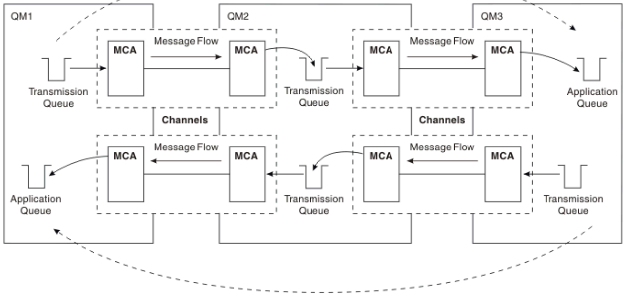
그림 12. 중간 큐 관리자를 통해 전달
