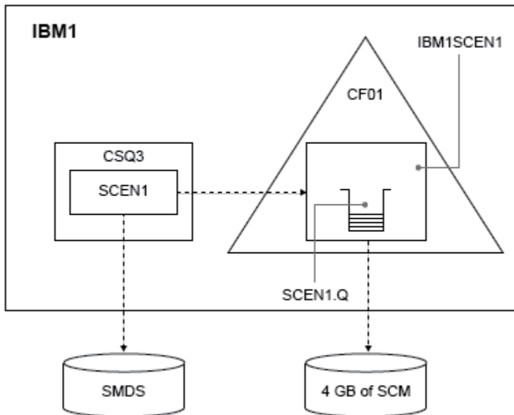
그림 63. 응급 스토리지용 SMDS 및 SCM을 추가하는 구성
