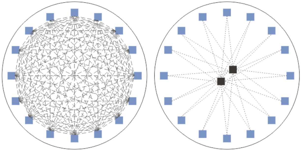
그림 36. 직접 라우팅 및 토픽 호스트 라우팅
