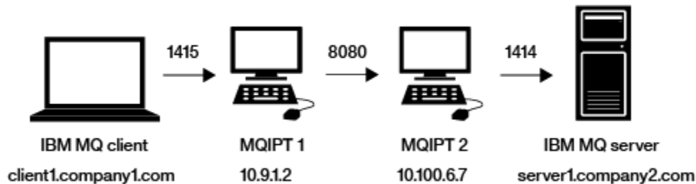
그림 33. HTTP 터널링 네트워크 다이어그램
