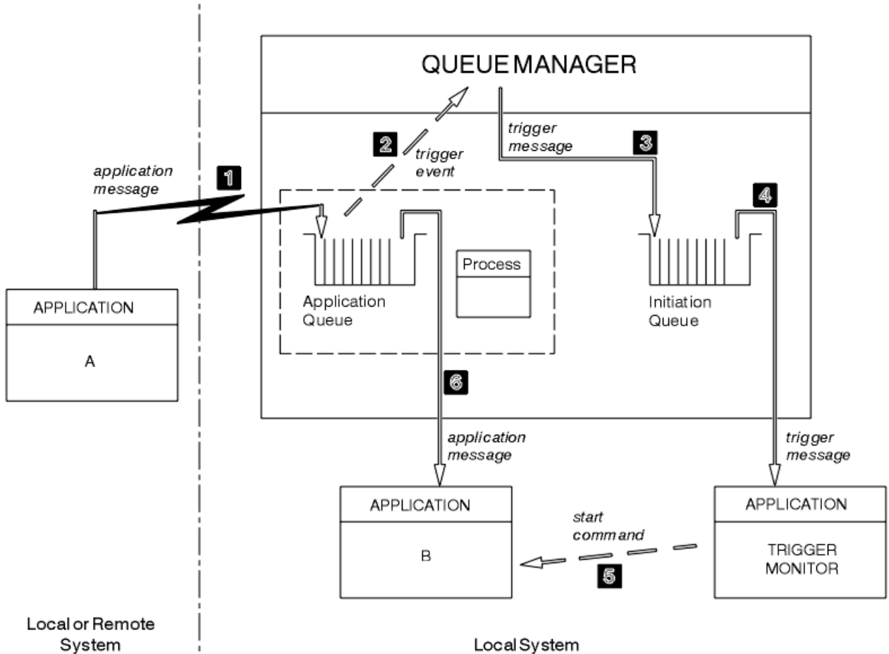
그림 99. 애플리케이션 및 트리거 메시지의 플로우
