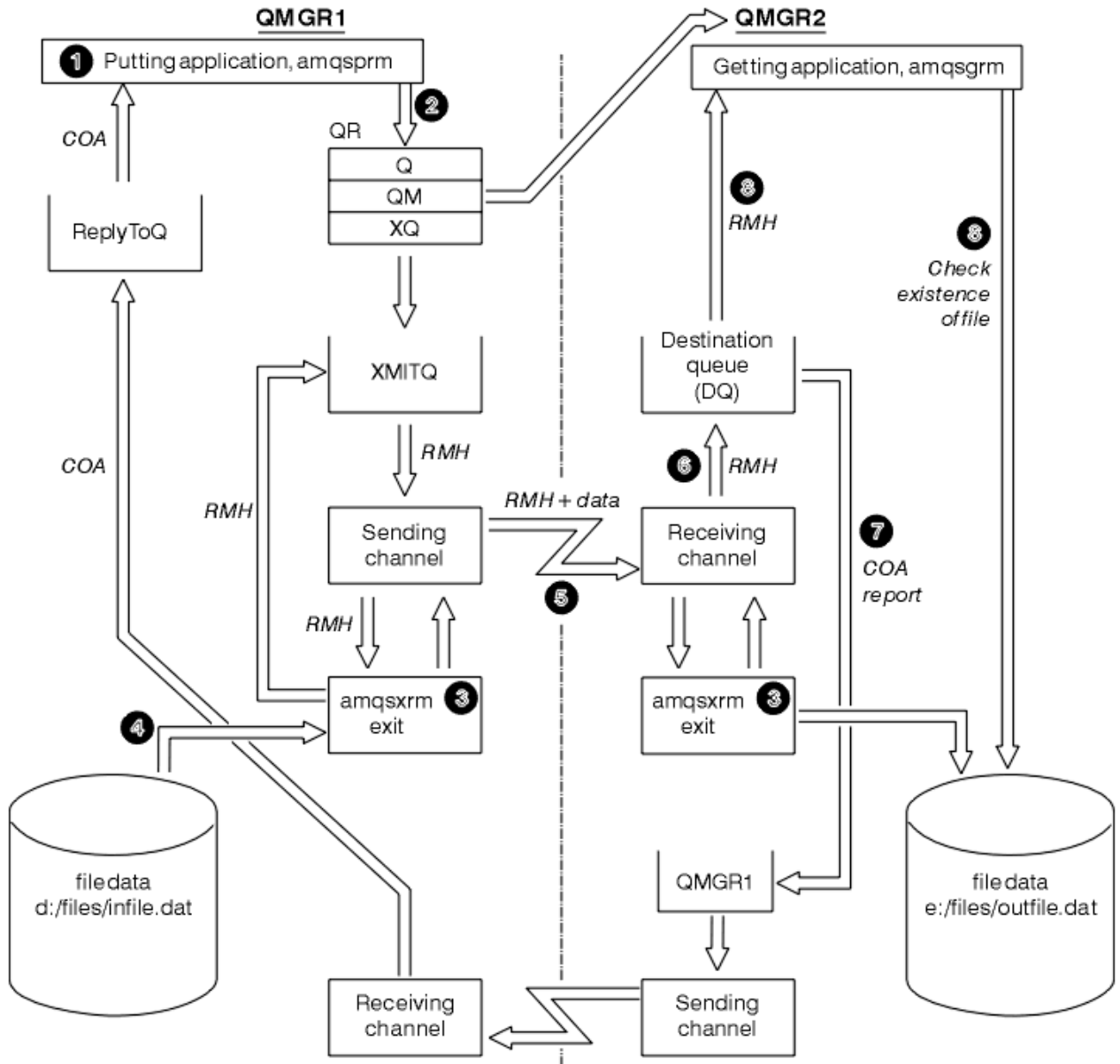
그림 135. 참조 메시지 샘플 실행
