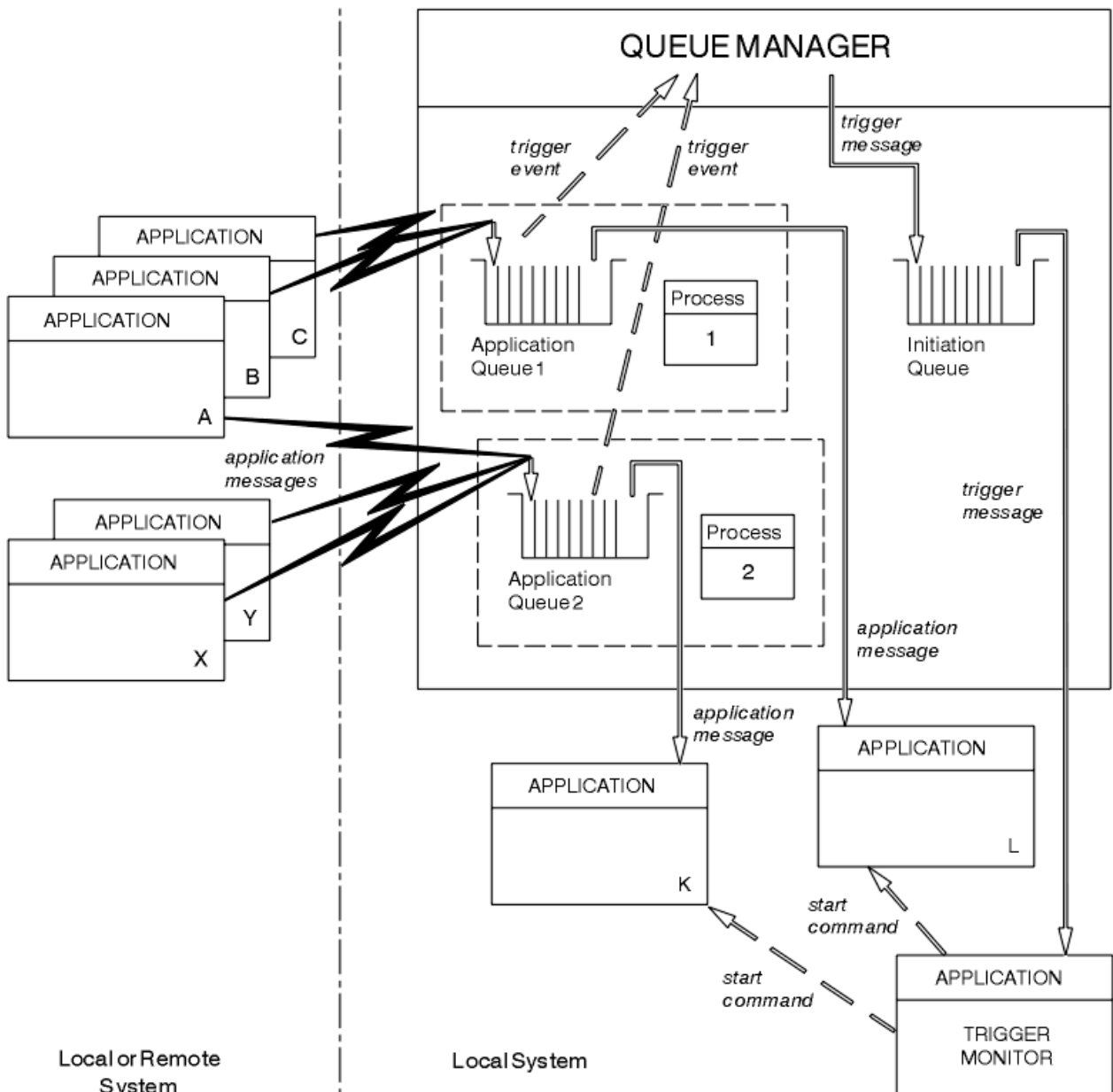
그림 100. 트리거 내에 있는 큐의 관계
