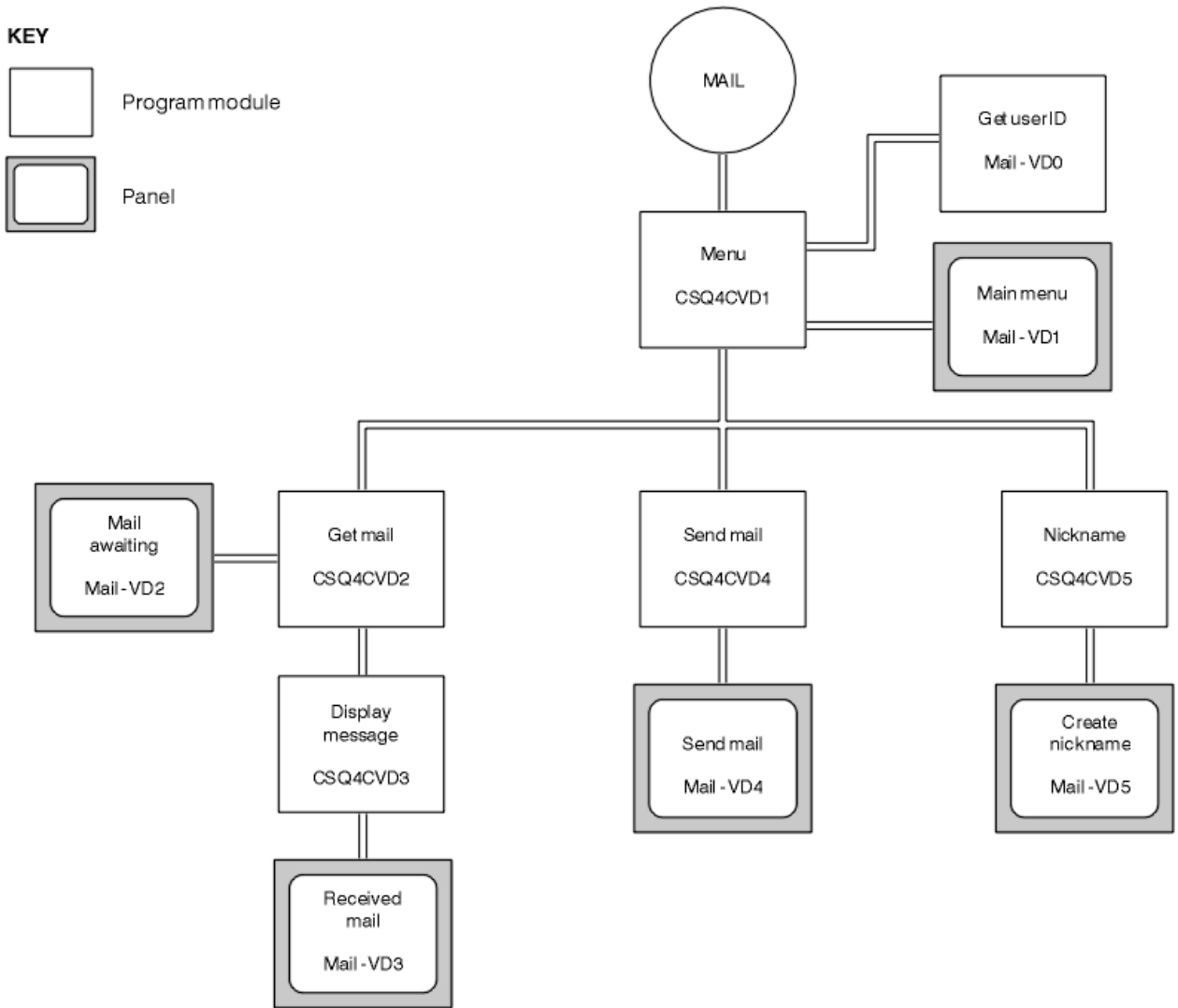
그림 145. 메일 관리자의 CICS 버전에 대한 프로그램 및 패널
