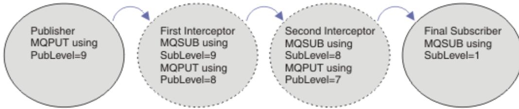
그림 90. 인터셉트 구독자의 순서
