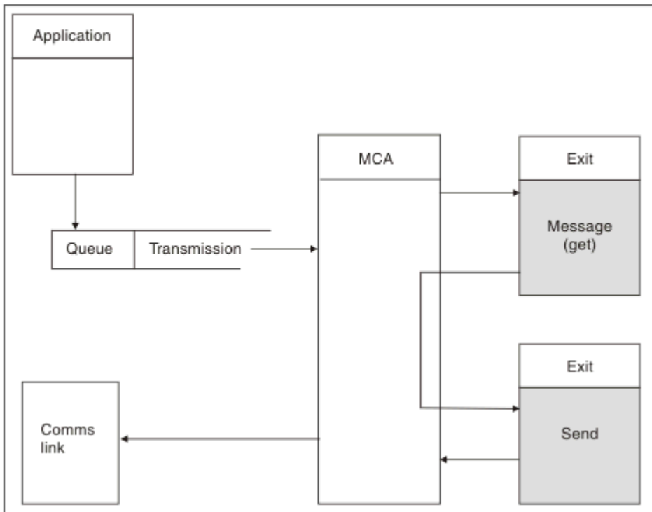
그림 108. 메시지 채널의 송신자 끝에서의 송신 엑시트의 예
