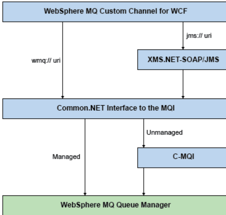
그림 154. 비SOAP/비JMS 인터페이스의 WCF 아키텍처
