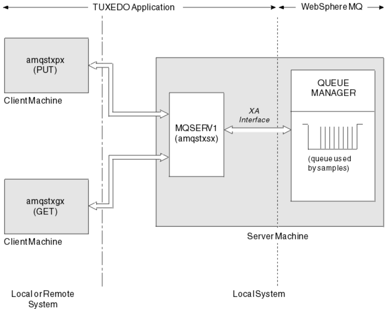
그림 142. TUXEDO 샘플이 함께 작동하는 방법
