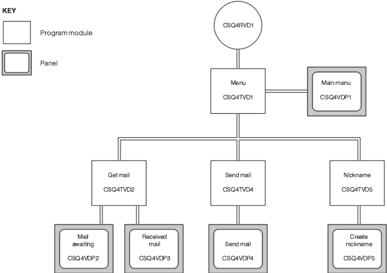
그림 144. 메일 관리자의 TSO 버전에 대한 프로그램 및 패널
