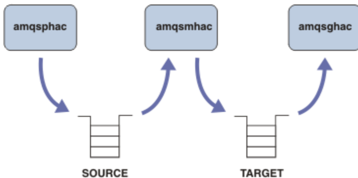
그림 133. 다시 연결 가능한 클라이언트 샘플
