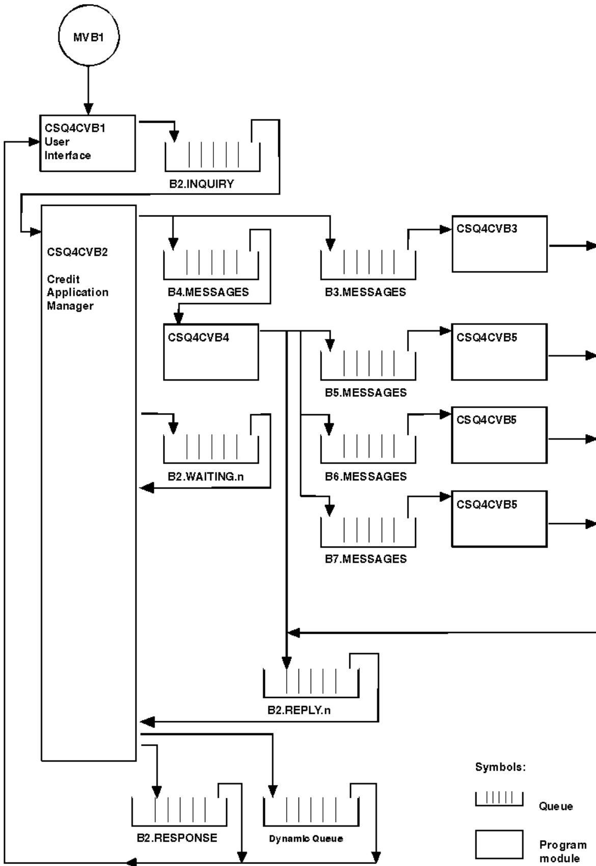
그림 149. 신용 조회 샘플 애플리케이션에 대한 프로그램 및 큐(COBOL 프로그램 전용)
