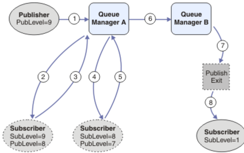
그림 97. 클러스터의 인터셉션 및 발행 엑시트
