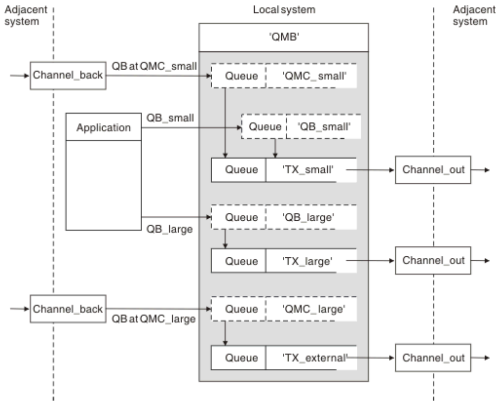
그림 12. 메시지 플로우 분리
