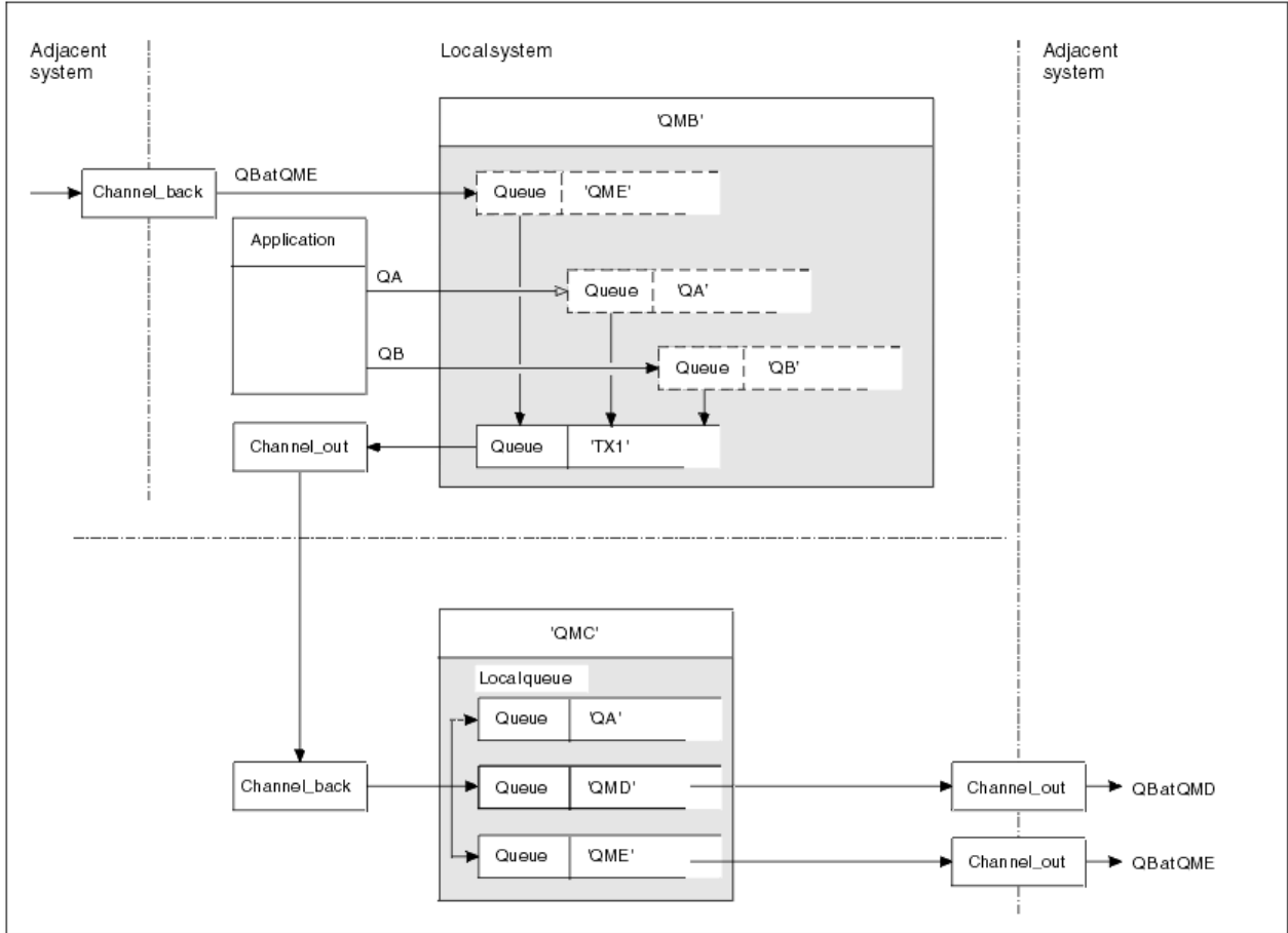
그림 13. 채널에 메시지 플로우 결합
