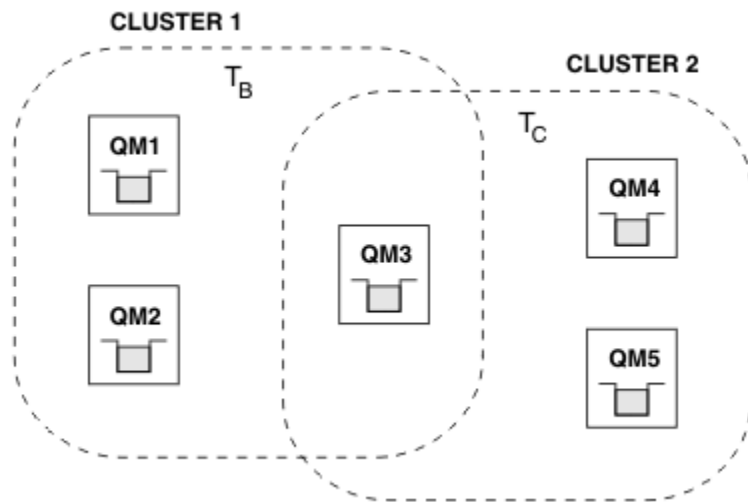
그림 69. 클러스터는 중첩되고 토픽 공간은 중첩되지 않는 경우
