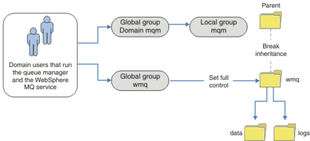
그림 77. 대체 글로벌 보안 그룹을 사용하여 큐 관리자 데이터 및 로그 보안 설정(2)
