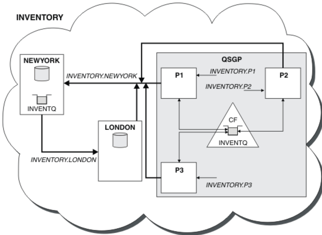
그림 45. 클러스터 및 큐 공유 그룹
