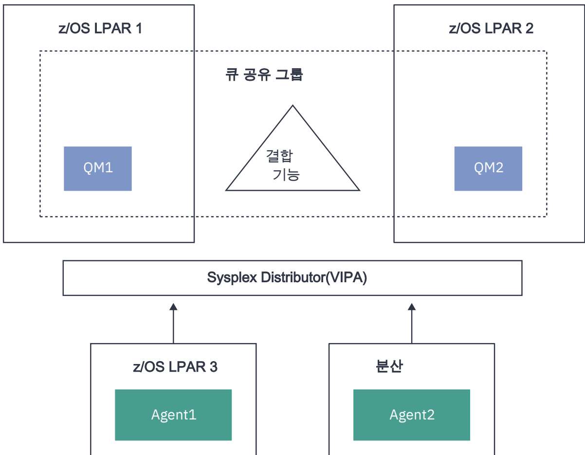
그림 99. 클라이언트로 큐 공유 그룹에 연결하는 MFT 에이전트
