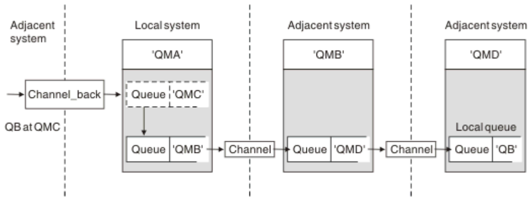
그림 14. 메시지 스트림을 다른 목적지로 전환
