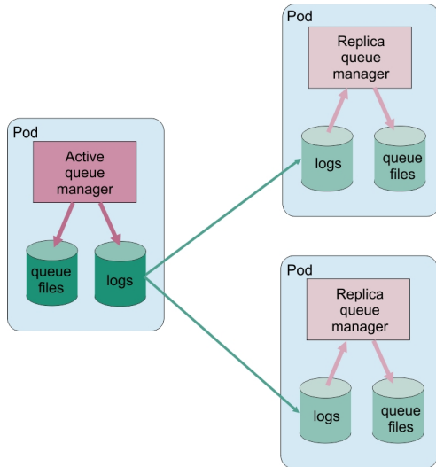
그림 86. 고유 HA 구성의 예제
