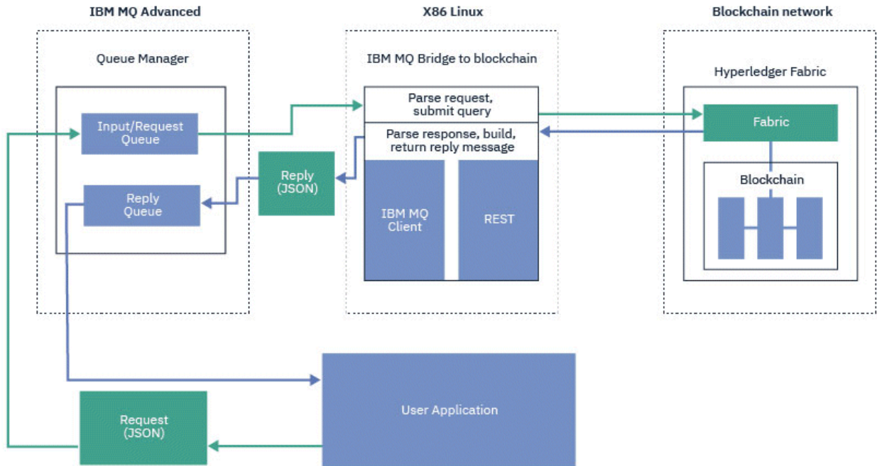
그림 101. IBM MQ Bridge to blockchain
