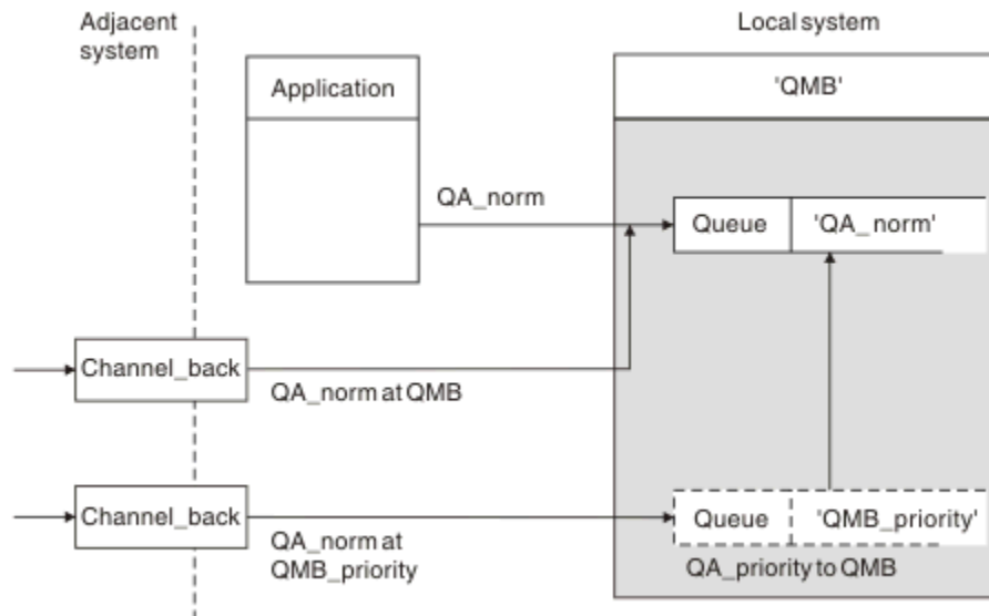
그림 10. 직접적인 메시지 수신과 알리어스 큐 관리자 이름 해석
