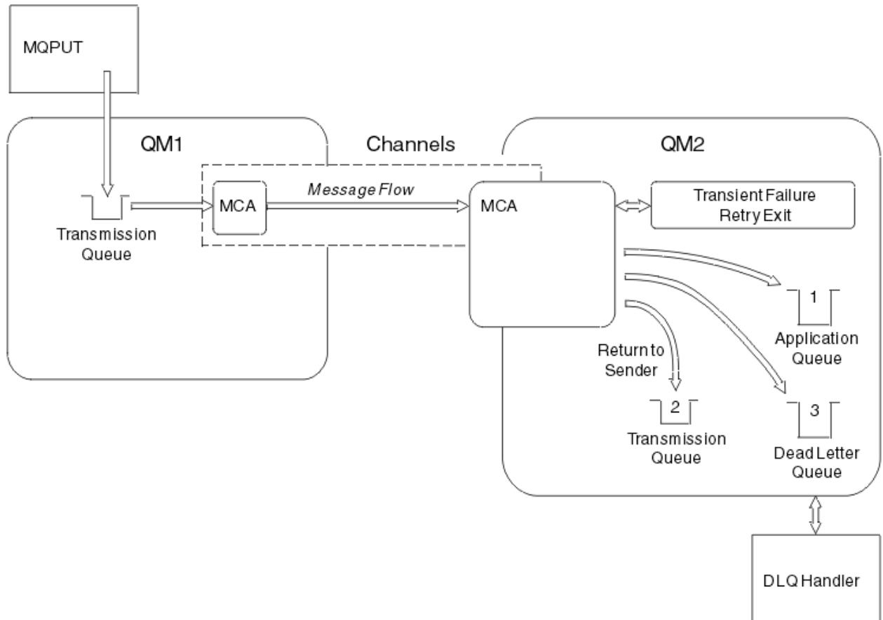
그림 25. 메시지를 전달할 수 없는 경우 발생하는 결과
