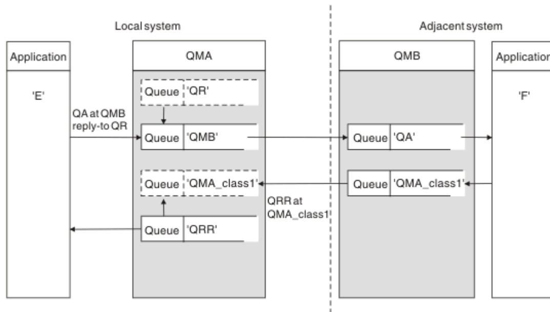
그림 15. PUT 호출 시 응답 대상 큐 이름 대체
