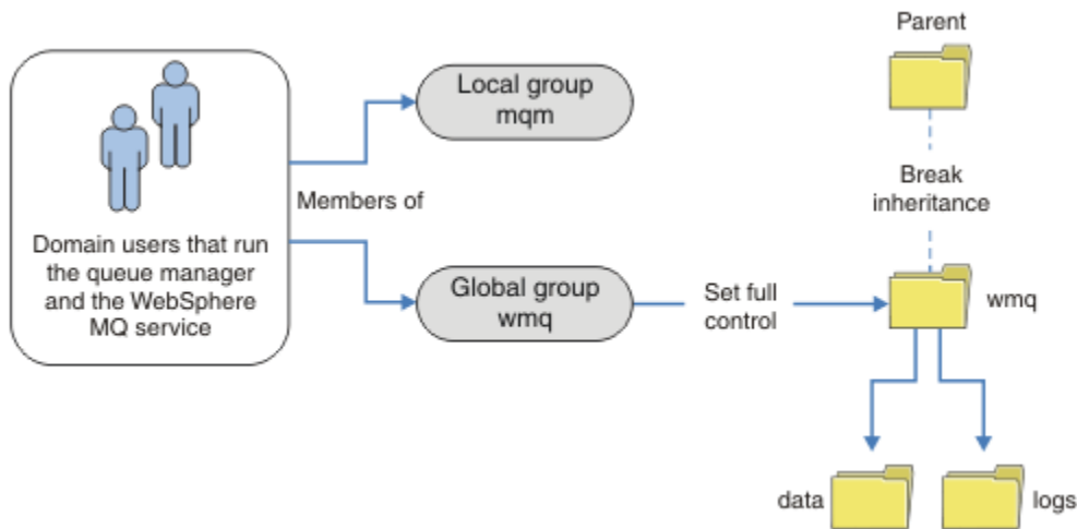
그림 76. 대체 글로벌 보안 그룹을 사용하여 큐 관리자 데이터 및 로그 보안 설정(1)
