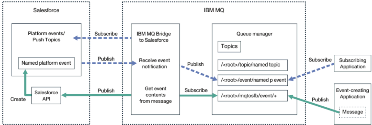
그림 100. IBM MQ Bridge to Salesforce
