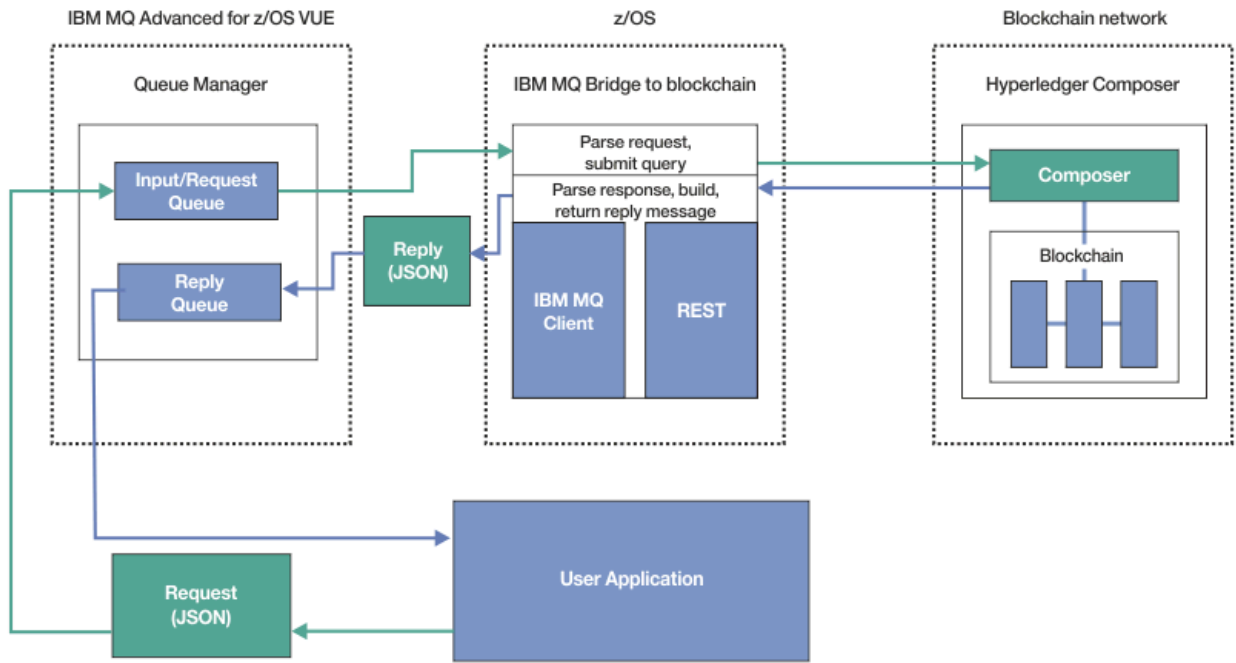
그림 128. IBM MQ Bridge to blockchain
