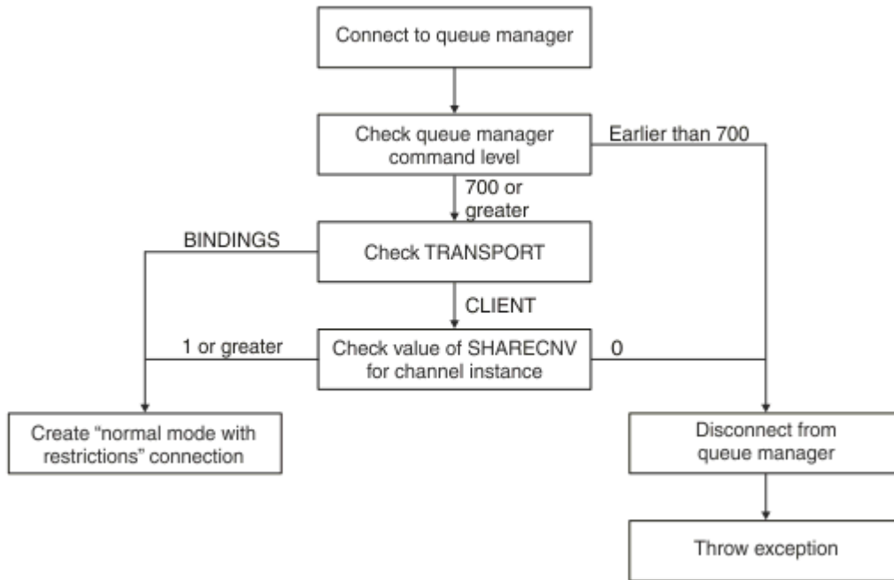
그림 94. 제한이 있는 PROVIDERVERSION 정상 모드
