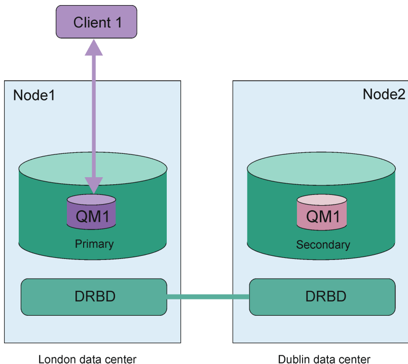
그림 84. 단일 RDQM 쌍
