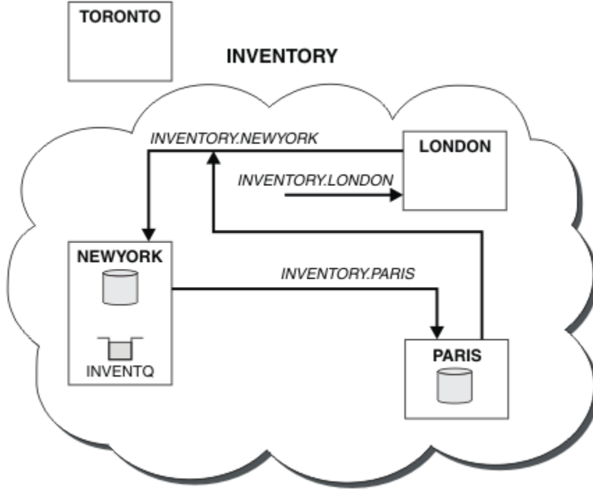
그림 46. 전체 저장소가 PARIS로 이동된 INVENTORY 클러스터
