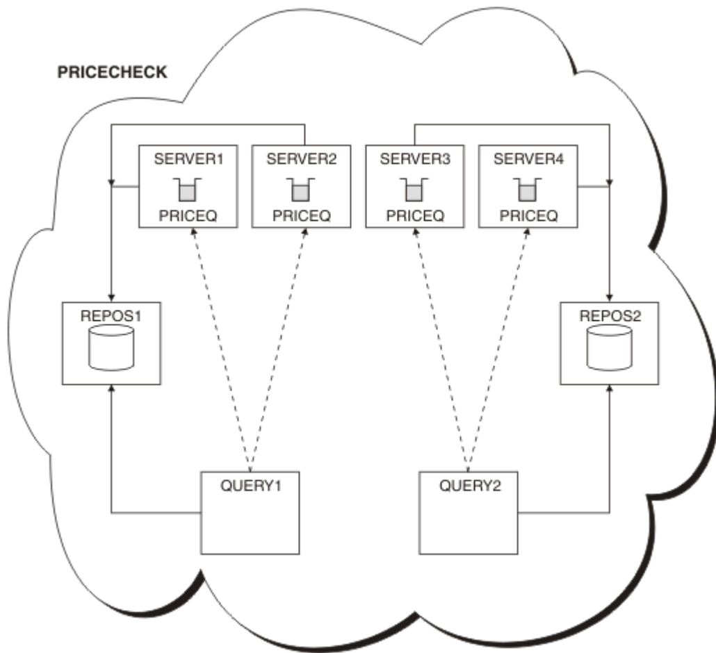
그림 65. 네 개의 서버 큐 관리자, 두 개의 저장소 및 두 개의 조회 큐 관리자가 포함된 PRICHECK 클러스터
