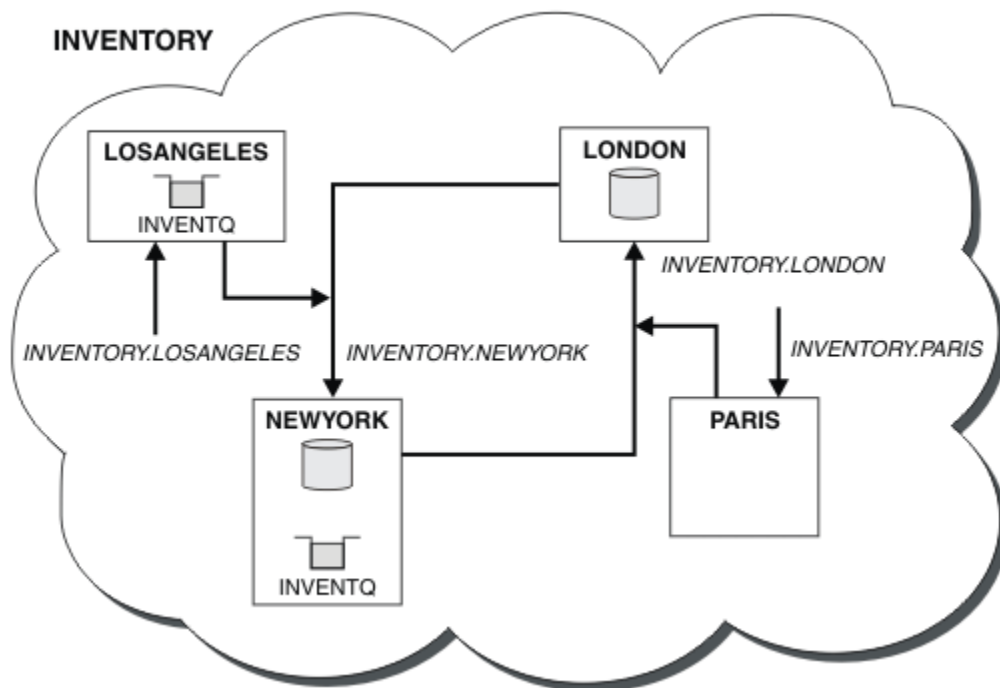
그림 66. 네 개의 큐 관리자가 있는 INVENTORY 클러스터
