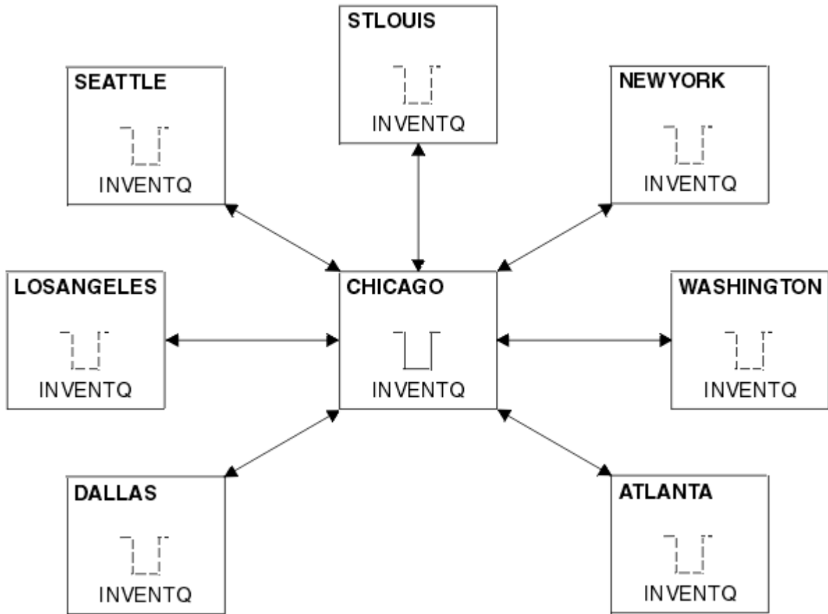
그림 47. 허브 및 스포크 네트워크
