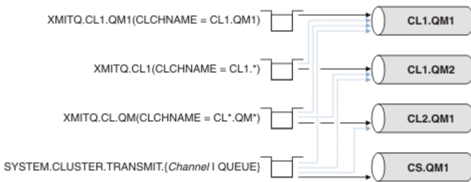
그림 39. 전송 큐 / 클러스터 송신자 채널 우선순위
