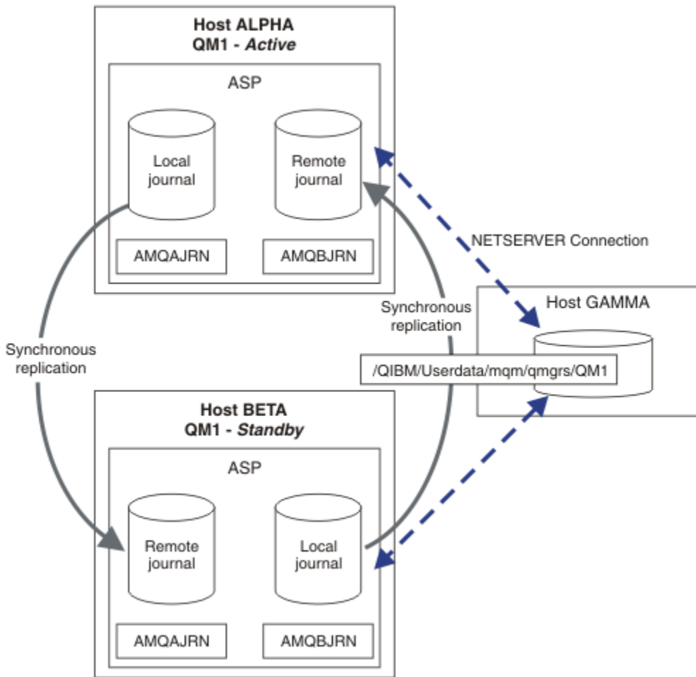
그림 29. 미러링된 저널 구성
