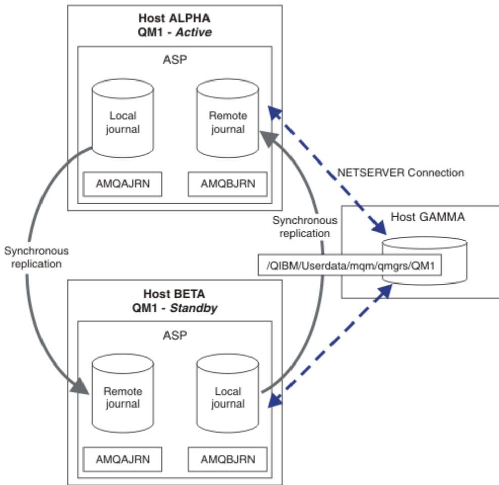
그림 27. 큐 관리자 저널 미러링
