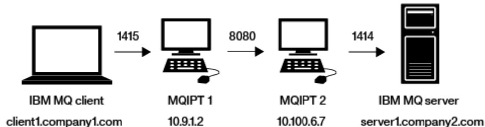
図 33. HTTP トンネリングネットワーク図
