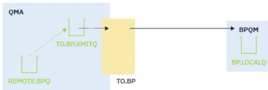
図 15. アウトバウンド構成
