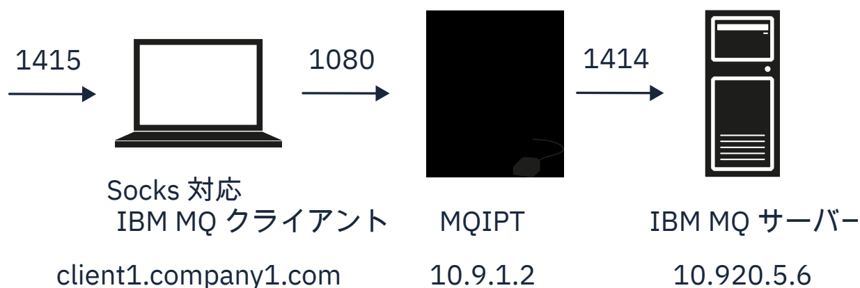
図 35. SOCKS プロキシのネットワーク図
