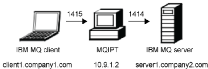
図 42. セキュリティー出口のネットワーク図
