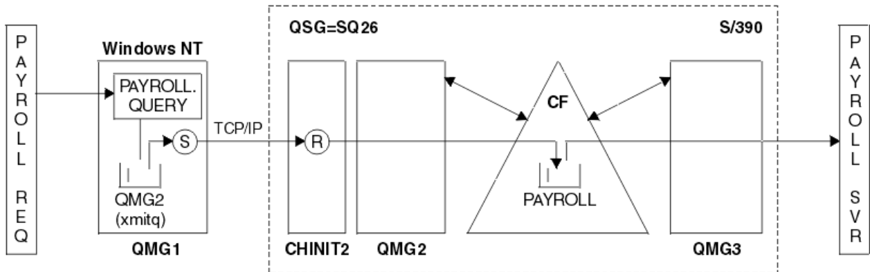
図 4. 構成 3
