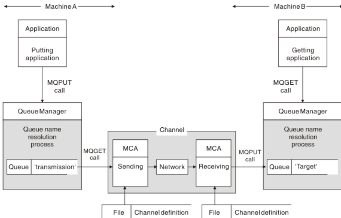
図 5. 名前の解決
