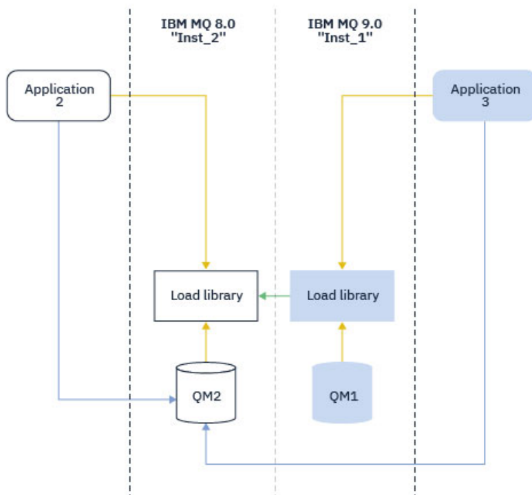
図 11. 別のライブラリーでのロードの呼び出し
