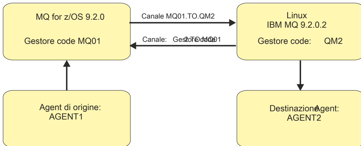
Figura 55. Esempio di un semplice diagramma che mostra come un agent di origine, AGENT1, e un agent di destinazione, AGENT2, e i relativi gestori code agent, MQ01 e QM2 sono connessi.
