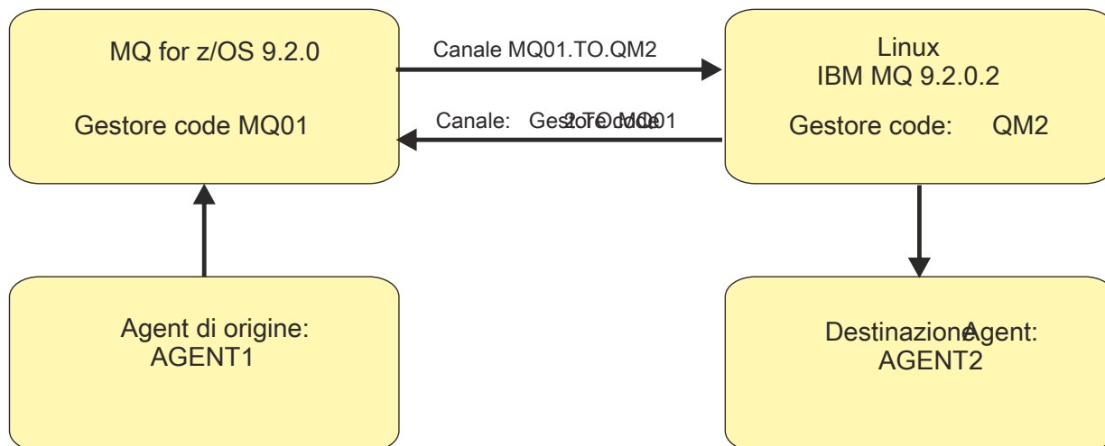
Figura 56. Esempio di un semplice diagramma che mostra come un agent di origine, AGENT1, e un agent di destinazione, AGENT2, e i relativi gestori code agent, MQ01 e QM2 sono connessi.
