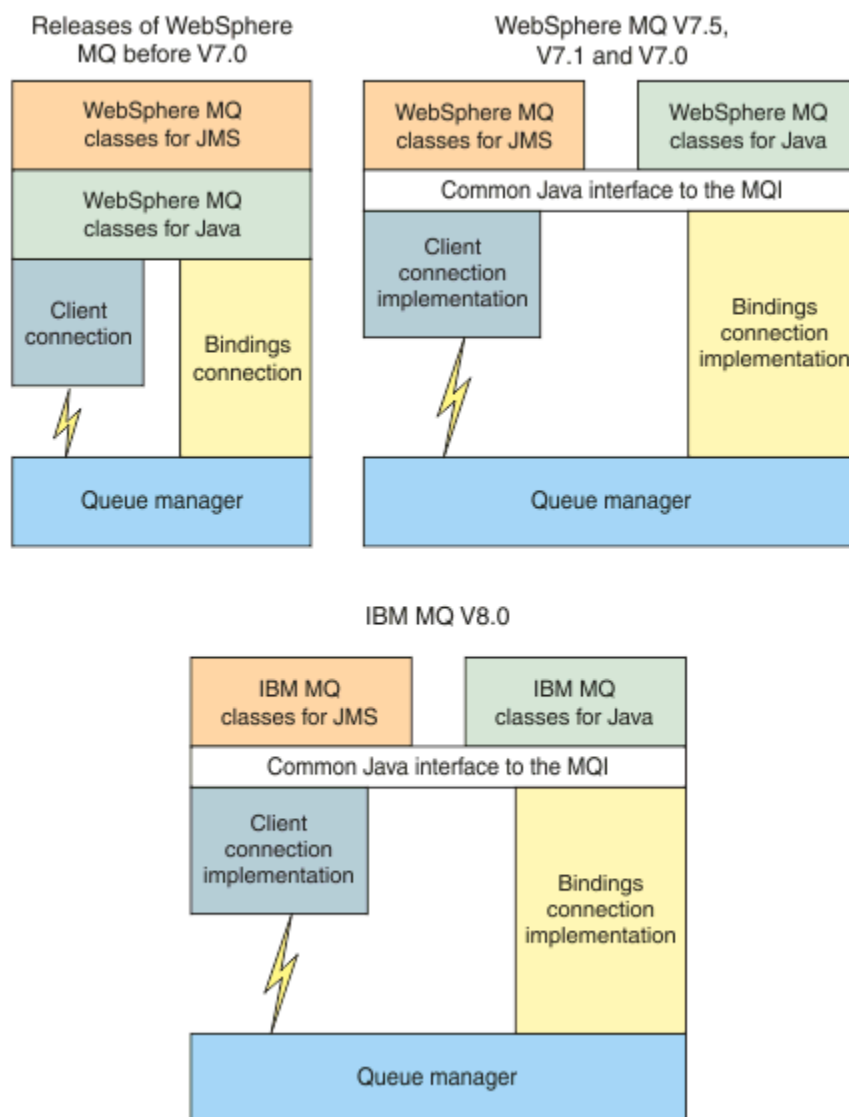
Figura 56. La relazione tra IBM MQ classes for JMS e IBM MQ classes for Java
