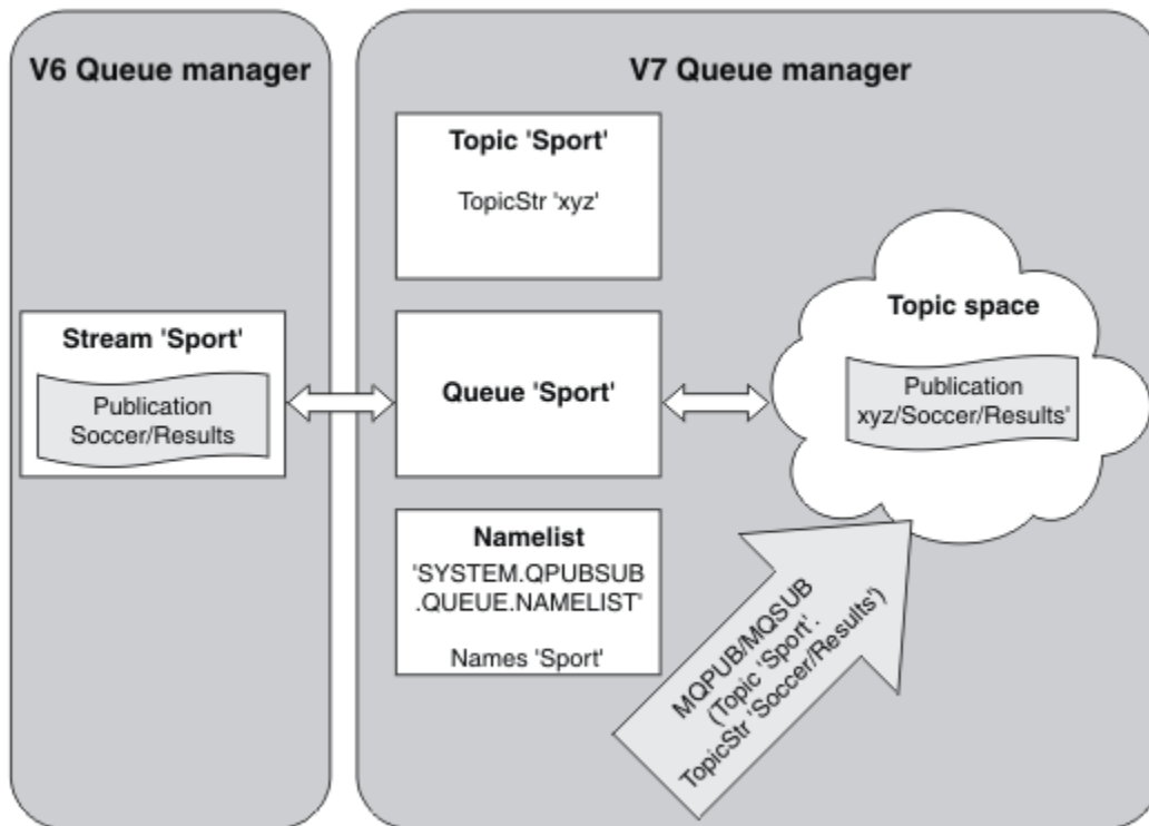
Figura 31. Stream di IBM WebSphere MQ 6 che coesistono con argomenti IBM WebSphere MQ 7
