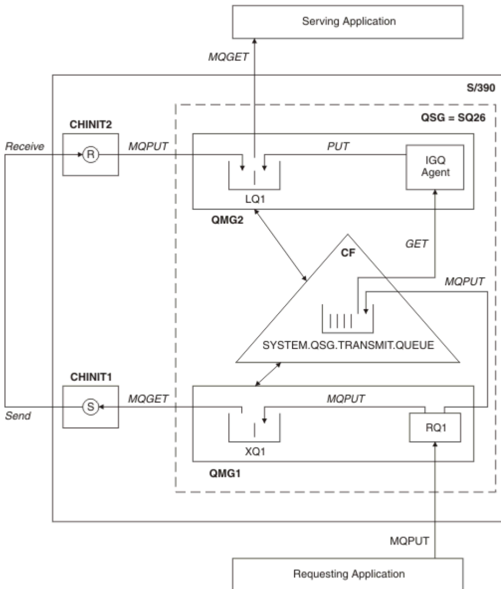
Figura 70. Una configurazione di esempio
