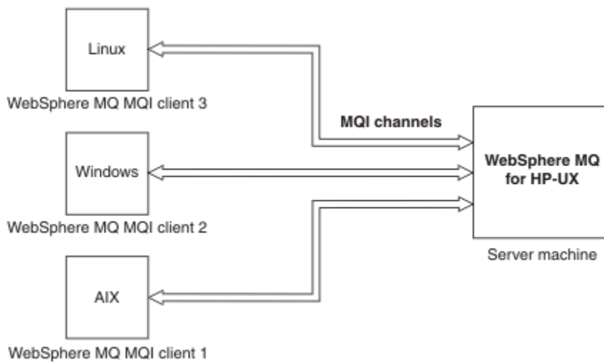
Figura 53. Server IBM MQ connesso a client su piattaforme differenti
