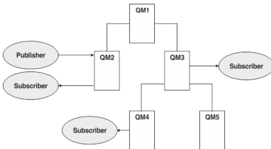
Figura 35. Gerarchia di pubblicazione / sottoscrizione
