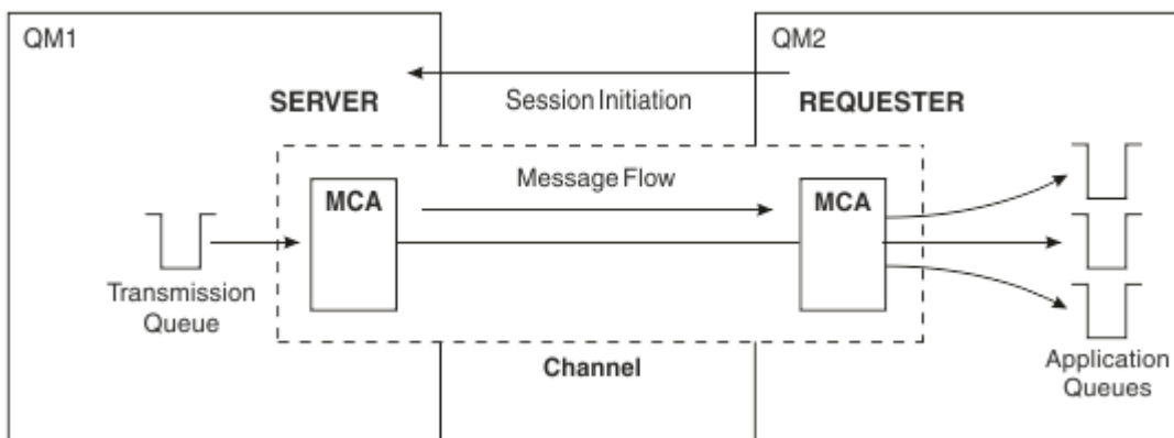
Figura 9. Un canale richiedente - server
