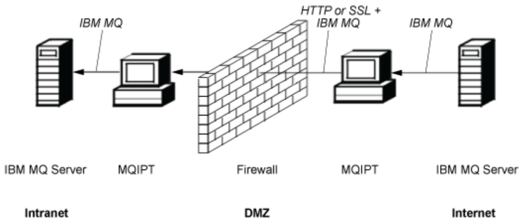
Figura 82. Esempio di tunneling MQIPT e HTTP
