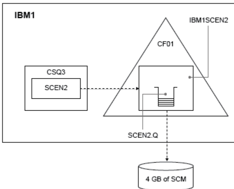
Figura 65. Configurazione dell'aggiunta di SCM per prestazioni migliori
