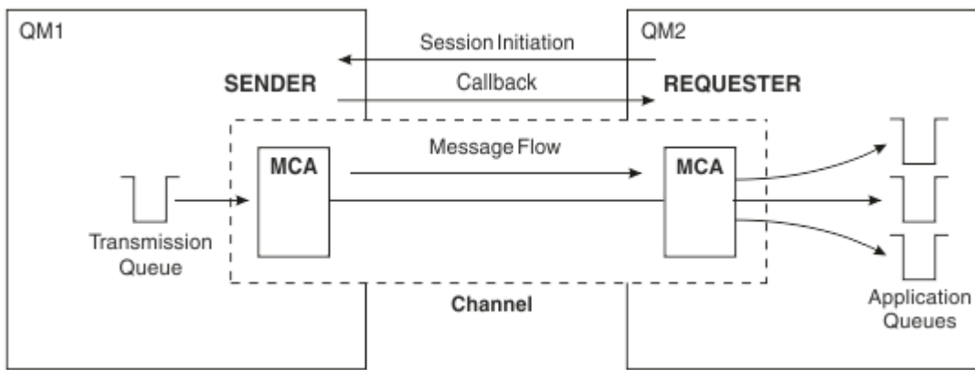
Figura 10. Un canale richiedente - mittente
