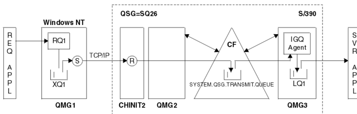
Figura 69. Un esempio di supporto di migrazione
