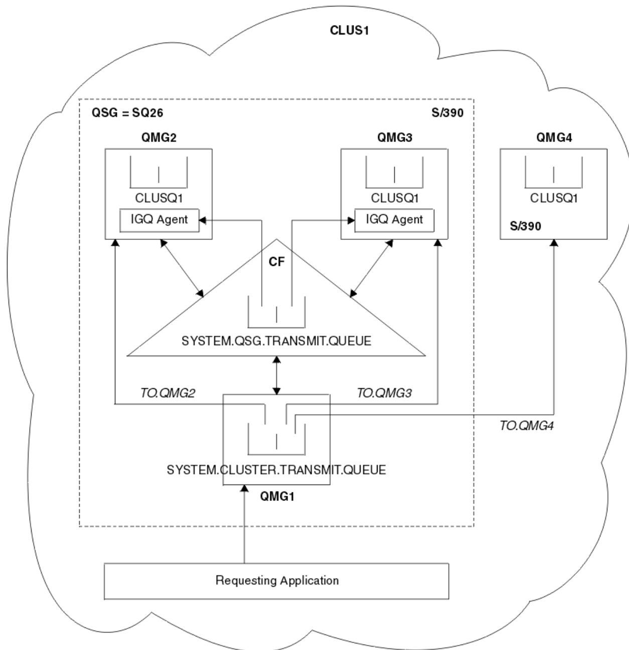
Figura 71. Un esempio di cluster con accodamento all'interno del gruppo
