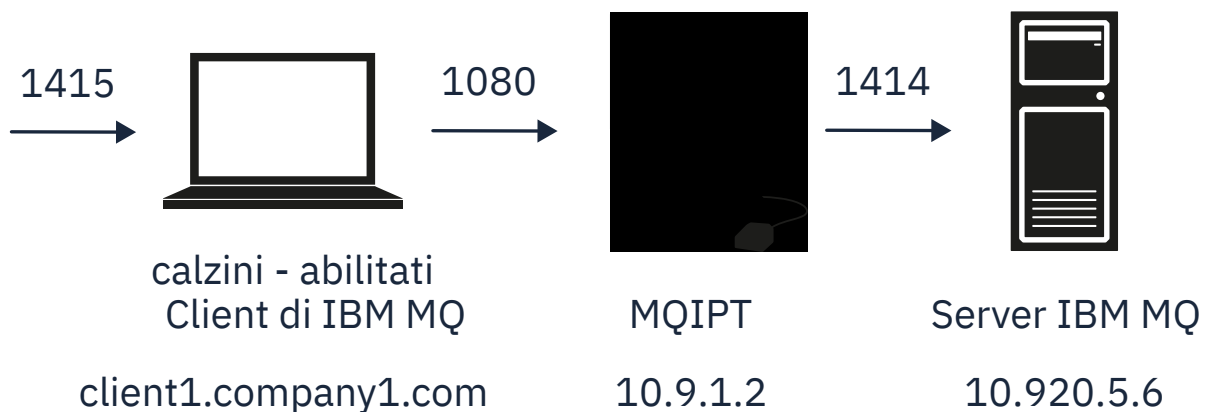
Figura 35. Diagramma di rete proxy SOCKS
