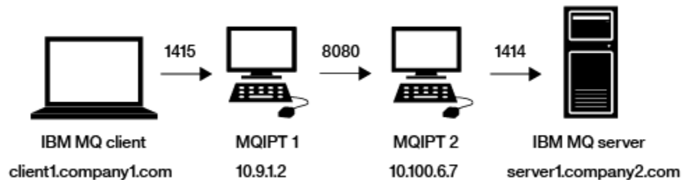
Figura 33. Diagramma di rete di tunneling HTTP
